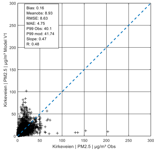
Figure A 146: Hourly values PM 2.5 in Kirkeveien, V1
