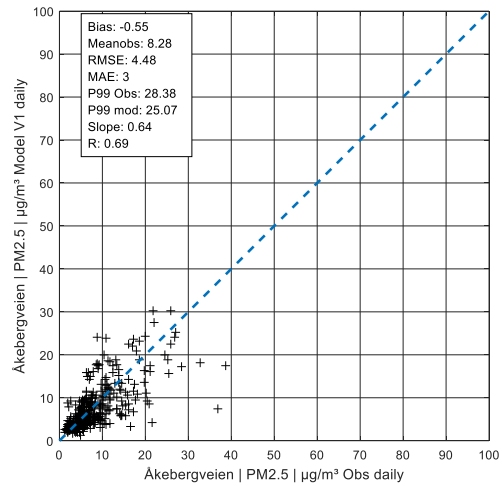
Figure A 135: Daily values PM 2.5 in Åkebergveien, V1
