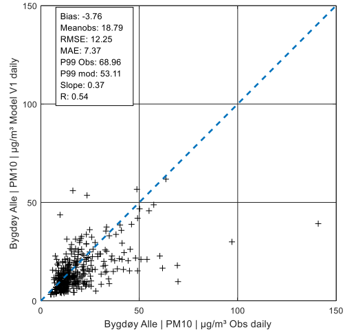
Figure A 114: Daily values PM 10 in Bygdøy Allè, V1
