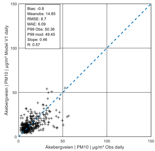
Figure A 108: Daily values PM 10 in Åkebergveien, V1
