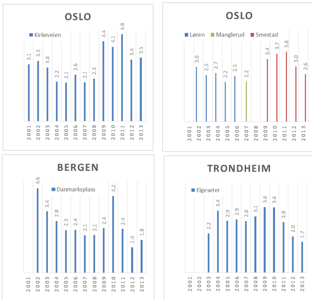
Figur 10: Årsmiddelverdi av benzen i Oslo, Bergen og Trondheim. Årsgrenseverdi er 5 \mu\text{g m}^{-3} , den øvre vurderingsterskelen er 3,5 \mu\text{g m}^{-3} ) og den nedre vurderingsterskelen er 2 \mu\text{g m}^{-3} .
