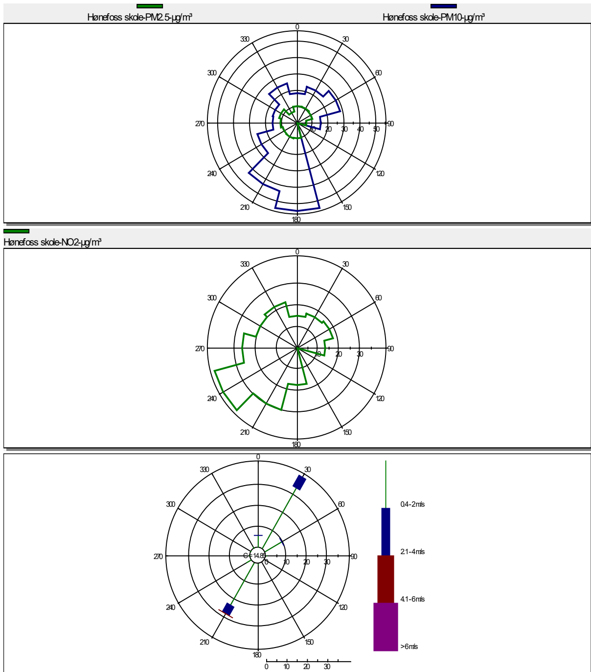
Belastning av \text{PM}_{10} , \text{PM}_{2.5} og \text{NO}_2 fordelt på vindretning i sektorer for mars-april-mai 2019.
