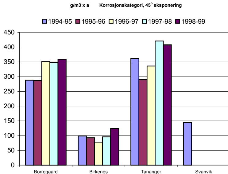
Figur 2: Ett-års korrosjon for stål på NILUs feltstasjoner, 1996, 1997 og 1998. ISOs klasser for korrosjon er vist på figuren.
