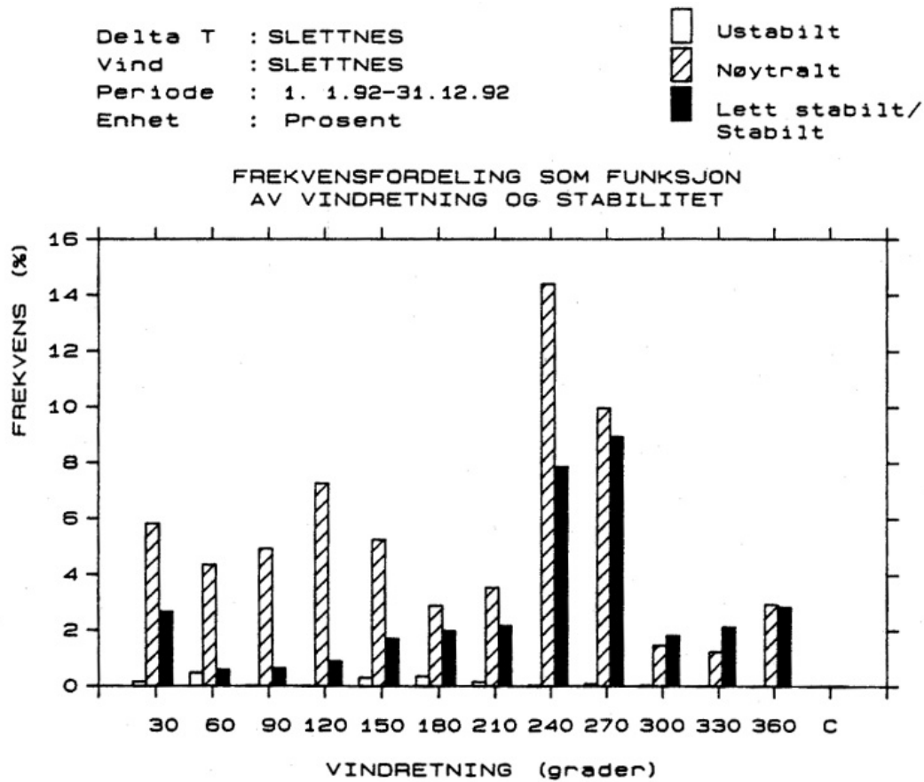
Figur B: Forekomst av ustabil, nøytral og stabil sjiktning for hele måleperioden fordelt på 12 vindsektorer.
