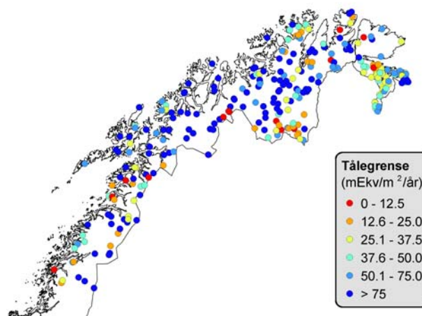
Figur 6: Tålegrenser for forsuring av overflatevann.
