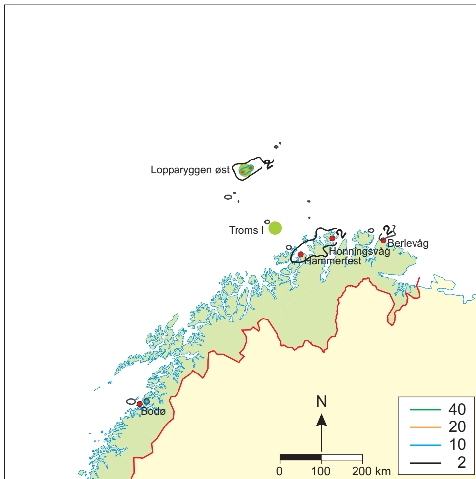
Figur 23: Avsetning av nitrogen fra utslipp av nitrogenoksider for middels aktivitetsnivå, med bidrag fra faste installasjoner. Enhet: mg N/m 2 for ett år.
