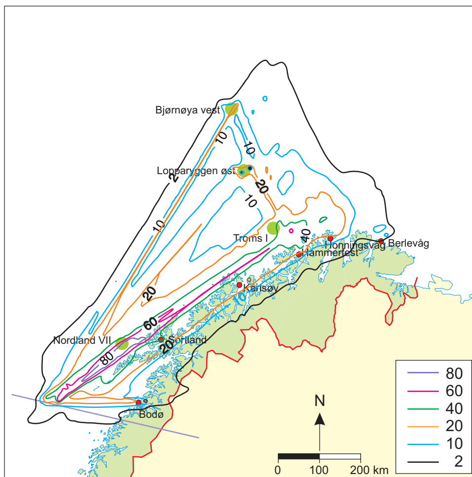
Figur 28: Avsetning av nitrogen fra utslipp av nitrogenoksider for høyt aktivitetsnivå, med bidrag fra alle kilder. Enhet: mg N/m 2 for ett år.
