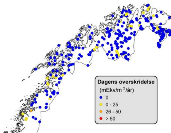
Figur 7: Overskridelse av tålegrensen for forsuring av vann, beregnet med SSWC modellen og dagens avrenning av nitrogen, gitt avsetning av nitrogen og svovel som gjennomsnitt for 1997-2001.
