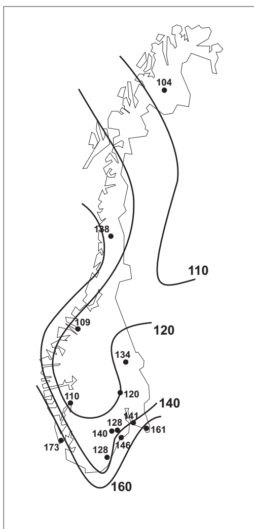
Figur 9: Antall døgn med 8-timers middelveier av ozon over 60 \mu\text{g}/\text{m}^3 , april–september 2001 (Aas et al., 2002).
