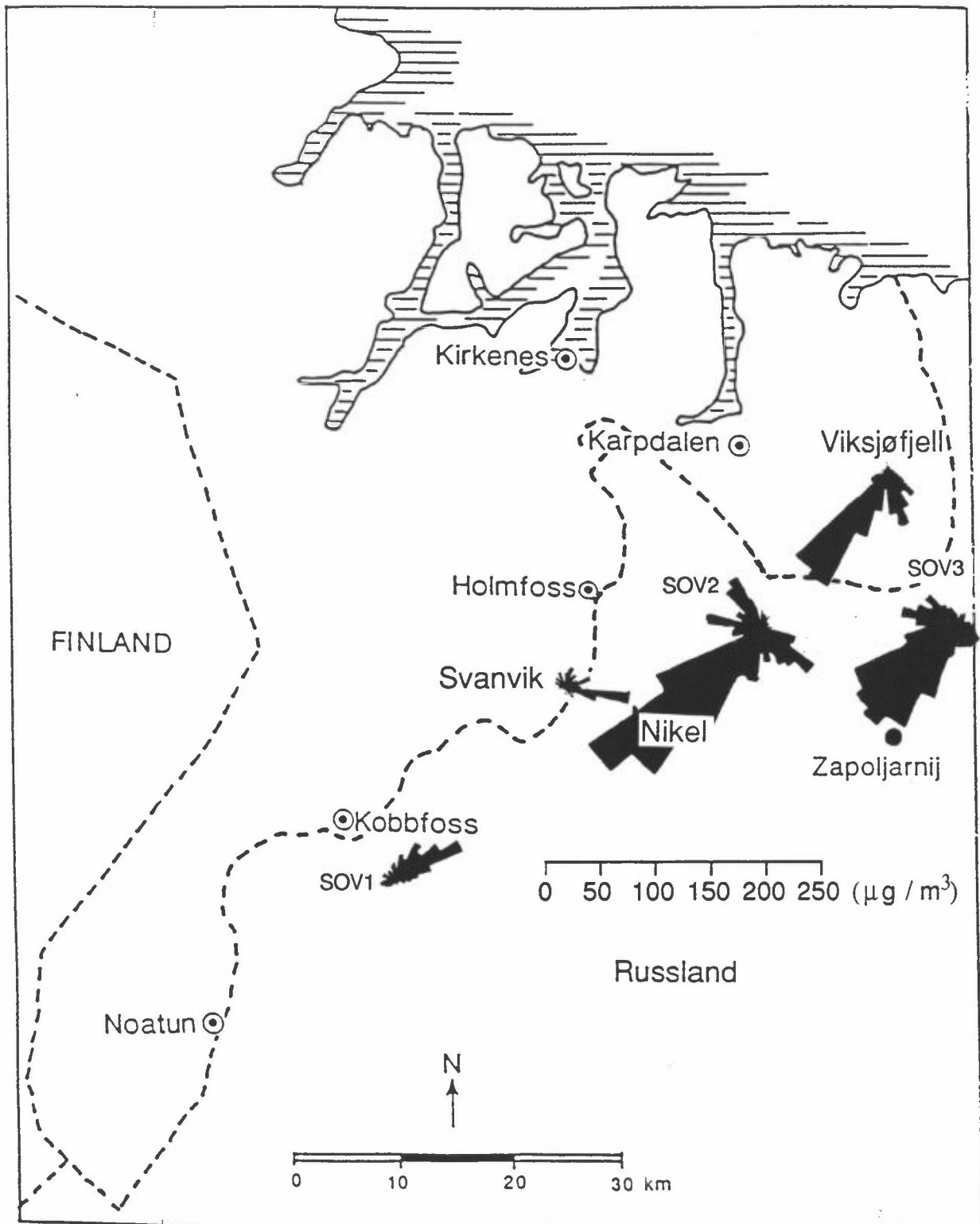
Figur 25: Middelkonsentrasjoner av \text{SO}_2 for Viksjøfjell, Svanvik, SOV 1, SOV 2 og SOV 3 i 36 vindsektorer i perioden oktober 1991-mars 1992 ( \mu\text{g}/\text{m}^3 ).
