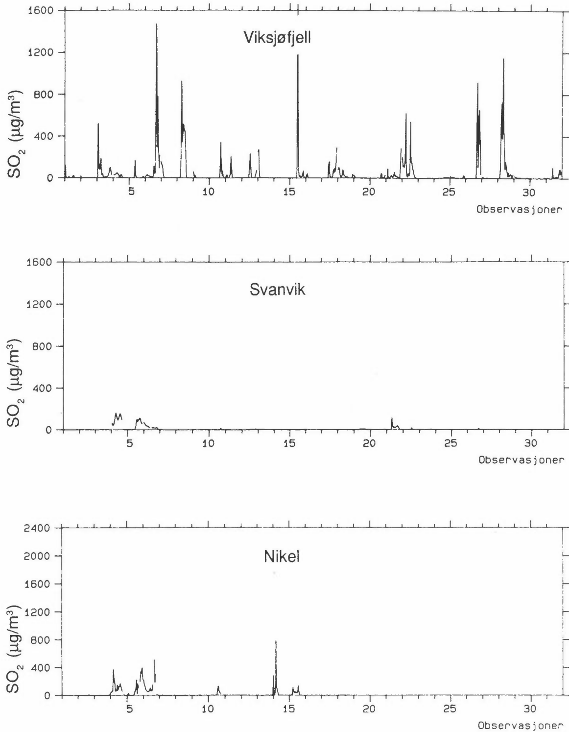
Figur 17: Timemiddelkonsentrasjoner av SO 2 i desember 1991 på Viksjøfjell, i Svanvik og i Nikel (µg/m 3 ).
