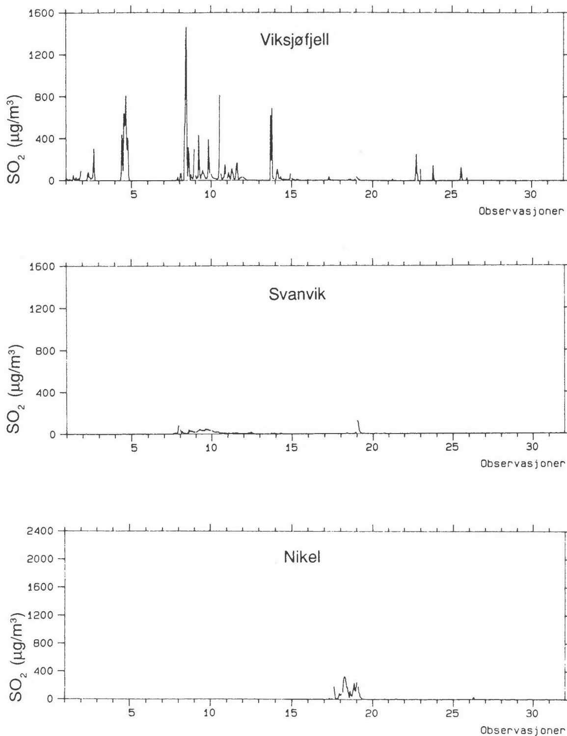
Figur 19: Timemiddelkonsentrasjoner av \text{SO}_2 i januar 1992 på Viksjøfjell, i Svanvik og i Nikel ( \mu\text{g}/\text{m}^3 ).
