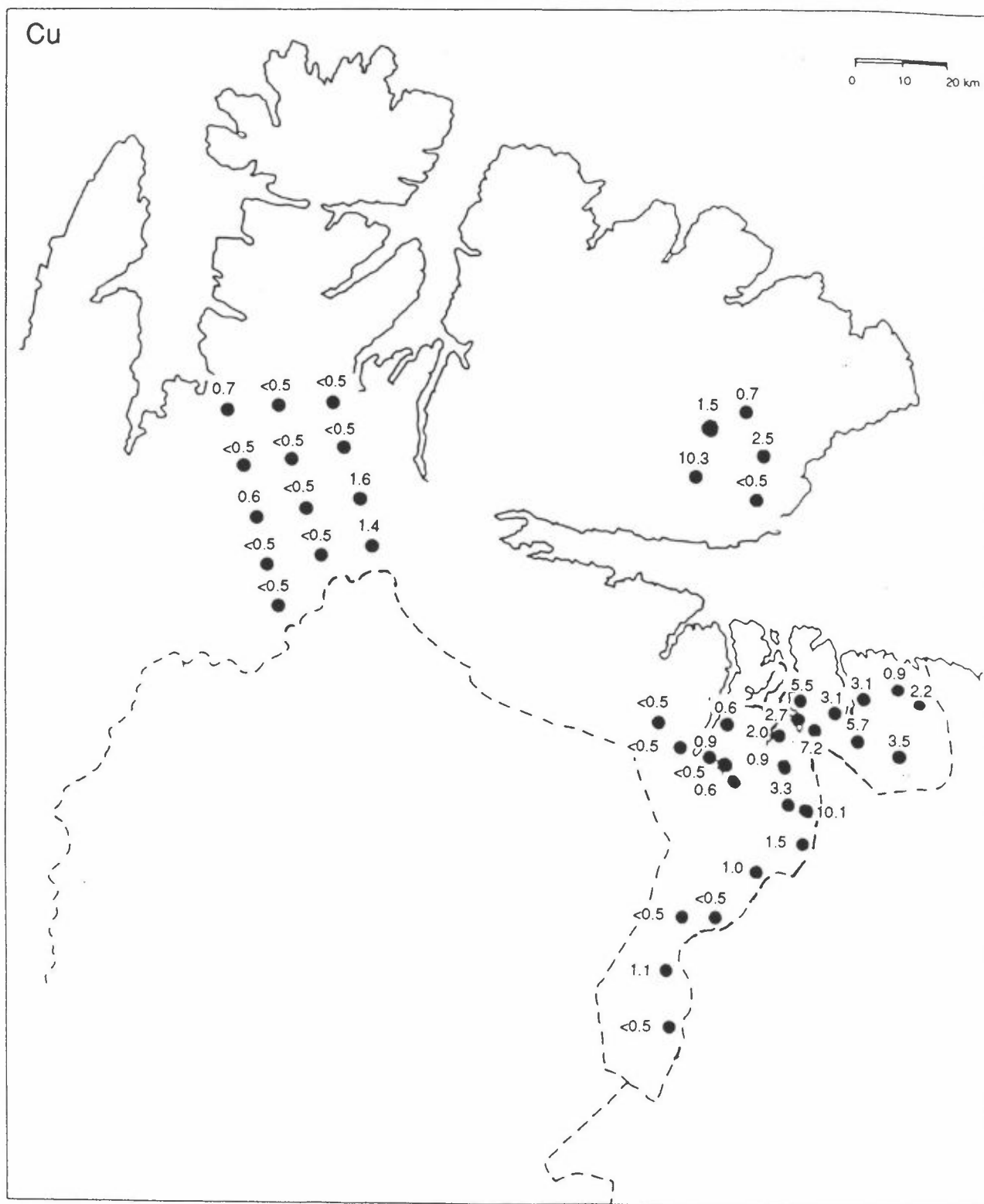
Figur 33: Konsentrasjoner av kopper (Cu) i snøprøver fra Øst-Finnmark, mars/april 1992 ( \mu\text{g/l} ).
