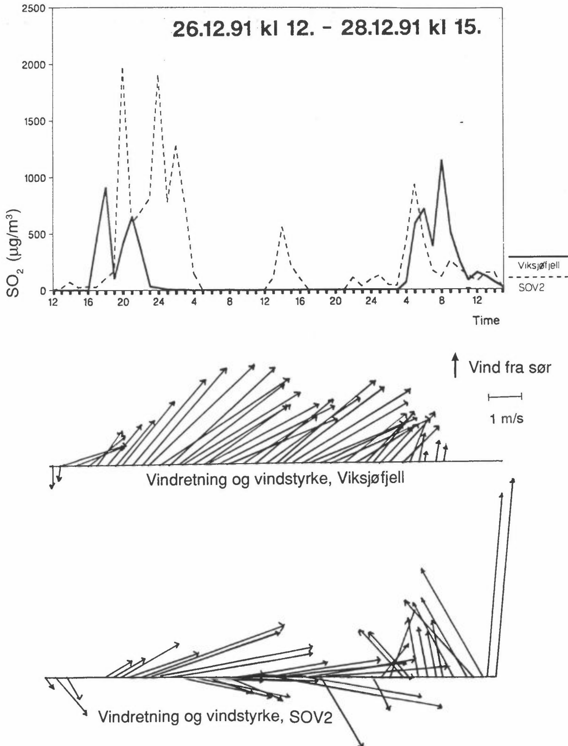
Figur 8: Timemiddelverdier av SO 2 , vindretning og vindstyrke på Viksjøfjell og SOV 2 26.-28.12.1991.
