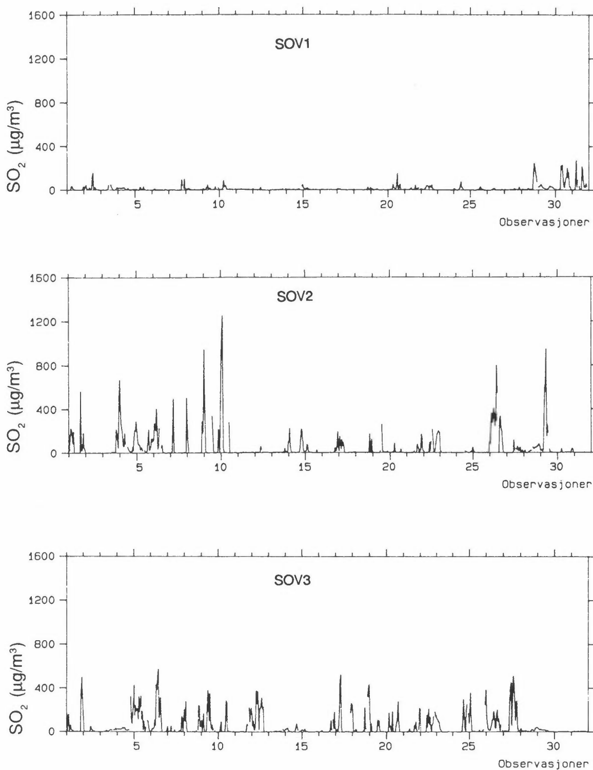
Figur 24: Timemiddelkonsentrasjoner av SO 2 i mars 1992 på SOV 1, SOV 2 og SOV 3 (µg/m 3 ).
