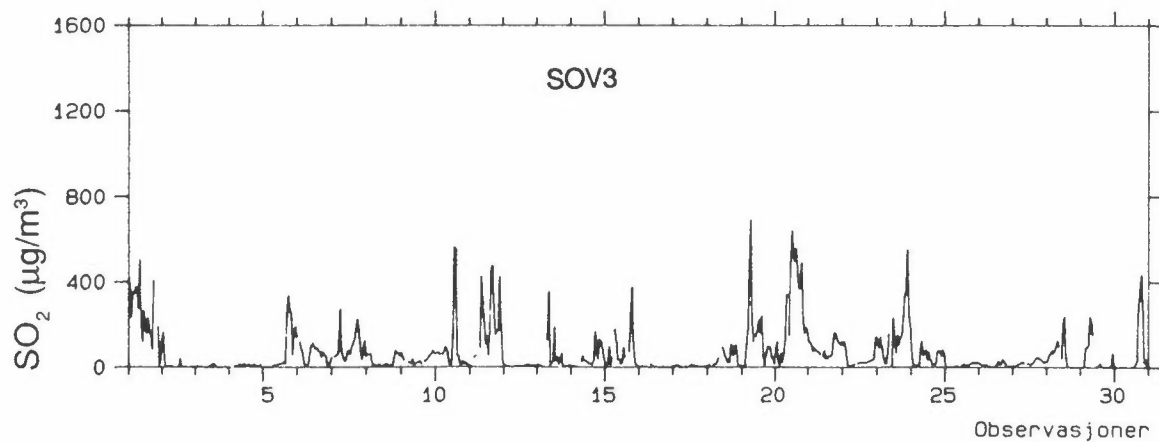
Figur 16: Timemiddelkonsentrasjoner av SO 2 i november 1991 på SOV 1, SOV 2 og SOV 3 (µg/m 3 ).
