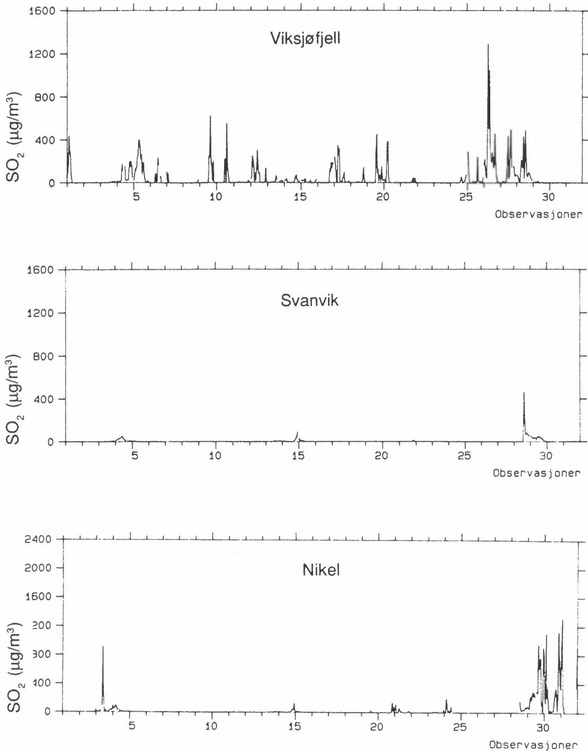
Figur 23: Timemiddelkonsentrasjoner av \text{SO}_2 i mars 1992 på Viksjøfjell, i Svanvik og i Nikel ( \mu\text{g}/\text{m}^3 ).
