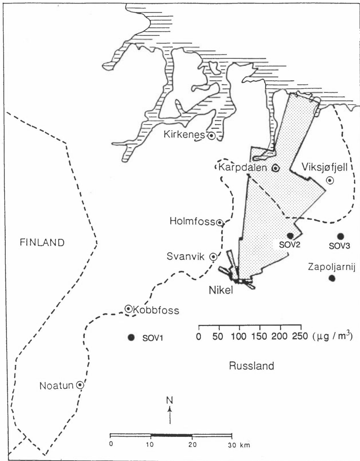
Figur 26: Middelkonsentrasjoner av SO 2 for Nickel (samme skala som i figur 25) i 36 vindsektorer i perioden oktober 1991-mars 1992 ( \mu\text{g}/\text{m}^3 ).
