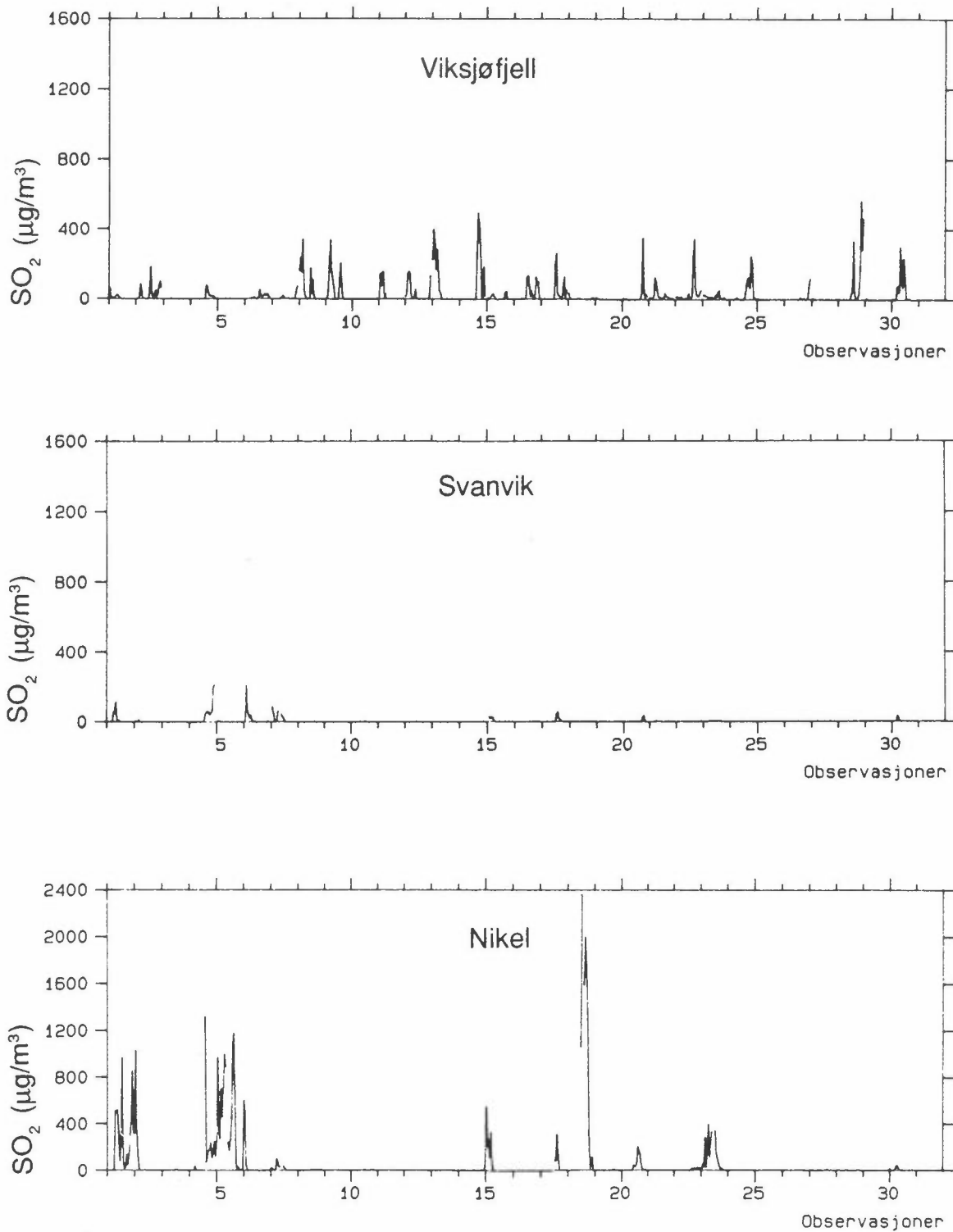
Figur 13: Timemiddelkonsentrasjoner av SO 2 i oktober 1991 på Viksjøfjell, i Svanvik og i Nikel (µg/m 3 ).
