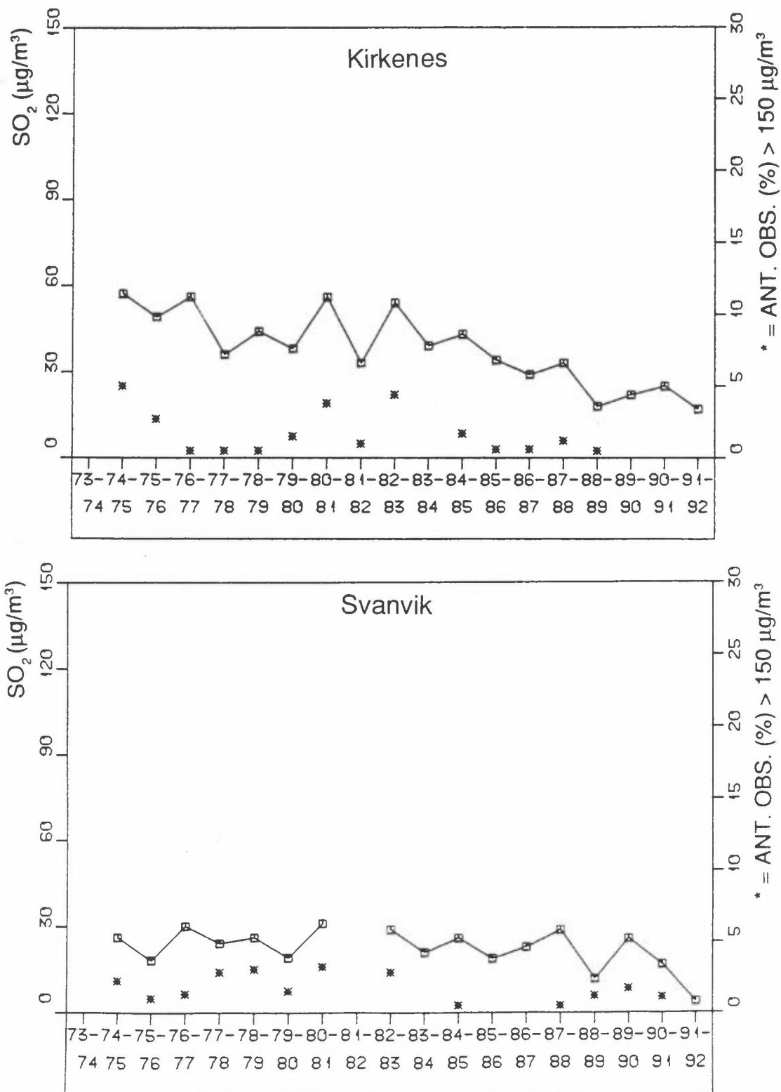
Figur 11: Vintermiddelkonsentrasjoner av SO 2 (µg/m 3 ) og frekvens av døgnmiddelverdier over 150 µg/m 3 på Rådhuset i Kirkenes og i Svanvik.
