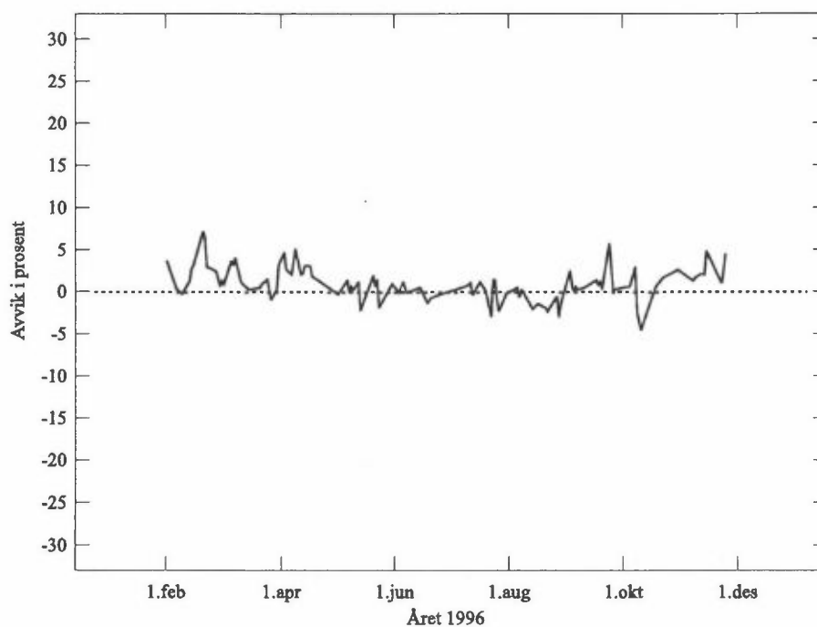
Figur 17: Sammenligning mellom ozonmålinger utført med Dobson og GU-511 for Oslo in 1996, 100 \cdot (\text{Dobson-GU}) / \text{Dobson} .
