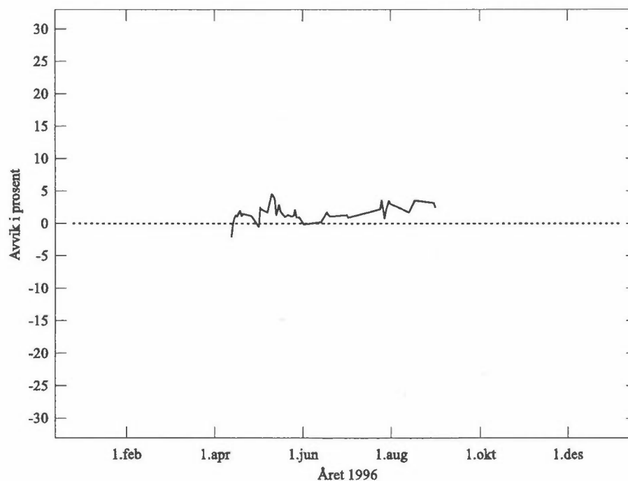
Figur 20: Sammenligning mellom ozonmålinger utført med GUV-541 og Dobson-instrumentet i Tromsø i 1996, 100 \cdot (\text{Dobson} - \text{GUV}) / \text{Dobson} .
