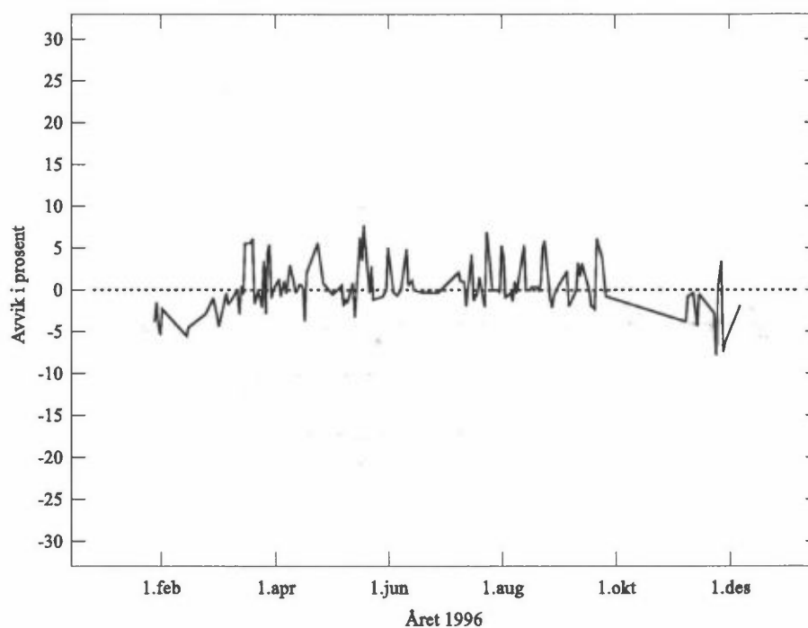
Figur 16: Sammenligning mellom ozonmålinger utført med Dobson- og Brewer-instrumentene for Oslo i 1996, 100 \cdot (\text{Dobson-Brewer}) / \text{Dobson} .
