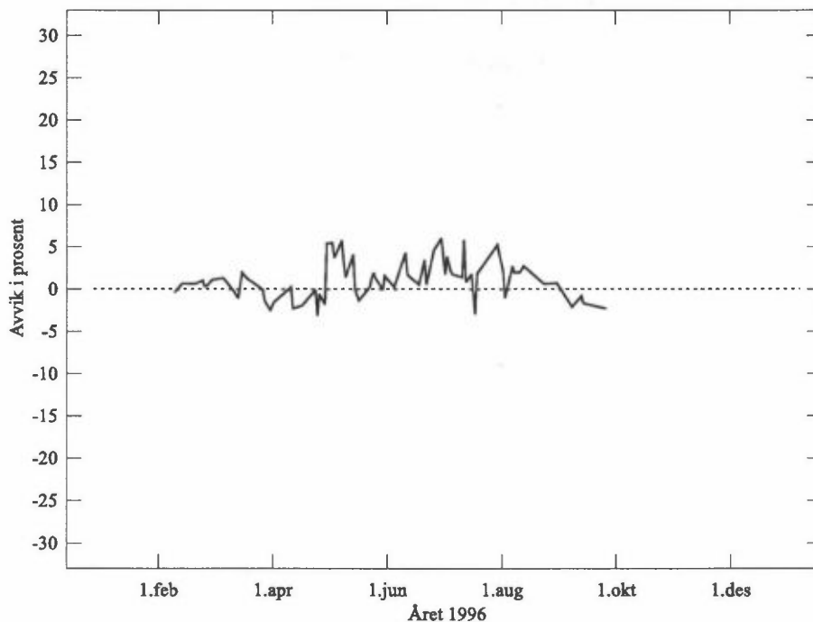
Figur 18: Sammenligning mellom ozonmålinger utført med Dobson- og Brewer-instrumentet for Tromsø i 1996, 100 \cdot (\text{Dobson} - \text{Brewer}) / \text{Dobson} .
