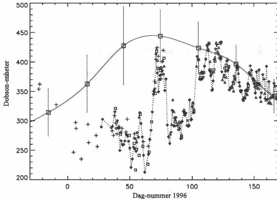
Figur 12: Målinger av totalozon fra Andøya (lidar) og Tromsø (Dobson, GUV og Brewer). Lidar målingene er markert med +. Langtidsmålinger med Dobson-instrumentet i Tromsø i perioden 1950-1972 er foreløpige data.
