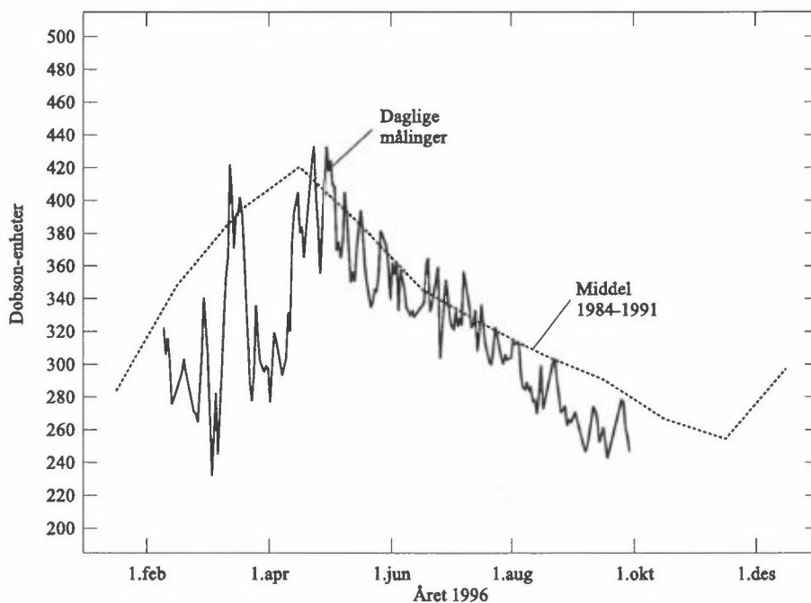
Figur 2: Daglige ozonverdier målt med Dobson- og Brewer-instrumentene ved Universitetet i Tromsø i 1996. Den stiplete kurven er månedsmidlene fra 1984 til 1991.
