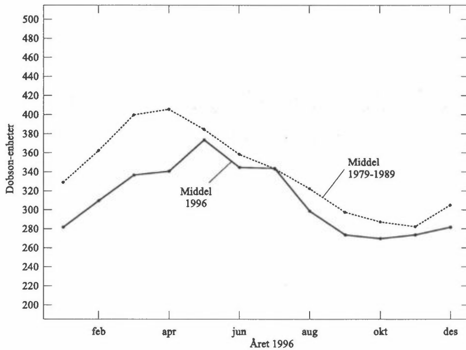
Figur 4: Månedsmiddelverdiene for 1996 og månedsmiddelverdiene for 1979 til 1989 for Oslo.
