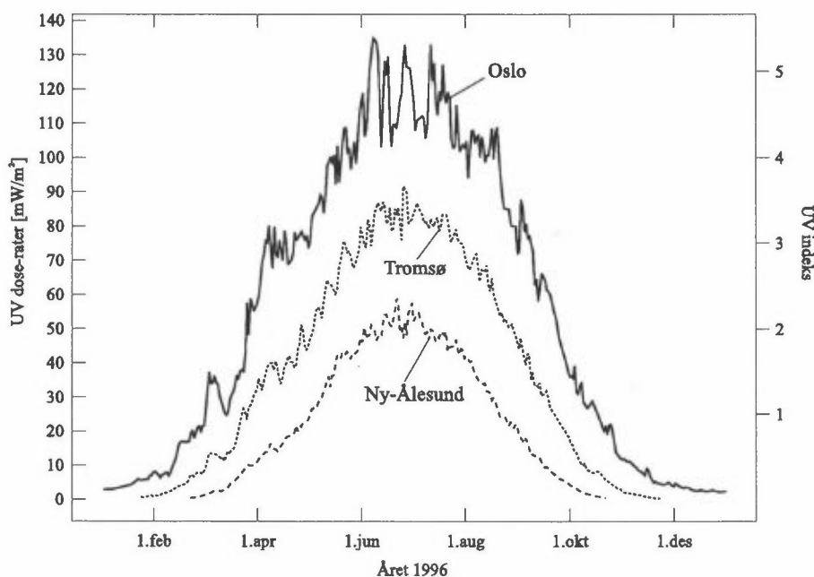
Figur 29: UV-dose-raten midt på dagen redusert til klarvær og null bakkerefleksjon for Oslo, Tromsø og Ny-Ålesund.
