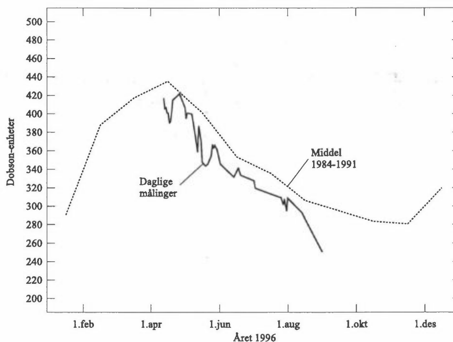
Figur 3: Daglige ozonverdier målt med Dobson-instrumentet i Ny-Ålesund 1996. Den stiplede kurven er månedsmidler fra 1984 til 1991.
