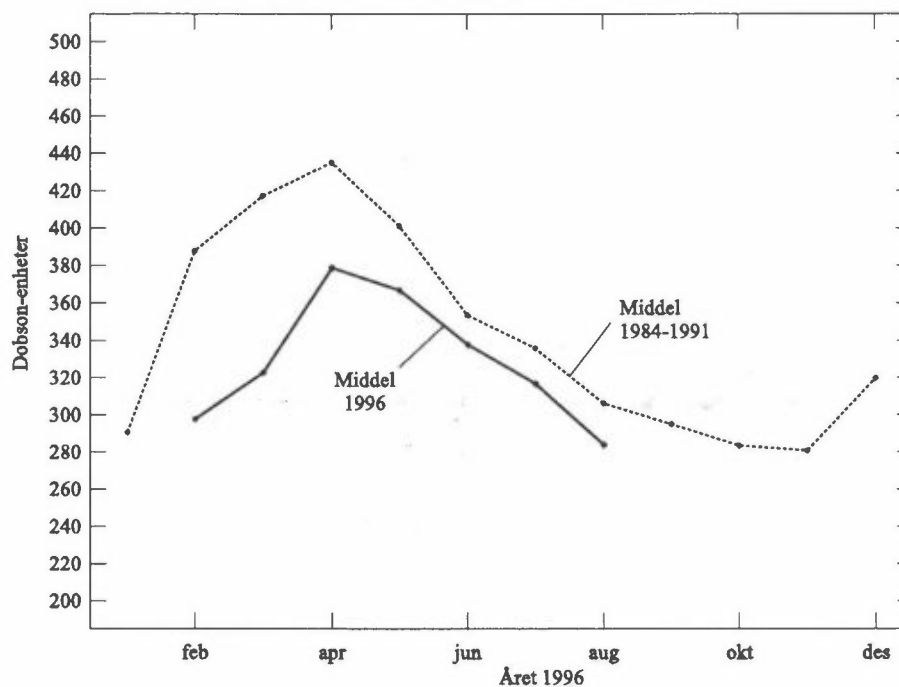
Figur 6: Månedsmiddelverdiene for 1996 og månedsmiddelverdiene for 1984 til 1991 for Ny-Ålesund.
