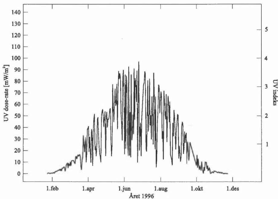
Figur 22: UV-doseraten midt på dagen fra 01.01.96 til 31.12.96 målt med GUV-541-instrumentet ved Universitetet i Tromsø.
