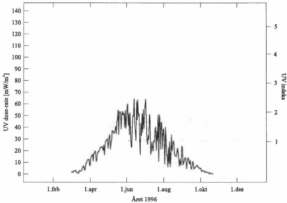
Figur 23: UV-doseraten midt på dagen fra 01.01.96 til 31.12.96 målt med GUV-541-instrumentet i Ny-Ålesund.
