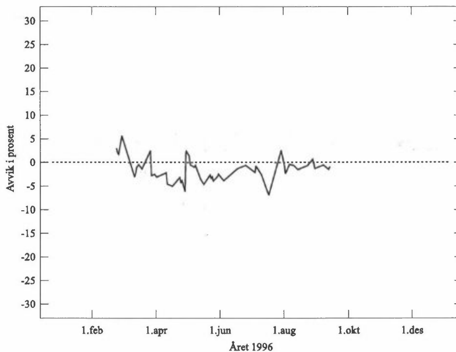
Figur 19: Sammenligning mellom ozonmålinger utført med GUV-541 og Dobson-instrumentet i Tromsø i 1996, 100 \cdot (\text{Dobson} - \text{GUV}) / \text{Dobson} .
