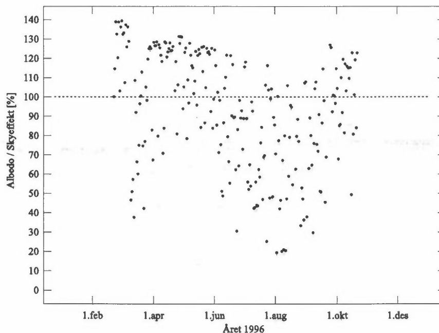
Figur 28: Effekter av skyer og bakkealbedo på UV-stråling ved jordens overflate i Ny-Ålesund i 1996 i prosent av klarværsverdien med null bakkerefleksjon. Hvert punkt representerer middelveien mellom 10:30 og 11:30 GMT for en bestemt dag. Den horisontale linjen representerer klarvær og barmark. Verdier over denne linjen betyr at skyer og/eller bakkealbedo øker UV-nivået sammenlignet med klarvær og bar bakke.
