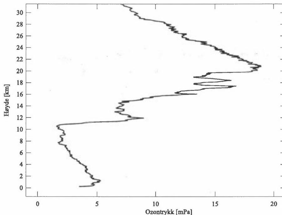
Figur 8: Høydefordelingen av ozon over Gardermoen 18. mars 1996 målt med ozonsonde sendt opp med ballong.
