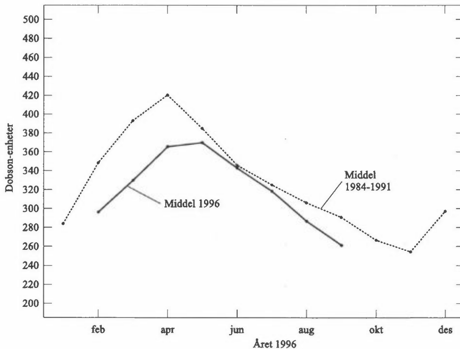
Figur 5: Månedsmiddelverdiene for 1996 og månedsmiddelverdiene for 1984 til 1991 for Tromsø.
