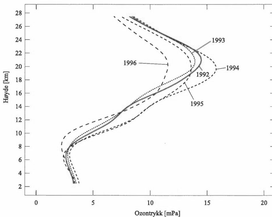
Figur 10: Midlere høydefordeling av ozon for januar-april for årene 1992 til 1996 over Gardermoen.
