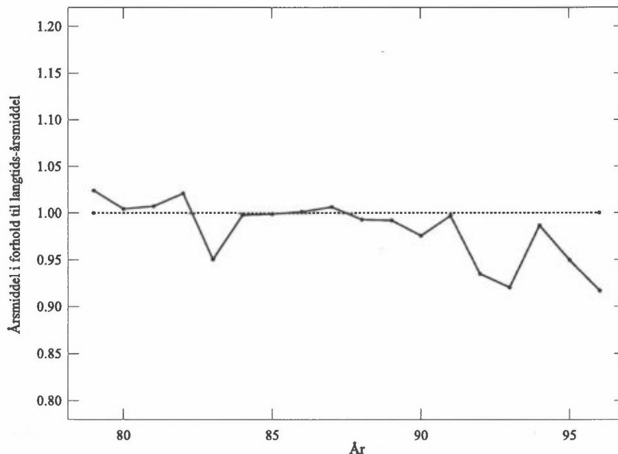
Figur15: Årsmidler i perioden 1979-1996 for Oslo basert på målinger med Dobson- og Brewer-instrumentet i Oslo. Figuren viser forholdet mellom hvert årsmiddel og langtids-årsmiddel for 1979-1989.
