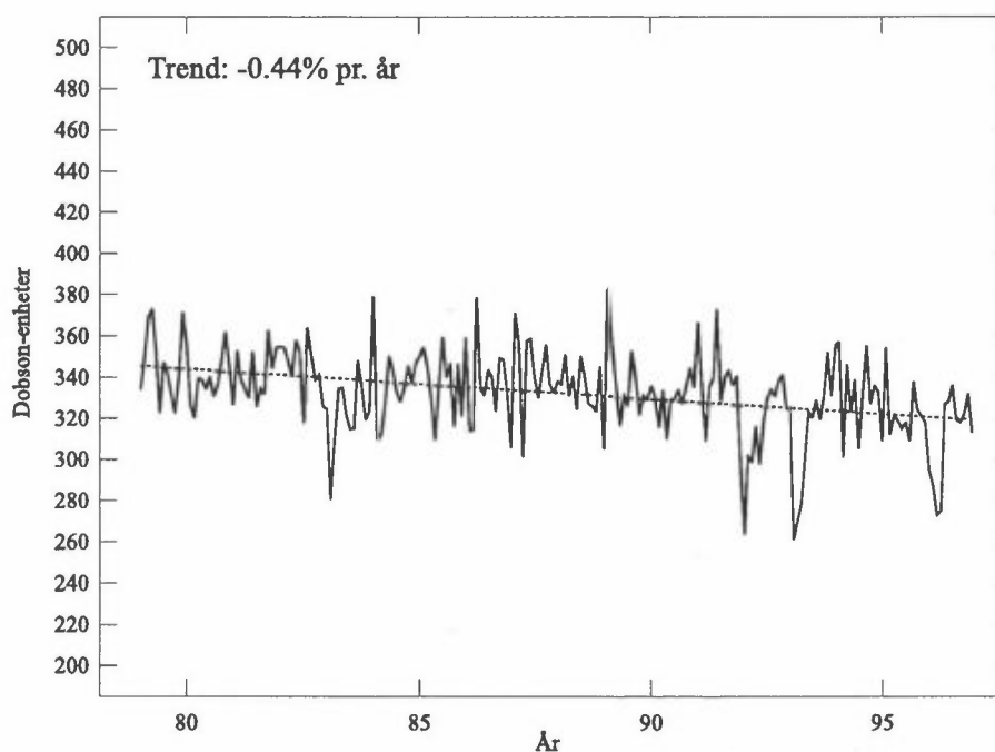
Figur14: Variasjon i ozonmengden over Oslo 1979-1996 basert på målinger med Brewer- og Dobson-instrumentene. Sesongvariasjonene er fjernet. På denne måten kommer trenden tydeligere frem enn i figur 13. Verdiene i figuren må ikke oppfattes som reelle månedsmidler (totalozon) siden sesongvariasjonene er fjernet.
