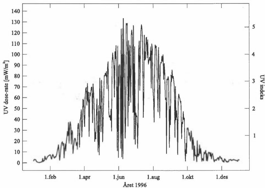
Figur 21: UV-doseraten midt på dagen fra 01.01.96 til 31.12.96 målt med GUV-511-instrumentet ved Universitetet i Oslo.
