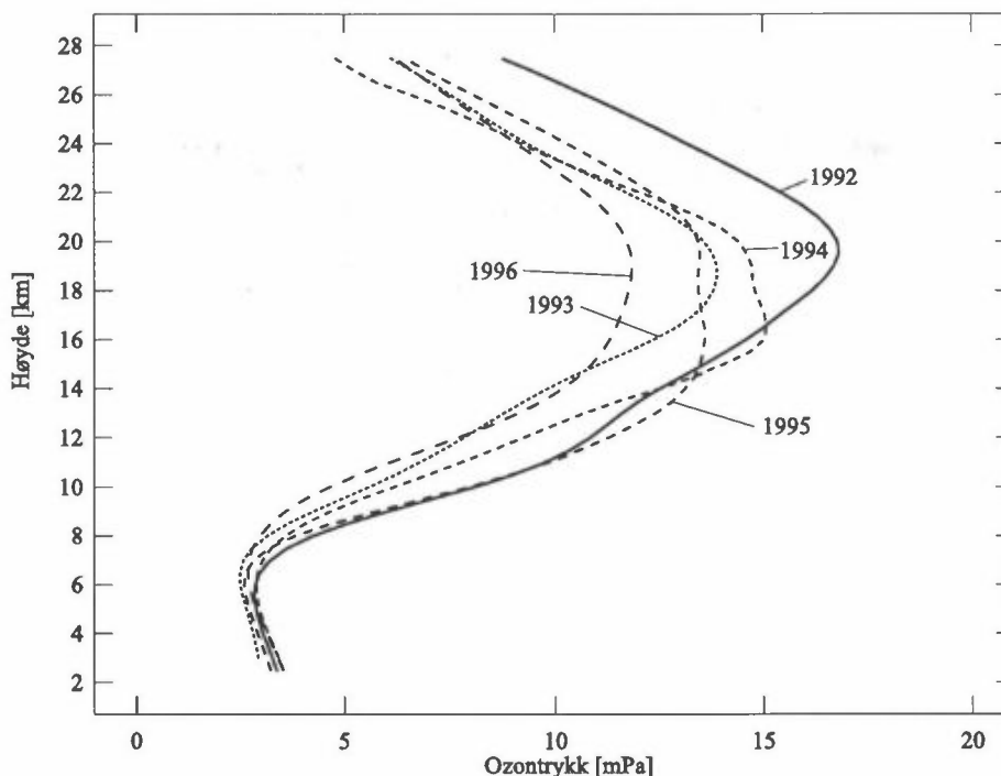
Figur 11: Midlere høydefordeling av ozon for januar-april for årene 1992 til 1996 over Bjørnøya.
