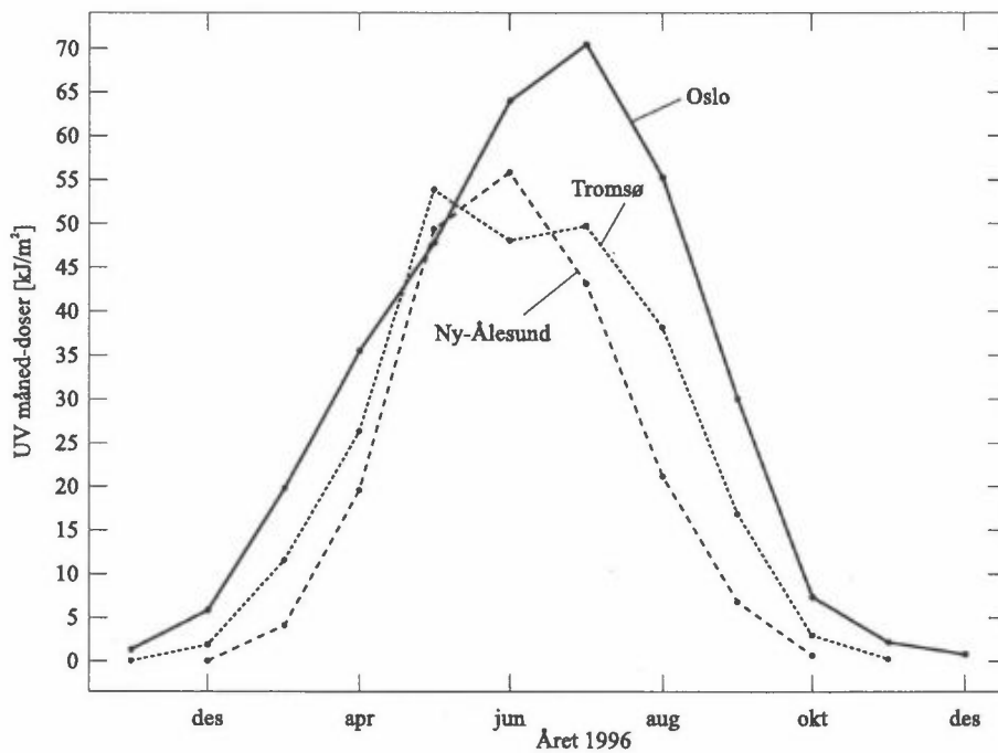
Figur 24: Månedlige integrerte UV-doser i 1996 målt med GUV-instrumentene i Oslo, Tromsø og Ny-Ålesund.
