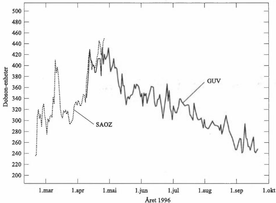
Figur 7: Daglige ozonverdier målt med GUV- og SAOZ-instrumentene i Ny-Ålesund i 1996.
