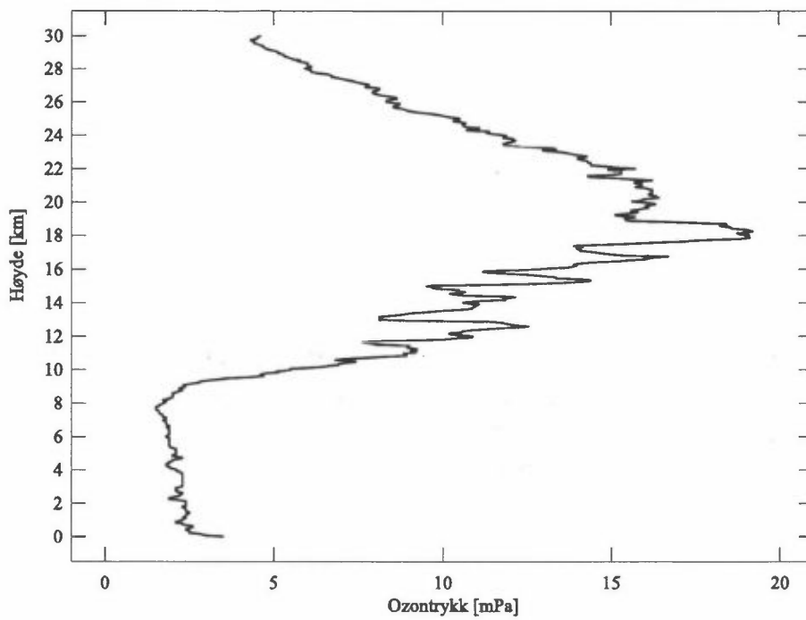
Figur 9: Høydefordeling av ozon målt over Bjørnøya 15. mars 1996 målt med ozonsonde sendt opp med ballong.
