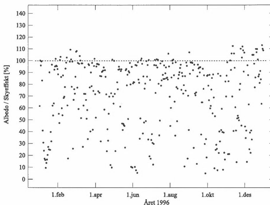
Figur 26: Effekter av skyer og bakkealbedo på UV-stråling ved jordens overflate i Oslo i 1996 i prosent av klarværsverdien med null bakkerefleksjon. Hvert punkt representerer middelverdien mellom 10:30 og 11:30 GMT for en bestemt dag. Den horisontale linjen representerer klarvær og barmark. Verdier over denne linjen betyr at skyer og/eller bakkealbedo øker UV-nivået sammenlignet med klarvær og bar bakke.
