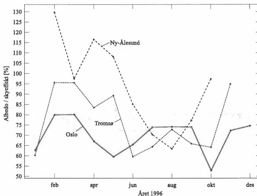
Figur 25: Albedo/skyeffekter for hver måned i 1996 målt med GUV-instrumentene i Oslo, Tromsø og Ny-Ålesund. Hvert punkt viser månedsverdien av UV-dosen i prosent av klarværsverdien med null bakkerefleksjon.
