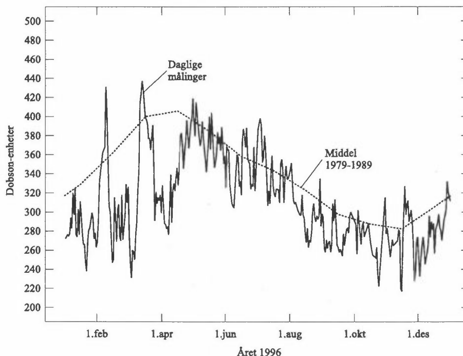
Figur 1: Daglige ozonverdier målt med Dobson- og Brewer-instrumentene ved Universitetet i Oslo i 1996. Den stiplede kurven er månedsmidler fra 1979 til 1989.
