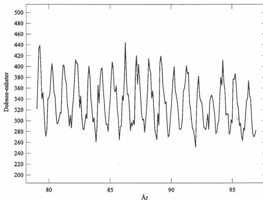
Figur 13: Månedsmidler av ozonmengden over Oslo 1979 til 1996 målt med Dobson- og Brewer-instrumentene basert på månedsmidler.
