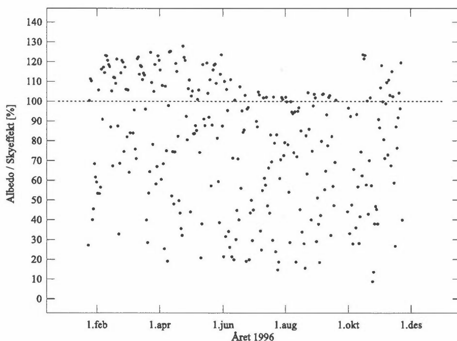
Figur 27: Effekter av skyer og bakkealbedo på UV-stråling ved jordens overflate i Tromsø i 1996 i prosent av klarværsverdien med null bakkerefleksjon. Hvert punkt representerer middelverdien mellom 10:30 og 11:30 GMT for en bestemt dag. Den horisontale linjen representerer klarvær og barmark. Verdier over denne linjen betyr at skyer og/eller bakkealbedo øker UV-nivået sammenlignet med klarvær og bar bakke.
