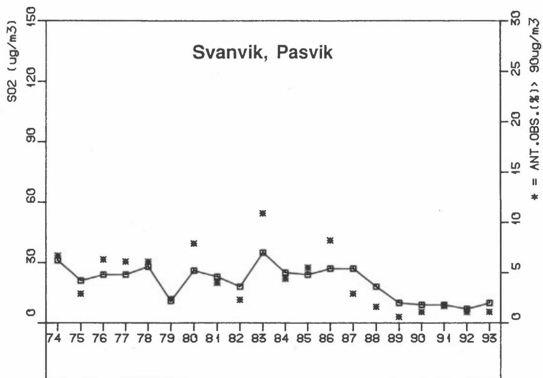
Figur 6: Sommermiddelkonsentrasjoner av SO 2 (µg/m 3 ) og frekvens av døgnmiddelverdier over 90 µg/m 3 i Kirkenes og Svanvik.
