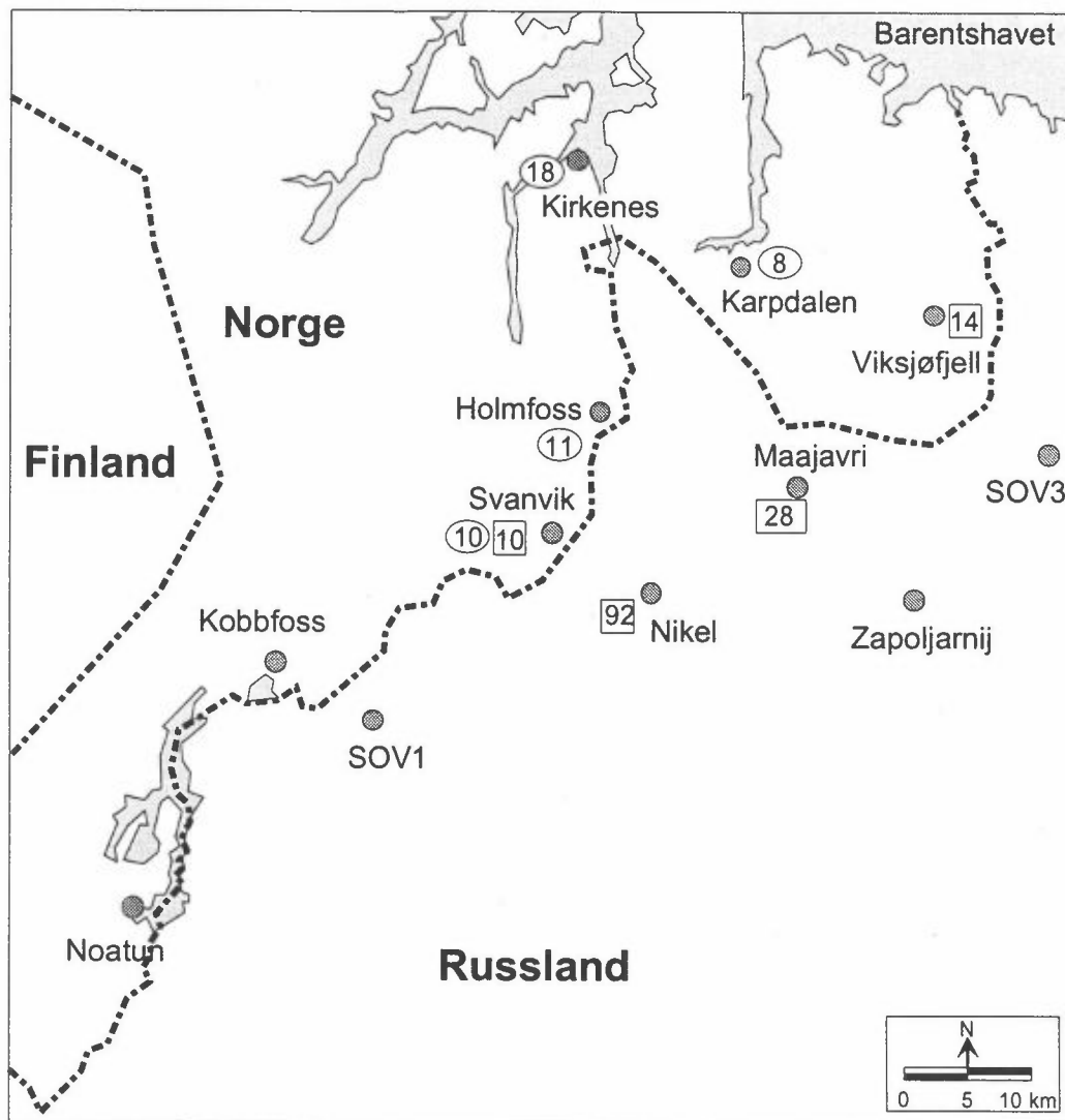
Figur 5: Middelkonsentrasjoner av \text{SO}_2 i perioden april-september 1993 målt med kontinuerlig registrerende prøvetakere \square og døgnprøvetakere \circ ( \mu\text{g}/\text{m}^3 ).
