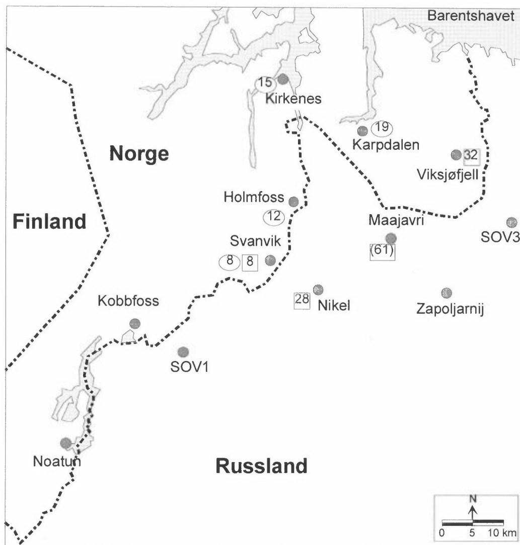
Figur 5: Middelkonsentrasjoner av SO 2 i perioden oktober 1993-mars 1994 målt med kontinuerlig registrerende prøvetakere □ og døgnsprøvetakere ○ (µg/m 3 ).
