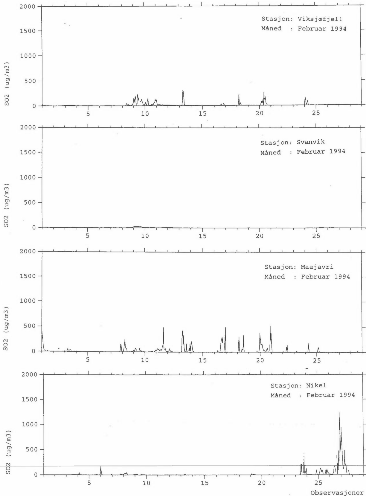
Figur 16: Timemiddelkonsentrasjoner av SO 2 i februar 1994 fra Viksjøfjell, Svanvik, Maajavri og Nikel ( \mu\text{g}/\text{m}^3 ).
