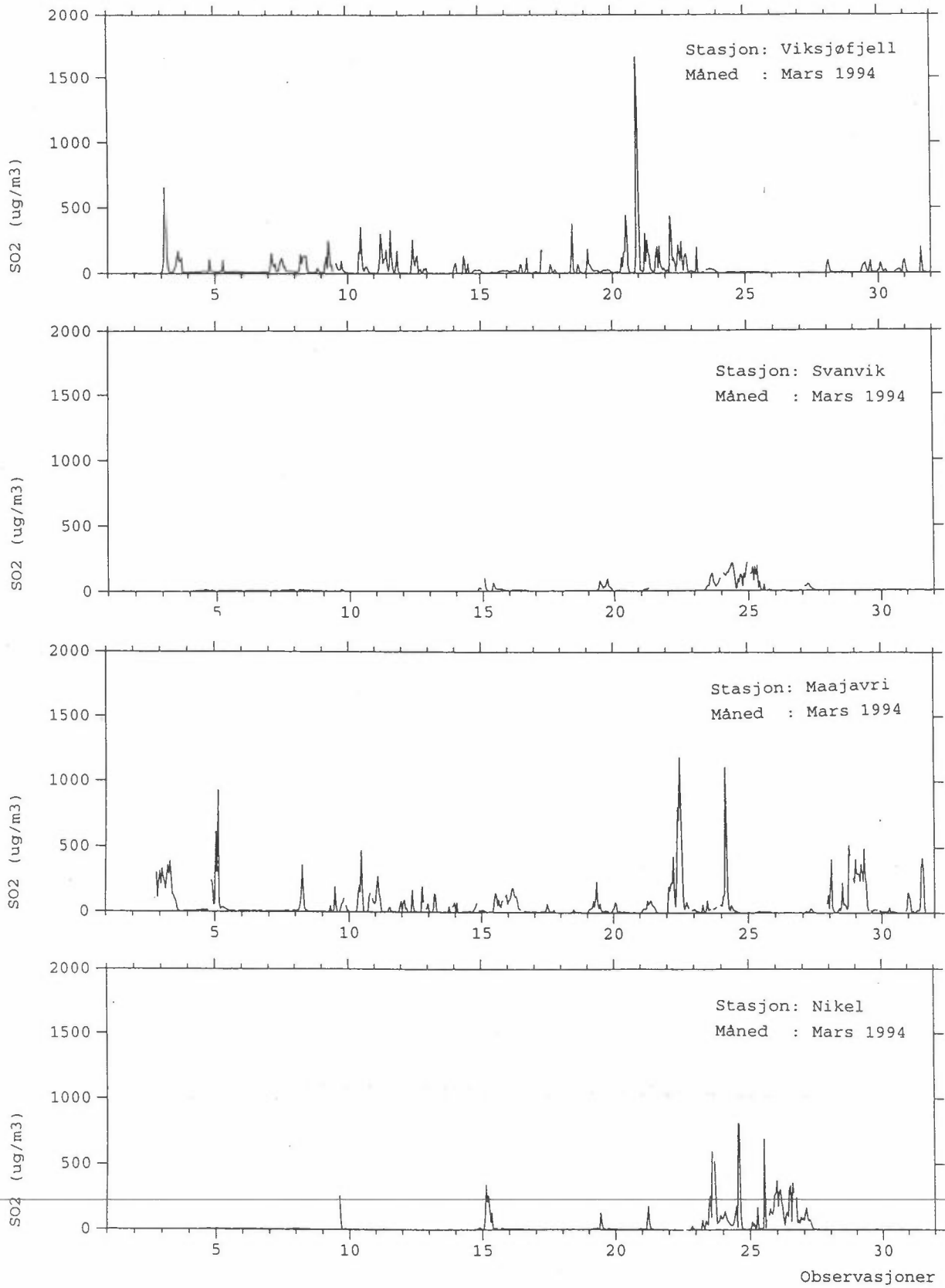
Figur 17: Timemiddelkonsentrasjoner av SO 2 i mars 1994 fra Viksjøfjell, Svanvik, Maajavri og Nikel (µg/m 3 ).
