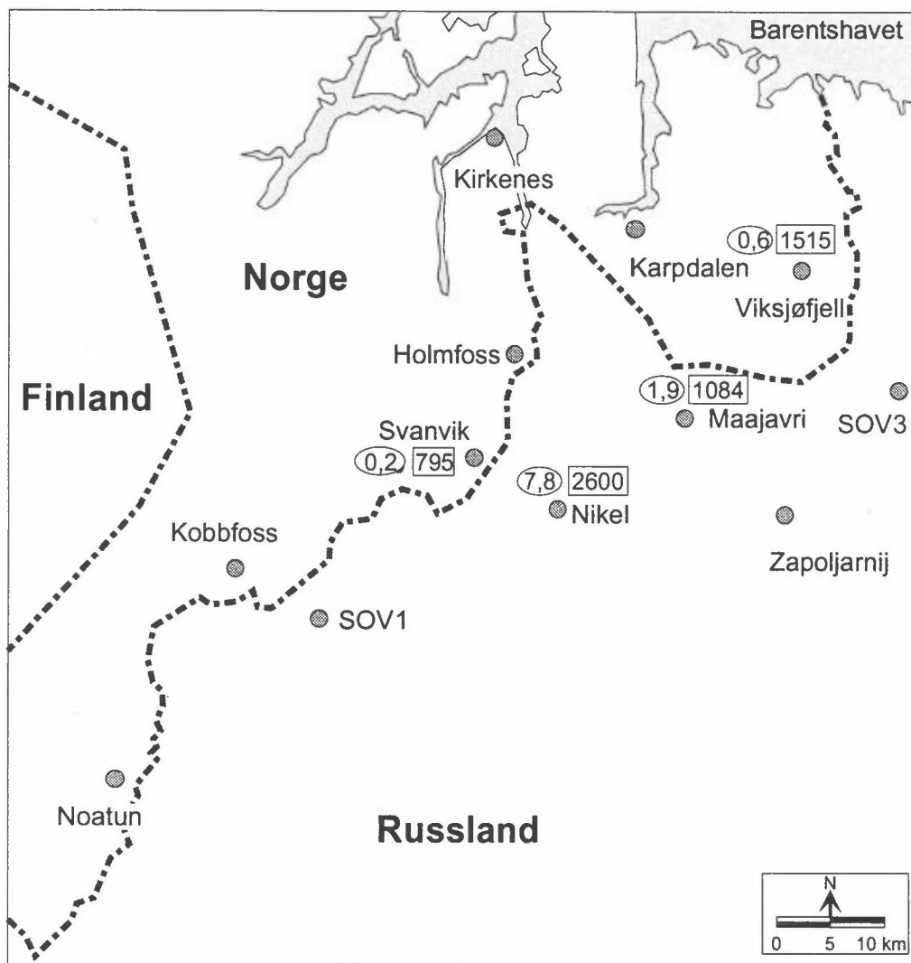
Figur 18: Maksimale timemiddelverdier av \text{SO}_2 \square ( \mu\text{g}/\text{m}^3 ) og prosent av tiden med timemiddelverdier over 350 \mu\text{g}/\text{m}^3 \circ i perioden april-september 1993.
