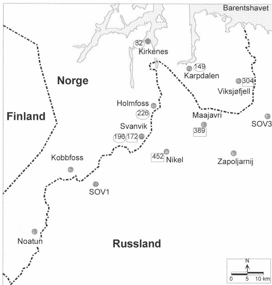
Figur 9: Maksimale døgnmiddelkonsentrasjoner av SO 2 i perioden oktober 1993-mars 1994 målt med kontinuerlig registrerende prøvetakere og døgnprøvetakere (µg/m 3 ).
