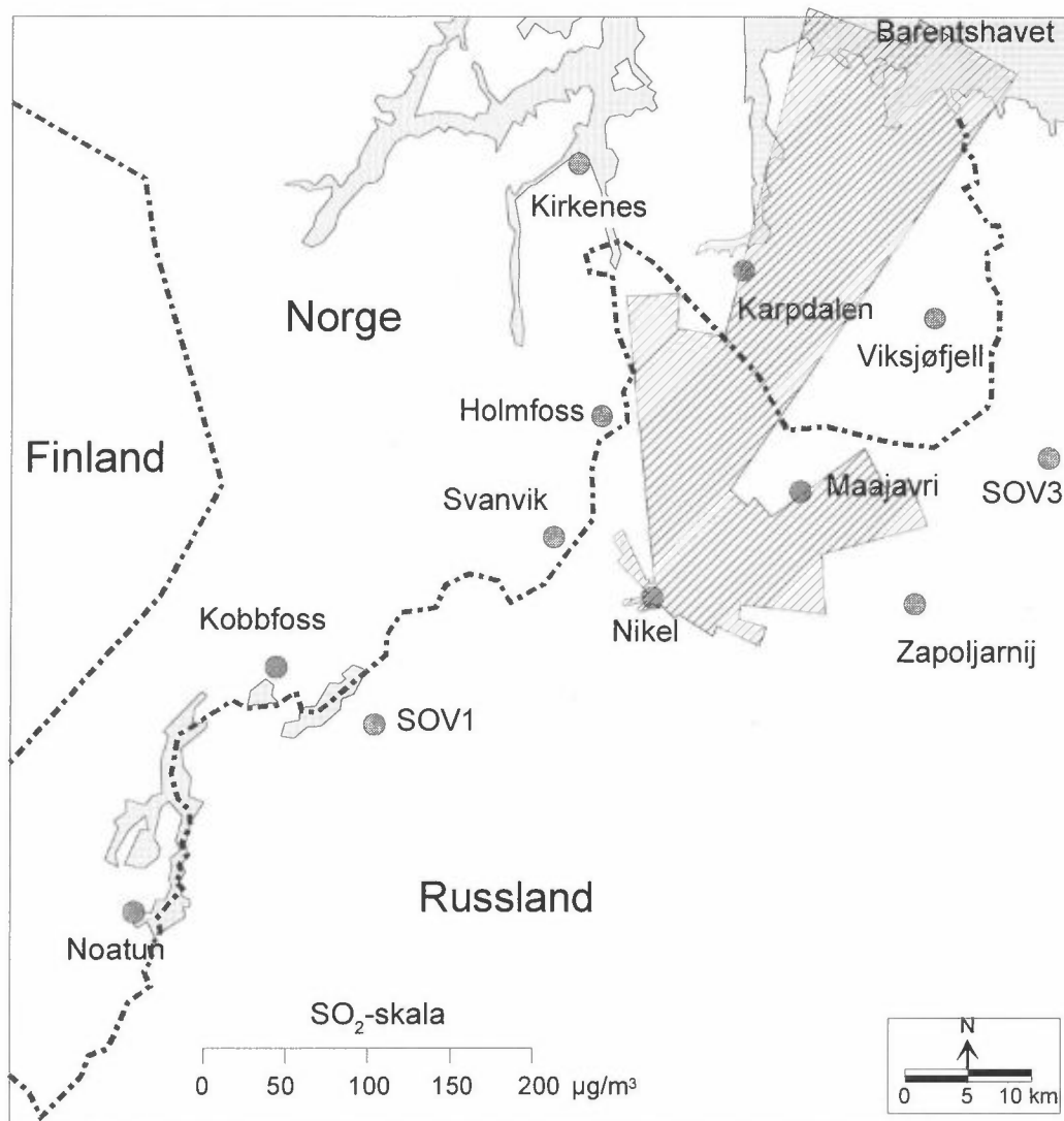
Figur 11: Middelskonsentrasjoner av SO_2 i Nikel (samme skala som i figur 10) i 36 vindsektorer i perioden oktober 1993-mars 1994 ( \mu\text{g}/\text{m}^3 ).
