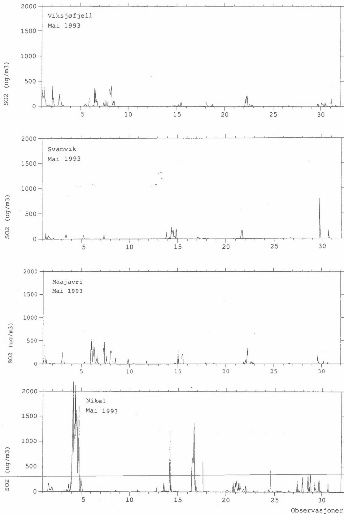
Figur 13: Timemiddelkonsentrasjoner av \text{SO}_2 i mai 1993 fra Viksjøfjell, Svanvik, Maajavri og Nikel ( \mu\text{g}/\text{m}^3 ).
