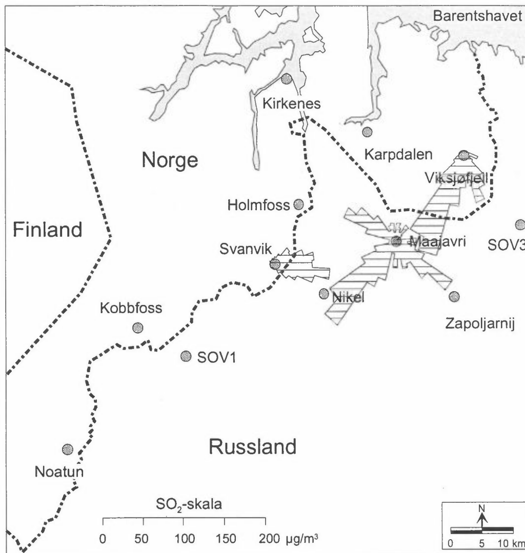
Figur 10: Middelkonsentrasjoner av SO_2 for Viksjøfjell, Svanvik, og Maajavri i 36 vindsektorer i perioden april-september 1993 ( \mu\text{g}/\text{m}^3 ).
