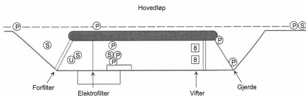
Figur C1: Plassering av støvprøvetakere (S), sporstoffprøvetakere (P) og sporgassutslipp (U) i området ved rensesløyfa.
