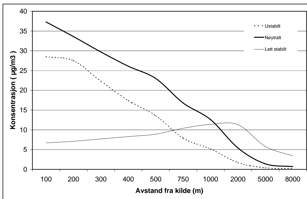
Figur 2b: Halv last (50%). NO 2 -bidrag til bakkekonsentrasjon. Røykgassmengde 10 960 Nm 3 /h, og avgasshastighet 9,5 m/s.
