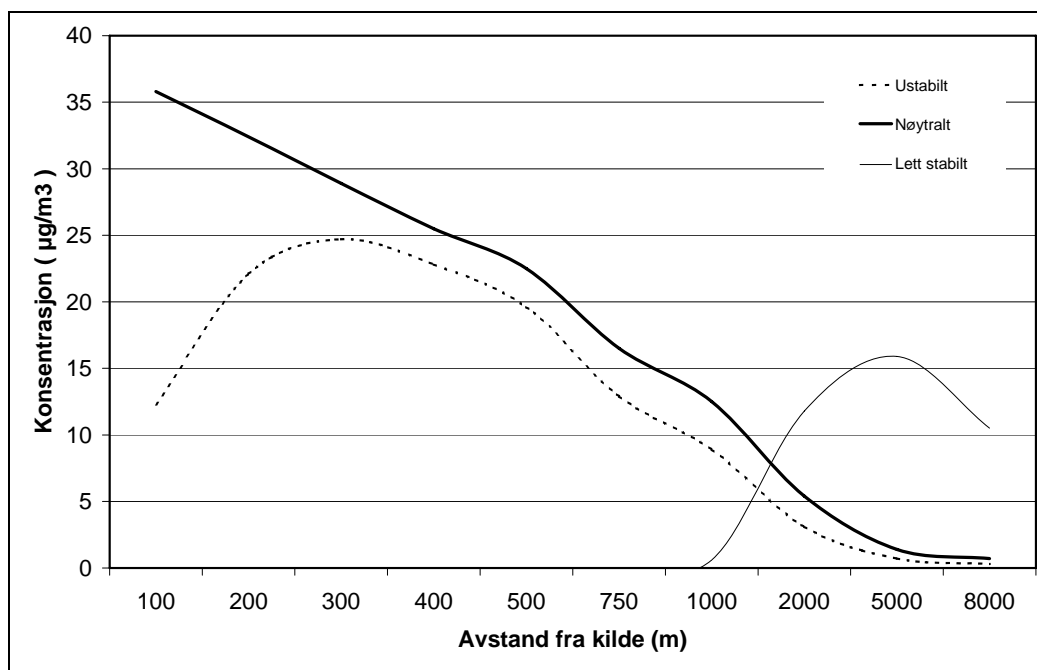
Figur 2a: Full last (100%). NO 2 -bidrag til bakkekonsentrasjon. Røykgassmengde 22 115 Nm 3 /h, og avgasshastighet 19,5 m/s.
