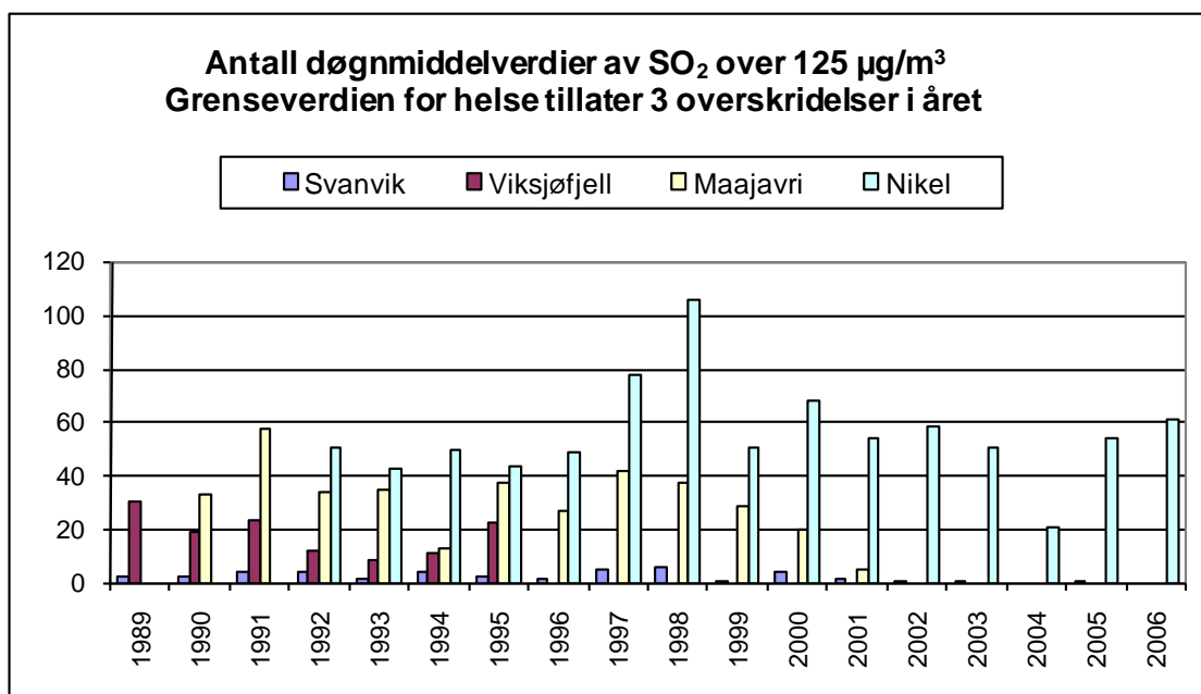
Figur 10: Antall døgnmiddelverdier av SO 2 over grenseverdien på 125 µg/m 3 i Svanvik (1989-2006), på Viksjøfjell (1989-1995), i Maajavri (1990-2001) og i Nikel (1992-2006) (3 tillatte overskridelser i året).
