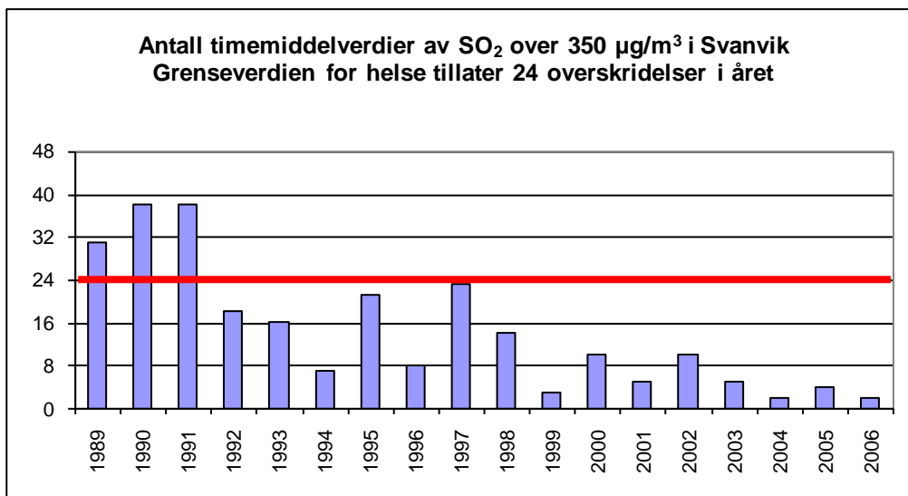
Figur 14: Antall timemiddelverdier av SO 2 over grenseverdien på 350 µg/m 3 i Svanvik i årene 1989-2006 (24 tillatte overskridelser i året).
