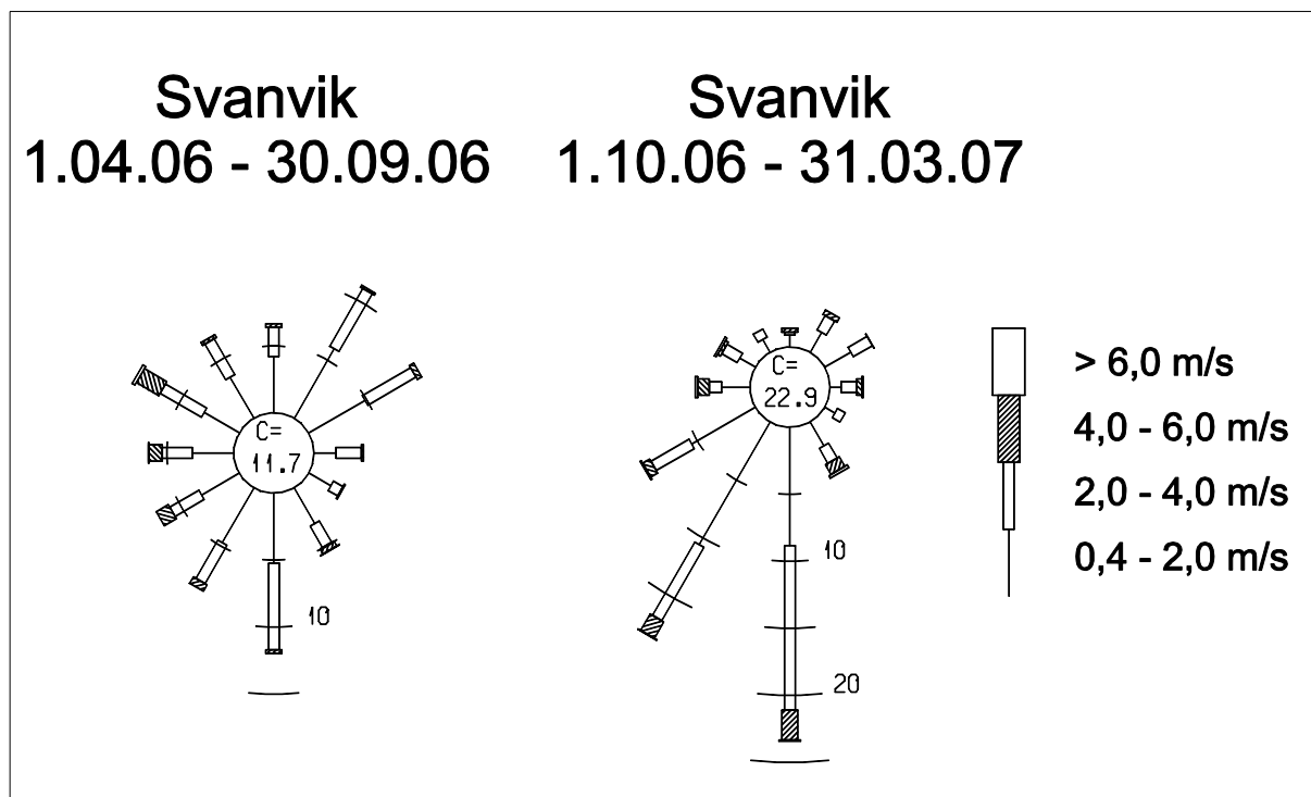
Figur 2: Vindroser fra Svanvik for periodene april-september 2006 og oktober 2006-mars 2007. (Vindrosene viser frekvensen av vind i tolv 30-graders sektorer, dvs. hvor ofte det blåser fra disse retningene).
