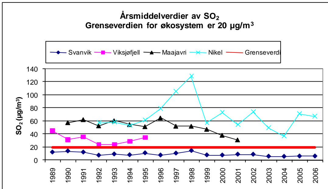
Figur 6: Årsmiddelverdier av SO 2 i Svanvik (1989-2006), på Viksjøfjell (1989-1995), i Maajavri (1990-2001) og i Nikel (1992-2006) (µg/m 3 ).
