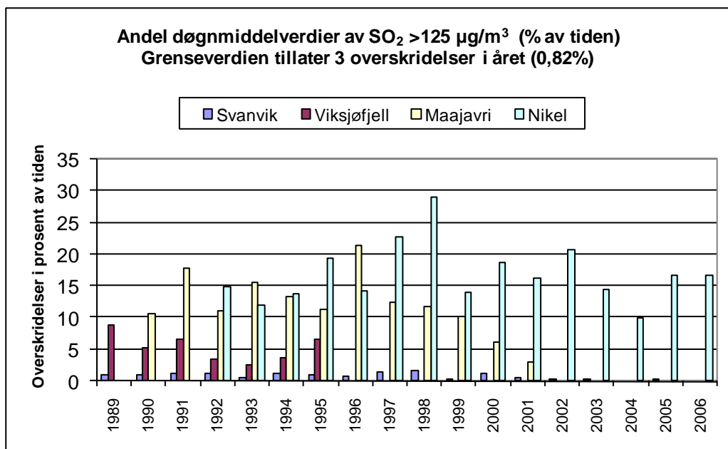
Figur 11: Andel av tiden grenseverdien for døgnmiddel av SO 2 på 125 µg/m 3 er overskredet i Svanvik (1989-2005), på Viksjøfjell (1989-1995), i Maajavri (1990-2001) og i Nikel (1992-2006) (3 tillatte overskridelser i året tilsvarer 0,82% av tiden).
