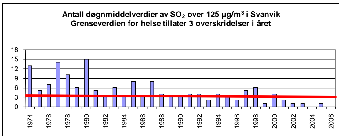
Figur 9: Antall døgnmiddelverdier av SO 2 over grenseverdien på 125 µg/m 3 i Svanvik i årene 1974-2006 (3 tillatte overskridelser i året).
