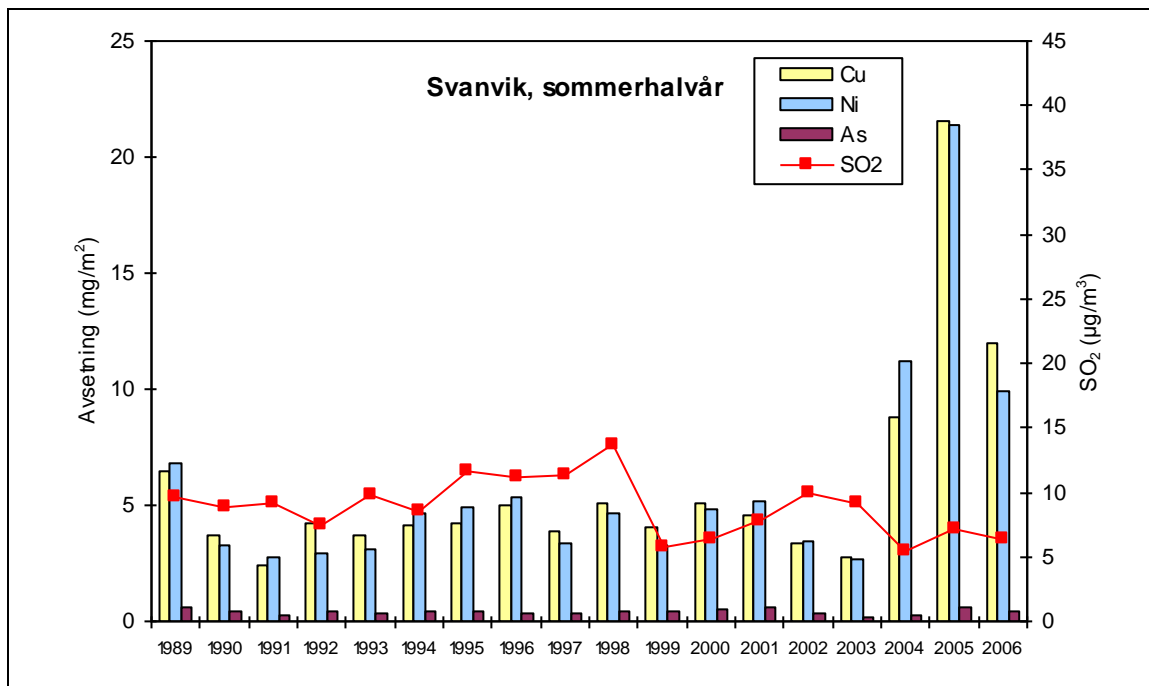
Figur 17: Avsetning med nedbør av Cu, Ni og As ( \text{mg}/\text{m}^2 ) i sommerhalvårene fra 1989 til 2006 og i vinterhalvårene fra 1988/89 til 2006/07. Halvårsmiddelkonsentrasjonene av \text{SO}_2 er også vist ( \mu\text{g}/\text{m}^3 ).
