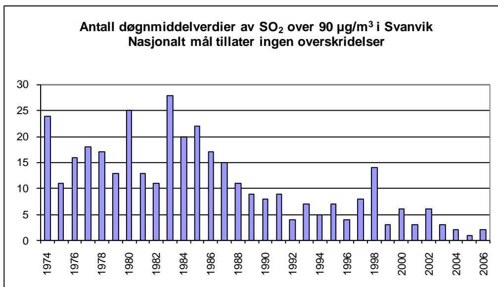
Figur 12: Antall døgnmiddelverdier av SO 2 over Nasjonalt mål på 90 µg/m 3 i Svanvik i årene 1974-2006 (ingen tillatte overskridelser).
