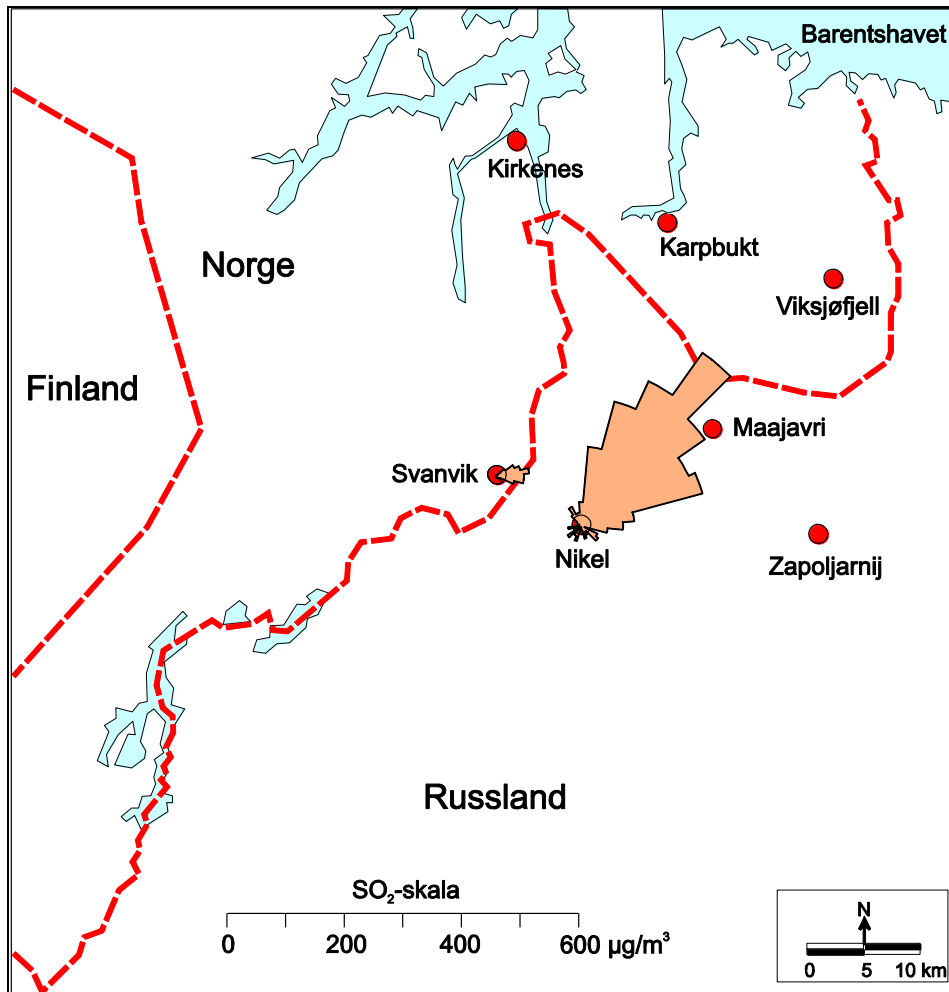
Figur 3: Middelkonsentrasjoner av \text{SO}_2 i Svanvik og Nikel i perioden april-september 2006 ( \mu\text{g}/\text{m}^3 ). Figuren viser middelkonsentrasjoner av \text{SO}_2 for hver av 36 10^\circ -vindsektorer. Begge stasjonene er mest belastet når det blåser fra smelteverket i Nikel.
