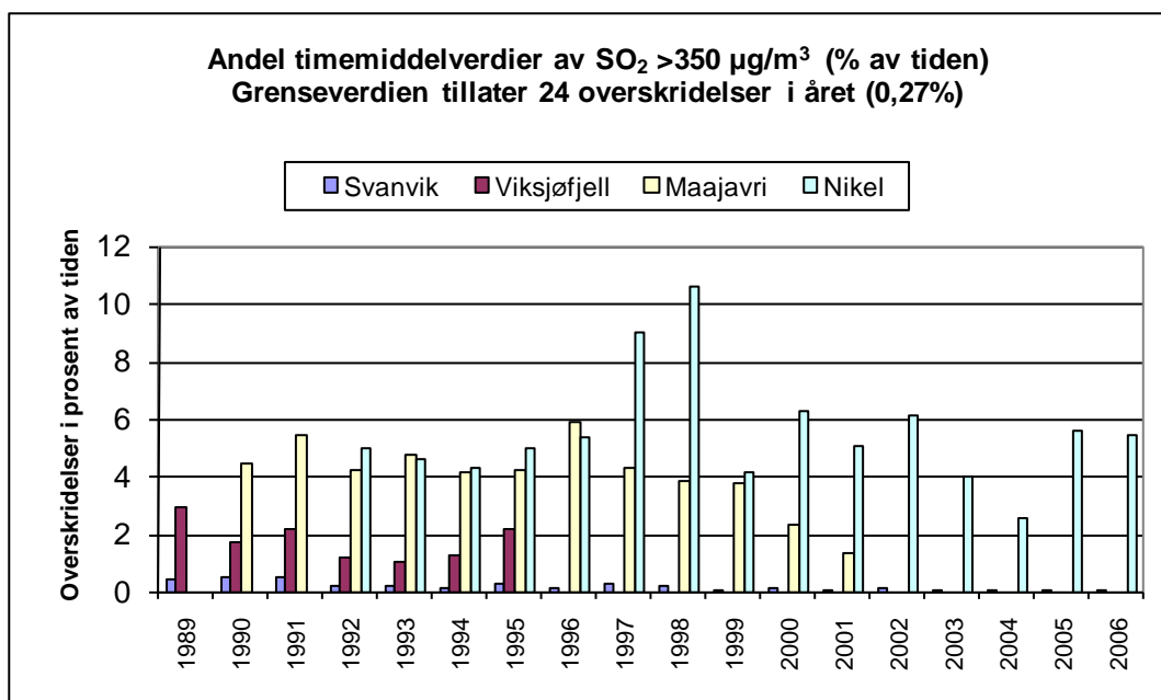
Figur 16: Andel av tiden grenseverdien for timemiddel av SO 2 på 350 µg/m 3 er overskredet i Svanvik (1989-2006), på Viksjøfjell (1989-1995), i Maajavri (1990-2001) og i Nikel (1992-2006) (24 tillatte overskridelser i året tilsvarer 0,27% av tiden).
