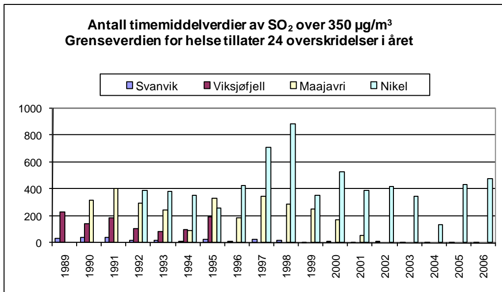
Figur 15: Antall timemiddelverdier av SO 2 over grenseverdien på 350 µg/m 3 i Svanvik (1989-2006), på Viksjøfjell (1989-1995), i Maajavri (1990-2001) og i Nikel (1992-2006) (24 tillatte overskridelser i året).
