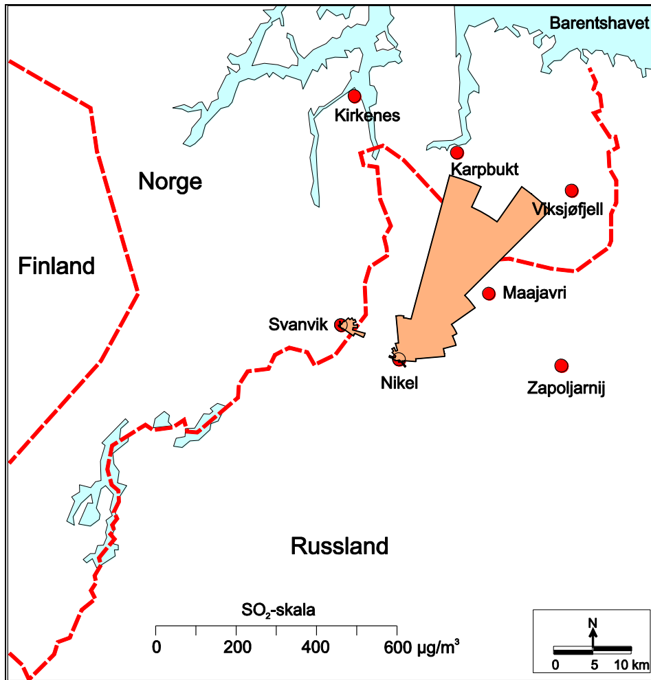
Figur 4: Middelkonsentrasjoner av SO 2 i Svanvik og Nikel i perioden oktober 2006-mars 2007 (µg/m 3 ). Figuren viser middelkonsentrasjoner av SO 2 for hver av 36 10 o -vindsektorer. Begge stasjonene er mest belastet når det blåser fra smelteverket i Nikel.
