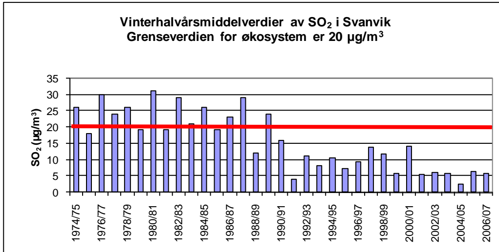
Figur 7: Vinterhalvårsmiddelverdier av SO 2 i Svanvik 1974/75-2006/07 (µg/m 3 ).
