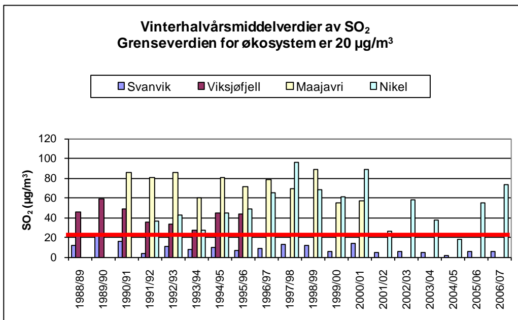
Figur 8: Vinterhalvårsmiddelverdier av SO 2 i Svanvik (1988/89-2006/07), på Viksjøfjell (1988/89-1995/96), i Maajavri (1990/91-2000/01) og i Nikel (1991/92-2006/07) (µg/m 3 ).
