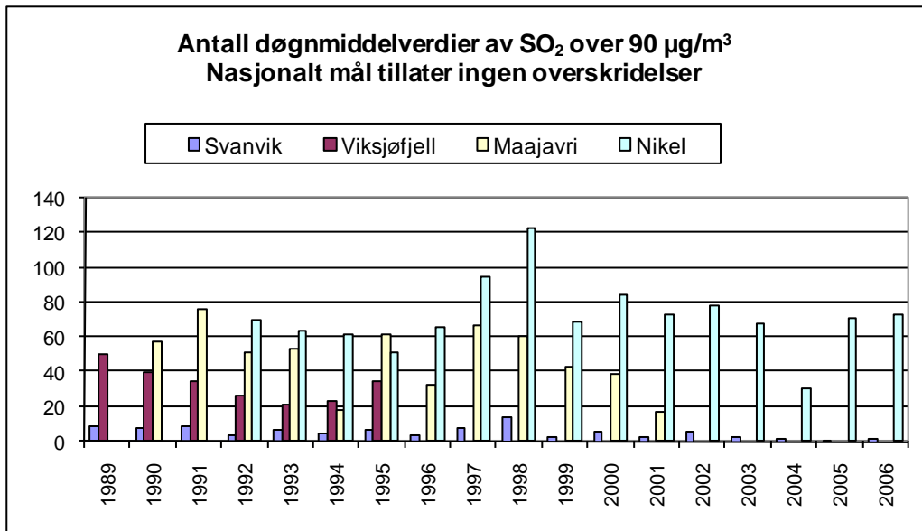
Figur 13: Antall døgnmiddelverdier av SO 2 over Nasjonalt mål på 90 µg/m 3 i Svanvik (1989-2006), på Viksjøfjell (1989-1995), i Maajavri (1990-2001) og i Nikel (1992-2006) (ingen tillatte overskridelser).
