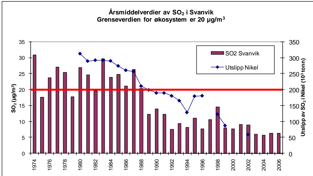
Figur 5: Årsmiddelverdier av SO 2 i Svanvik i årene 1974-2006 (µg/m 3 ).
