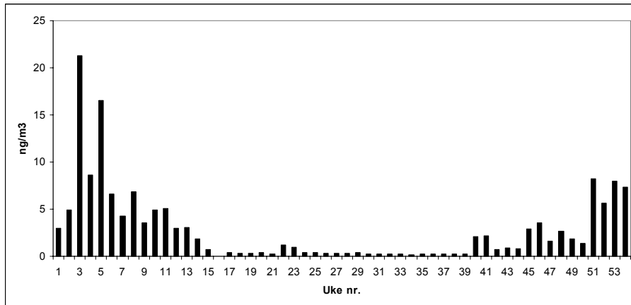
Figur 5.21: Ukentlig luftkonsentrasjon av sum PAH (38 PAH komponenter) på Zeppelinfjellet i 2003.
