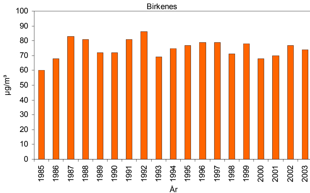
Figur 4.9: Middelskonsentrasjon av ozon for 7 timer (kl. 09-16) i vekstsesongen (april-september) ved Birkenes i perioden 1985-2003.
