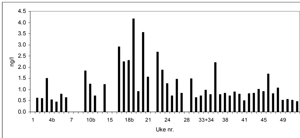
Figur 5.8: Nedbørkonsentrasjon av HCH (sum \alpha - og \gamma -HCH) i prøver samlet ukentlig på Lista i år 2003. Manglende data representerer uker uten tilstrekkelig nedbør. I en del tilfeller ble flere målinger gjort i løpet av en uke og i slike tilfeller ble prøvene nummerert med ukenummer og en bokstav, f.eks. 4a og 4b. I noen tilfeller ble prøver fra flere uker analysert som samleprøve og slike er nummerert som uke1 + uke2, f.eks 33+34.
