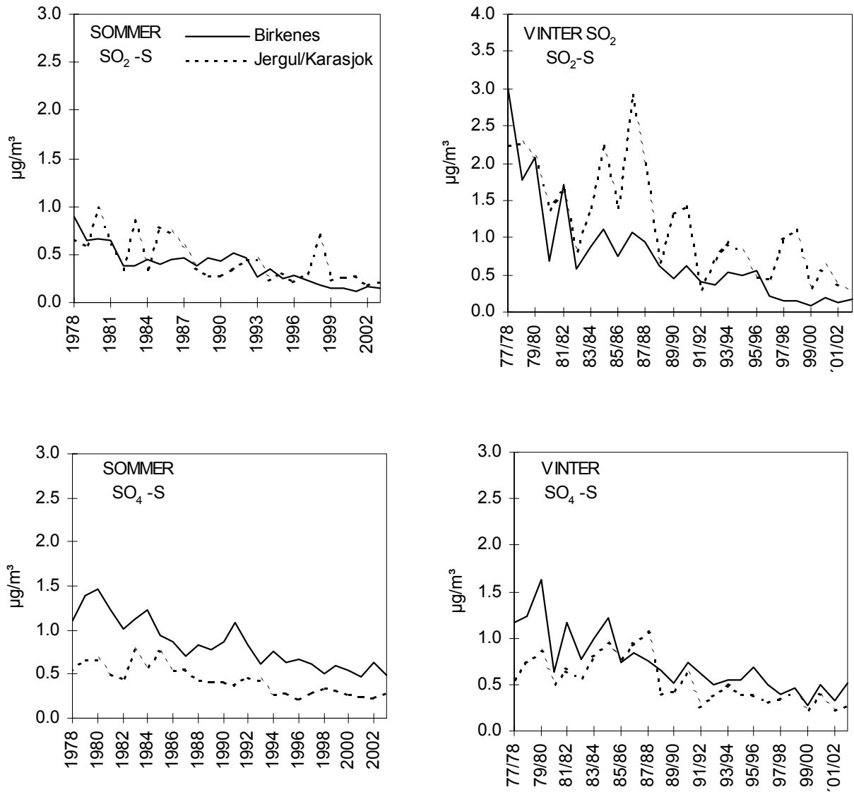
Figur 3.8: Middelskonsentrasjoner av partikulært sulfat og svoveldioksid i luft for vinterhalvårene 1977/1978 – 2002/2003 (oktober-mars) og sommerhalvårene 1978-2003 på Birkenes og Jergul/Karasjok.
