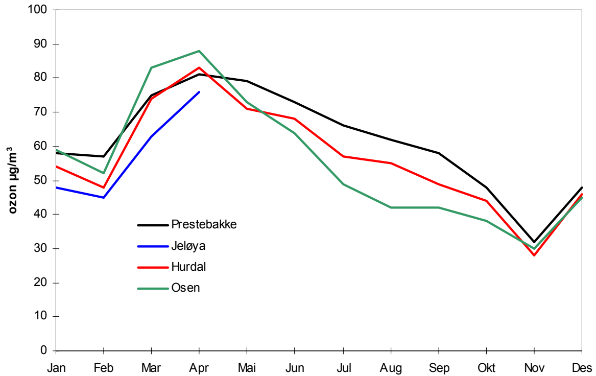
Figur 4.1: Månedsmiddeler av ozon 2003 ( \mu\text{g}/\text{m}^3 ) for Prestebakke, Jeløya, Hurdal og Osen.
