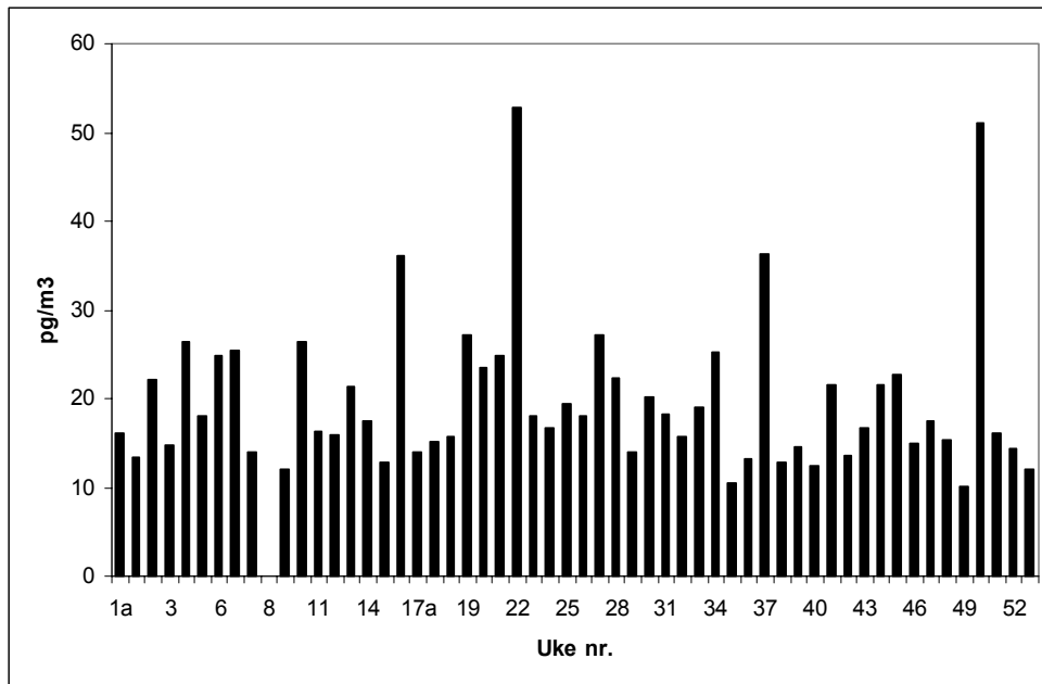
Figur 5.19: Ukentlig luftkonsentrasjon av sum tri- til dekalor PCB på Zeppelinfjellet i 2003.
