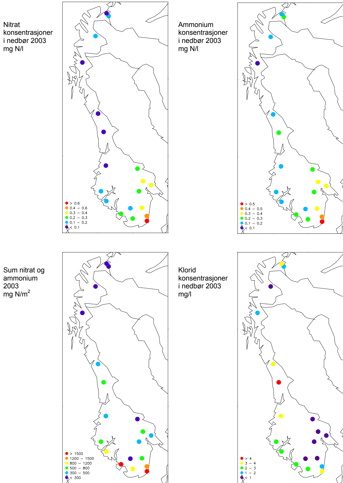
Figur 1.2: Middelskonsentrasjoner i nedbør av nitrat, ammonium og klorid, og våtavsetning av total nitrogen (nitrat + ammonium) på norske bakgrunnsstasjoner i 2003.
