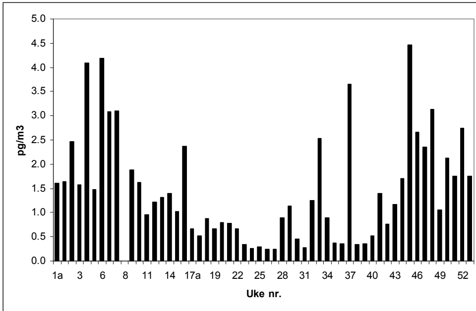
Figur 5.15: Ukentlig luftkonsentrasjon av "sum DDT" (sum o,p'-DDE, p,p'-DDE, o,p'-DDD, p,p'-DDD, o,p'-DDT og p,p'-DDT) på Zeppelifjellet i 2003. I en del tilfeller ble flere målinger gjort i løpet av en uke. I slike tilfeller ble prøvene nummerert med ukenummer og en bokstav, f.eks. 1a og 1b.
