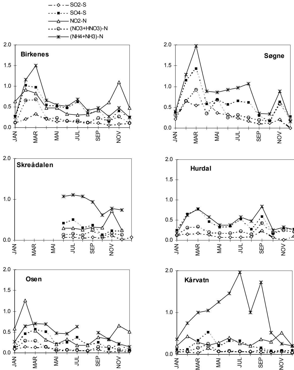
Figur 3.1: Månedlige middelkonsentrasjoner av svoveldioksid, partikulært sulfat, nitrogen-dioksid, (ammonium+ammoniakk) og (nitrat+salpetersyre) i luft på norske bakgrunnsstasjoner i 2003. Enhet: \mu\text{g}/\text{m}^3 .
