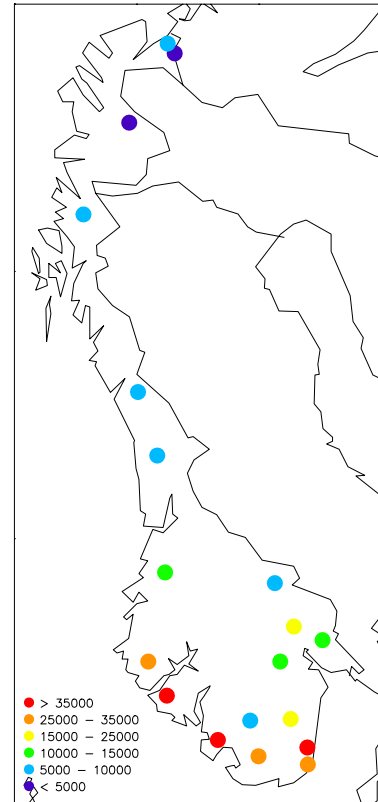
Figur 1.1: Middelkonsentrasjoner i nedbør og våtavsetning av sulfat (sjøsaltkorrigert) og sterk syre (pH) på norske bakgrunnsstasjoner i 2003.
