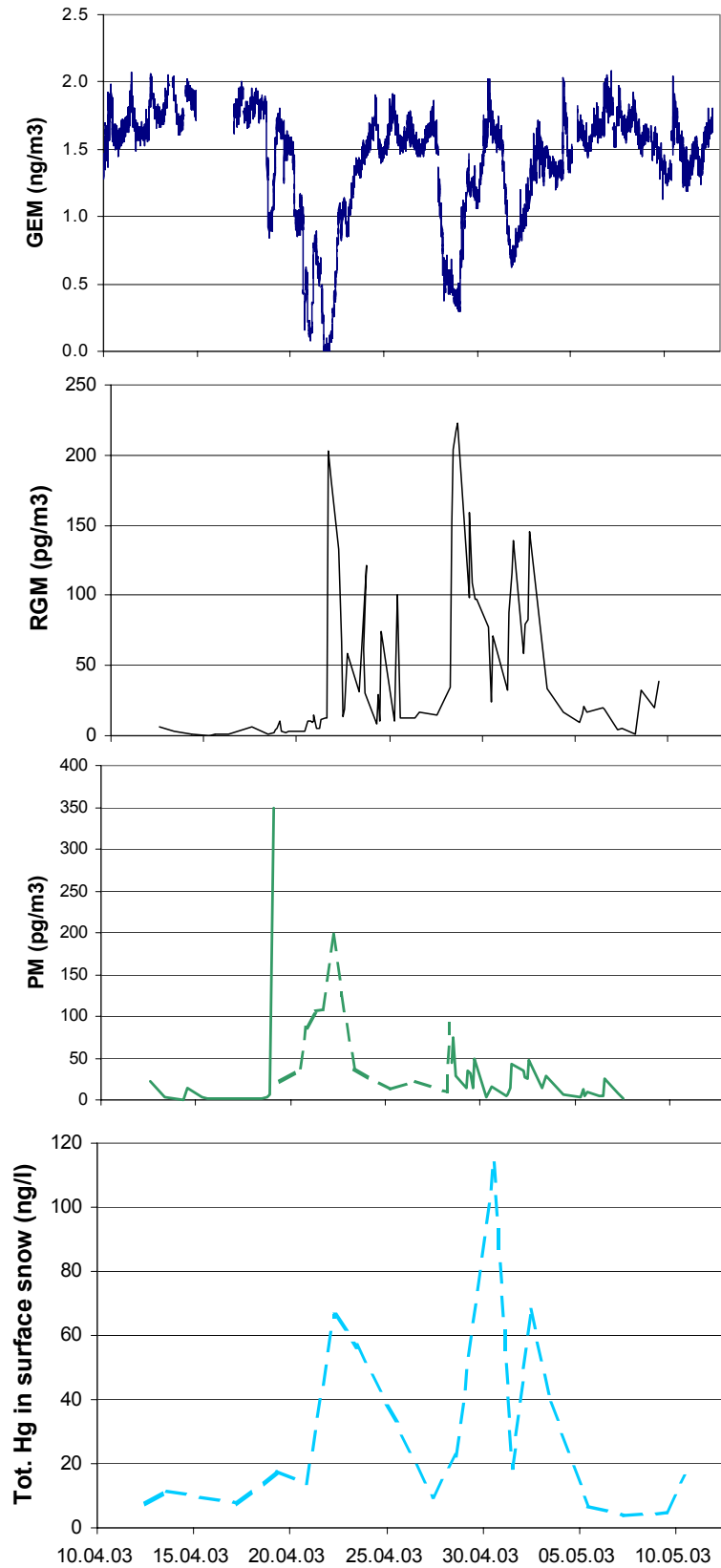
Figur 5.10: Tidsserier for elementært kvikksølv i gassfase (GEM), reaktivt gassfasekvikksølv (RGM), partikulært kvikksølv og kvikksølv i overflatesnø ved Ny-Ålesund, våren 2003.
