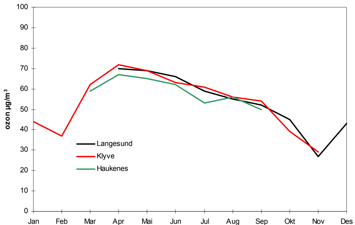
Figur 4.2: Månedsmiddeler av ozon 2003 ( \mu\text{g}/\text{m}^3 ) for Langesund, Klyve og Haukenes.
