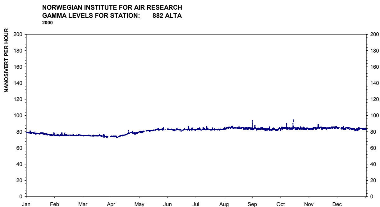
Figur 7 Årsplott av stasjon 882, Alta.
