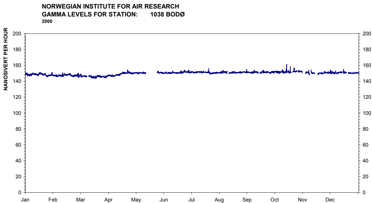
Figur 15: Årsplott av stasjon 1038, Bodø.
