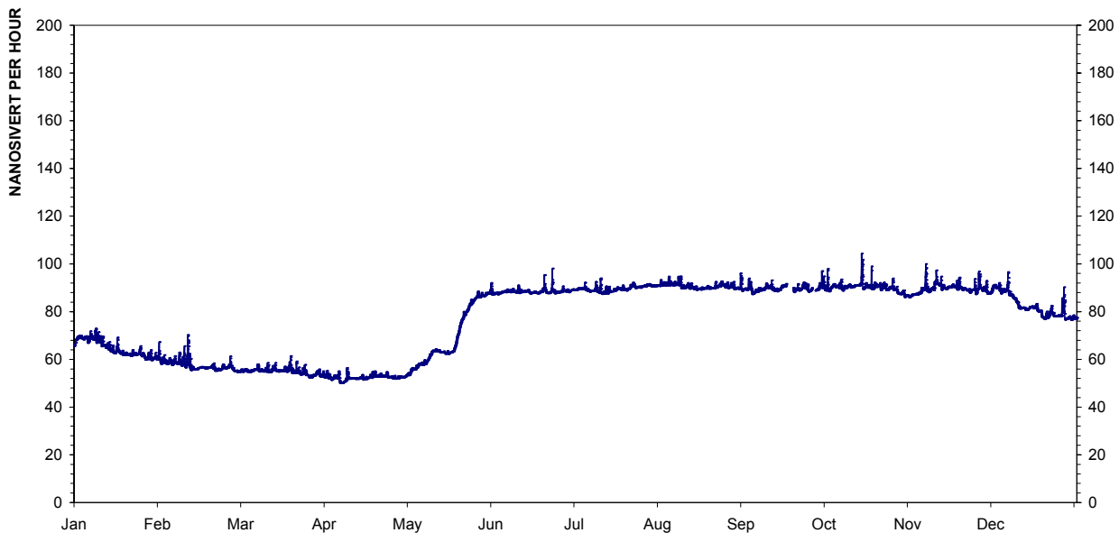
Figur 3: Årsplott av stasjon 887, Mehamn.
