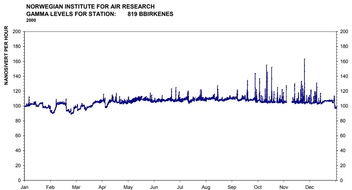
Figur 31: Årsplott av stasjon 819, BBirkenes.
