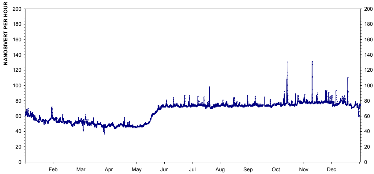
Figur 16: Årsplott av stasjon 215, Tustervatn.
