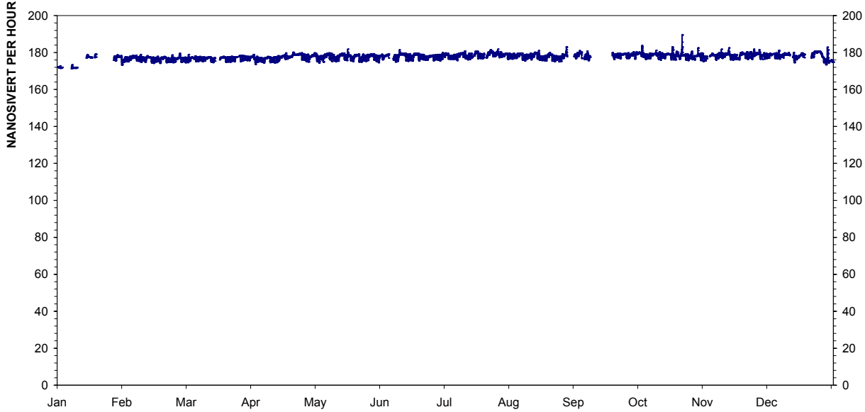
Figur 28: Årsplott av stasjon 1035, Stavanger.
