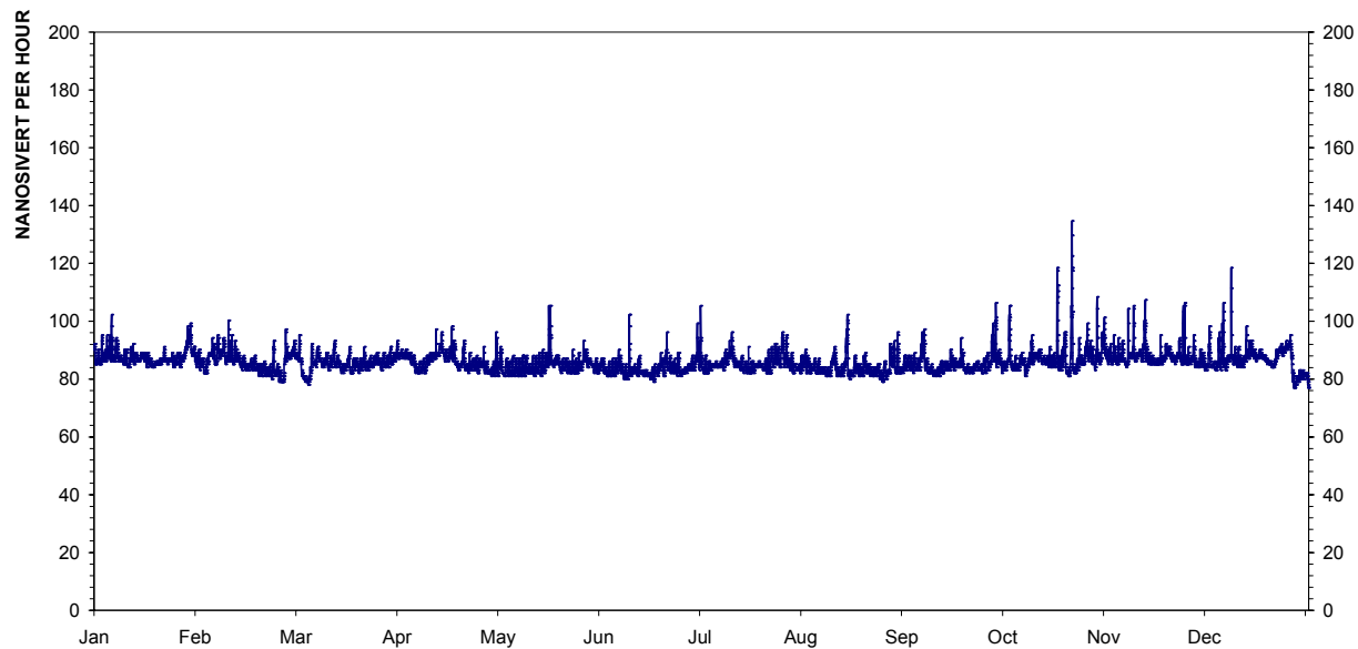
Figur 26: Årsplott av stasjon 572, Vikedal.
