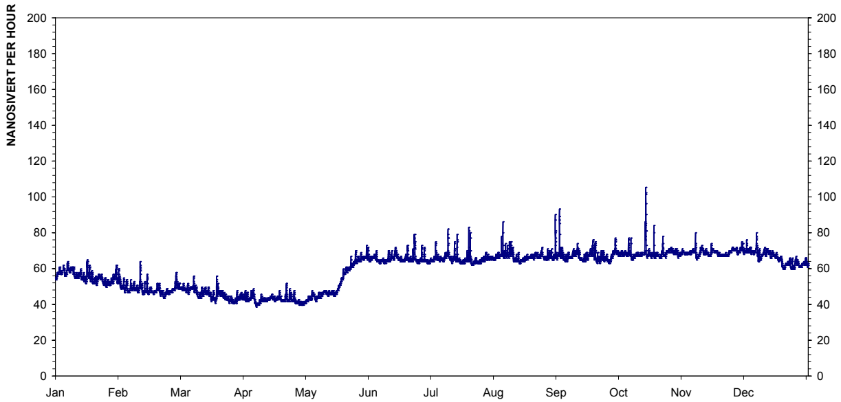
Figur 12: Årsplott av stasjon 477, Øverbygd.
