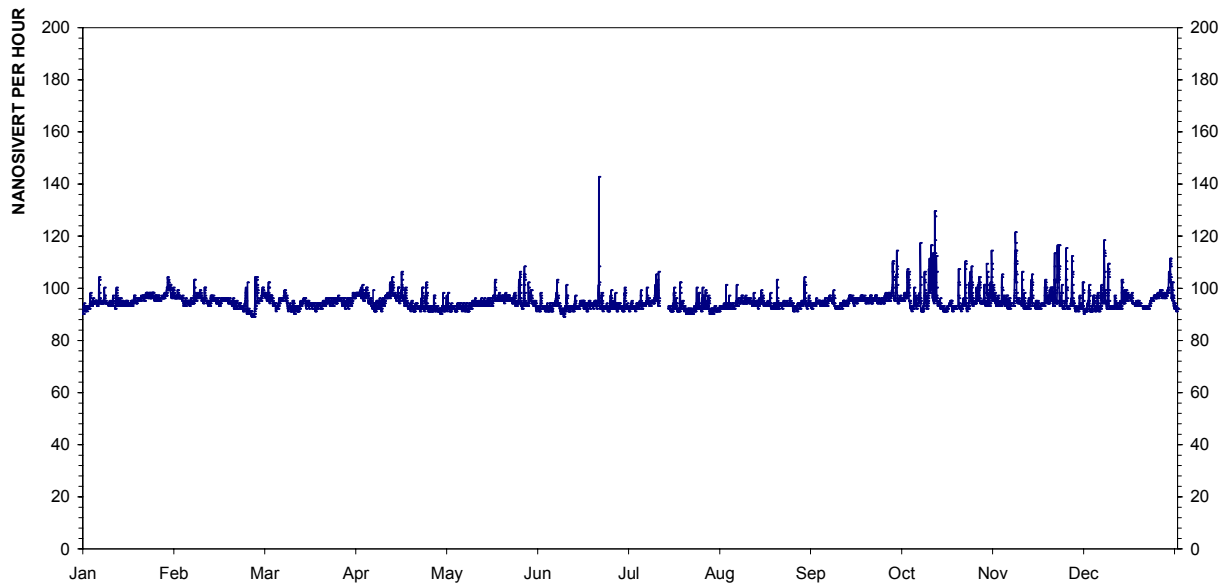
Figur 27: Årsplott av stasjon 689, Prestebakke.
