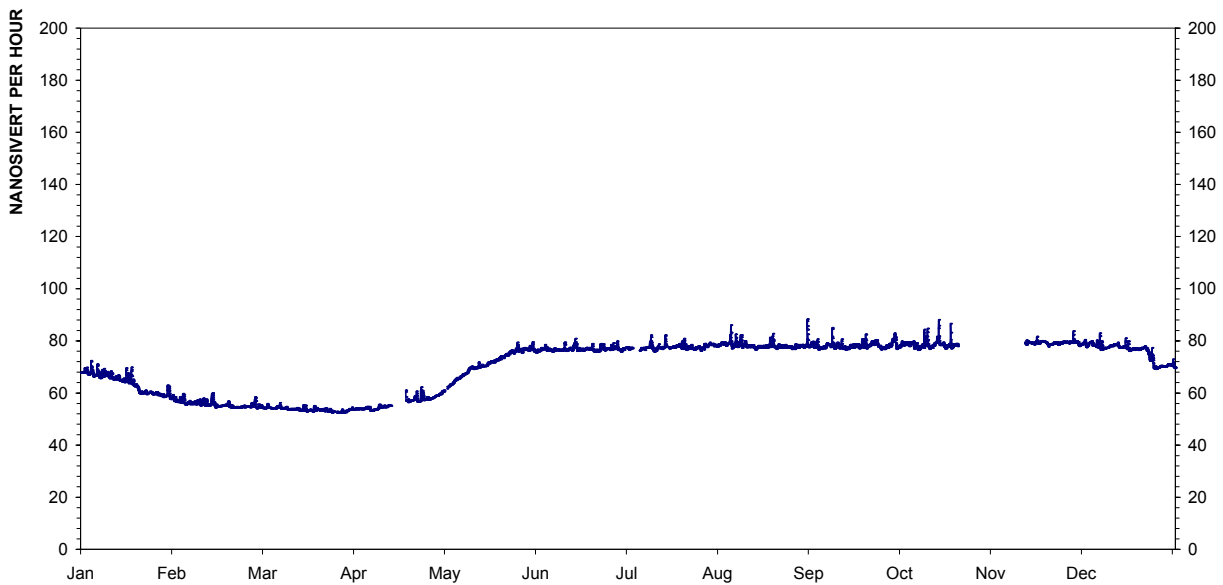
Figur 13: Årsplott av stasjon 880, Harstad.
