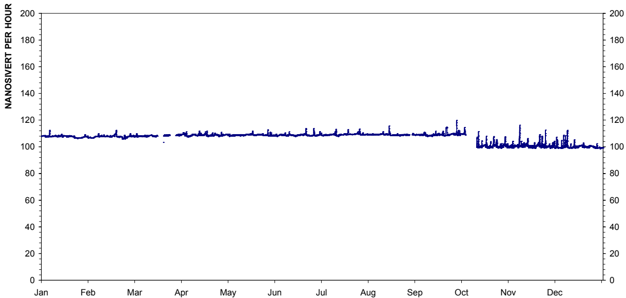
Figur 29: Årsplott av stasjon 1034, Grimstad.
