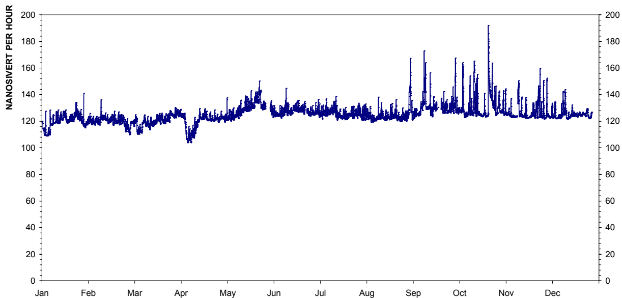
Figur 25: Årsplott av stasjon 983, NILU.
