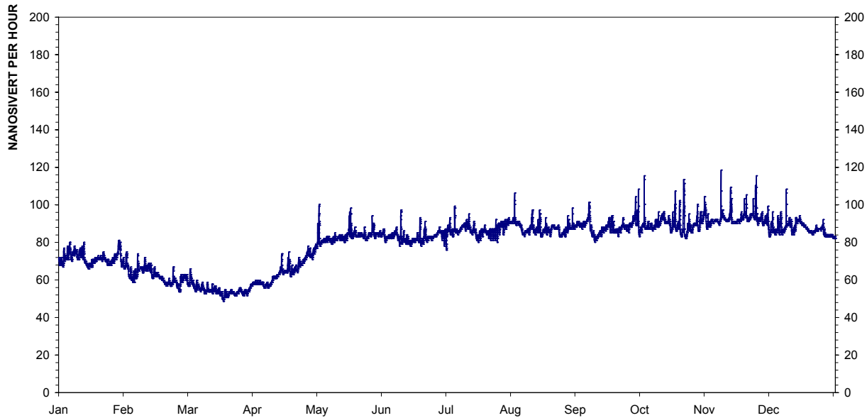
Figur 21: Årsplott av stasjon 655, Naustdal.
