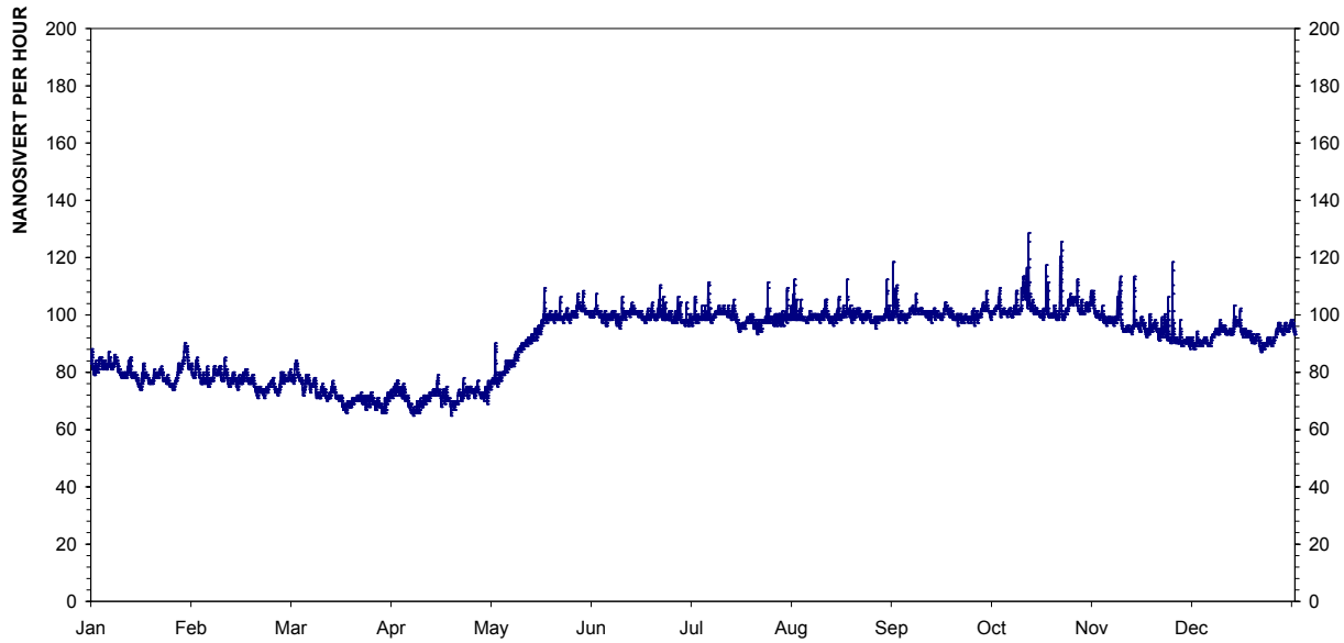
Figur 20: Årsplott av stasjon 756, Vålåsjø.
