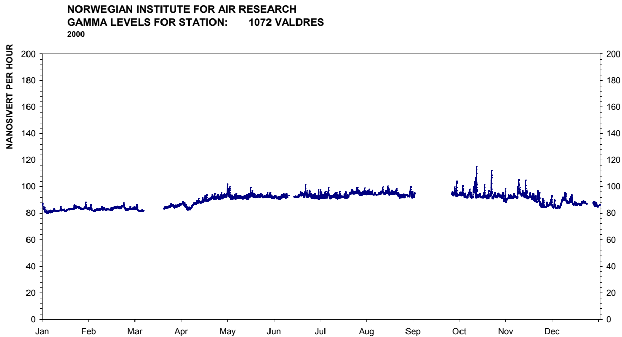
Figur 23: Årsplott av stasjon 1072, Valdres.
