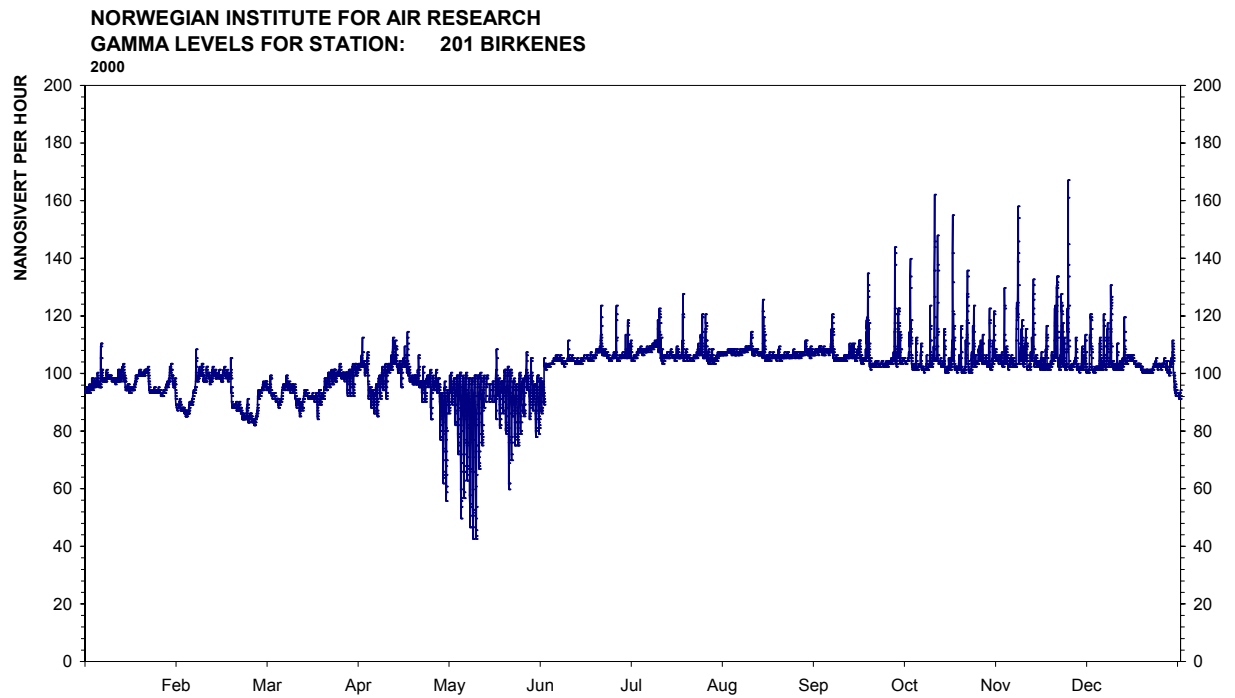
Figur 30: Årsplott av stasjon 201, Birkenes.
