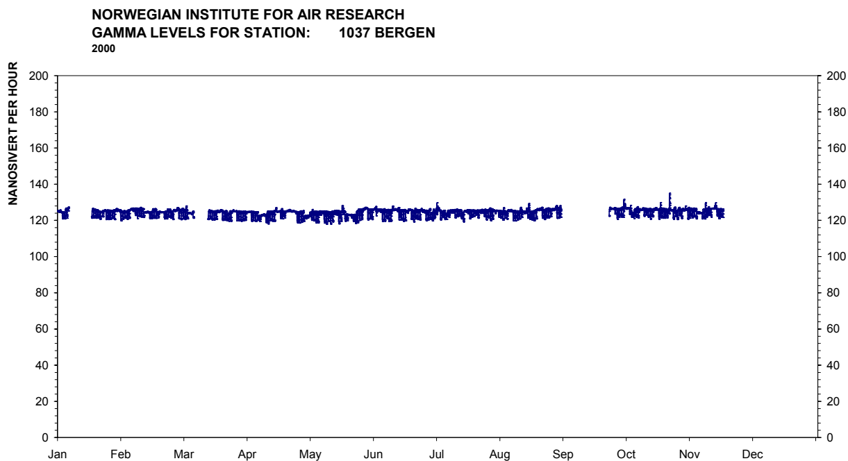
Figur 22: Årsplott av stasjon 1037, Bergen.
