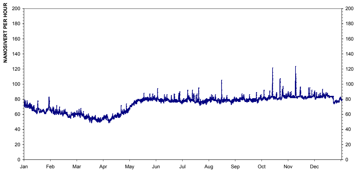
Figur 17: Årsplott av stasjon 478, Høylandet.
