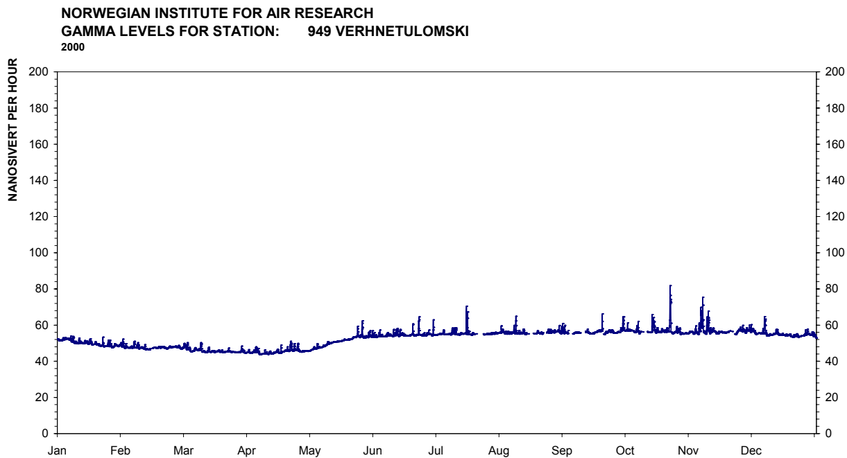
Figur 14: Årsplott av stasjon 949, Verhnetulomski.
