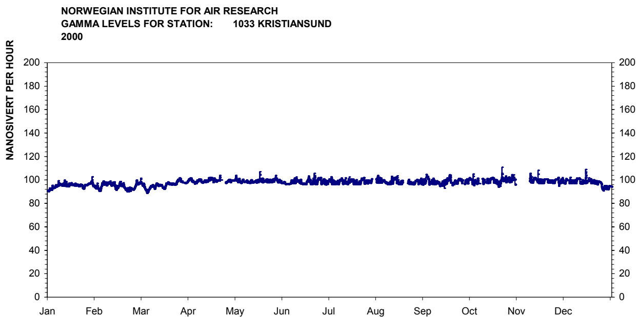
Figur 19: Årsplott av stasjon 1033, Kristiansund.
