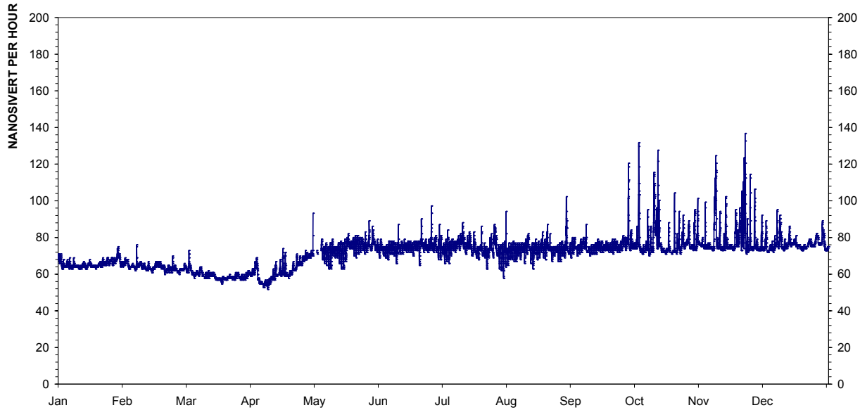
Figur 24: Årsplott av stasjon 312, Nordmoen.
