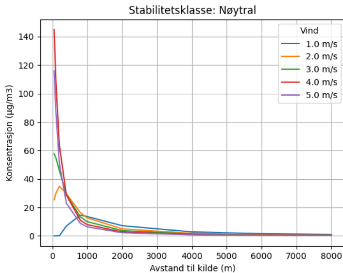
Figur 5-1 Konsentrasjonsprofil i avstand fra utslippskilden for nøytrale stabilitetsforhold for vindhastigheter fra 1 m/s til 5 m/s. Vindhastigheter over 5 m/s har lignende nivå og profil som denne vindhastigheten.
