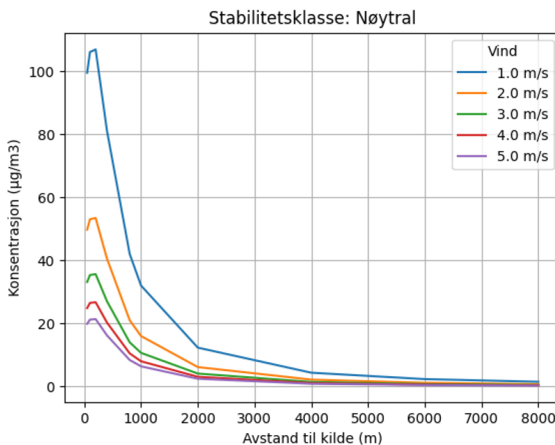
Figur 5-3 Konsentrasjonsprofil som funksjon av avstand fra utslippskilde ved nøytrale stabilitetsforhold og ved vindhastigheter fra 1 m/s til 5 m/s for dagens produksjon. Utvidelsen gir et tilleggsutslipp av \text{H}_2\text{SO}_4 på 70%. Beregningene ved lave vindhastigheter er svært konservative fordi det kan forventes et visst termisk løft under slike forhold.
