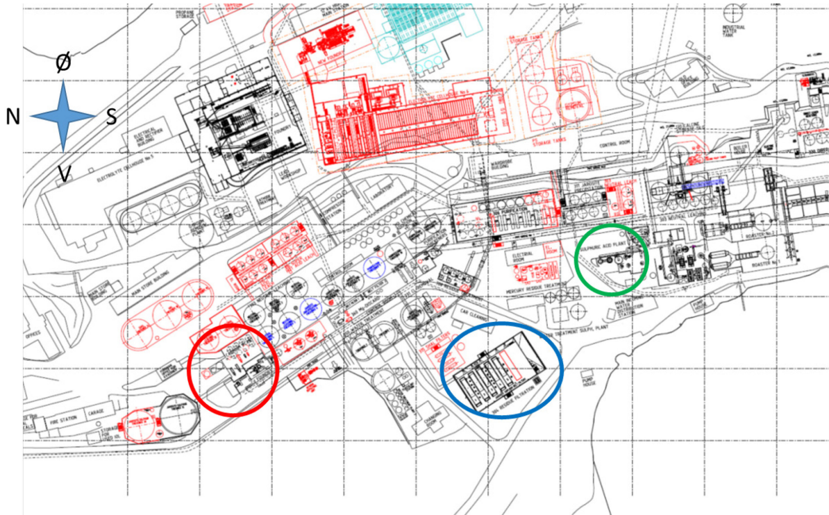
Figur 4-1 Figuren angir hvor utslippene er lokalisert i spredningsberegningene med CONDEP. Blå sirkel: Utslipp til luft av kadmium fra filterstasjon. Øvrige kadmiumutslipp fra lutningsprosessen er også forenklet allokert her. Rød sirkel: Utslipp av kadmium fra Cd støperi. Grønn sirkel: SO 2 -utslipp fra svovelsyrefabrikk.
