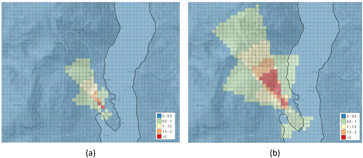
Figur 5-4 Årsmiddel konsentrasjonsfelt \text{SO}_2 ( \mu\text{g}/\text{m}^3 ) beregnet med CONDEP for (a) dagens produksjon og (b) samlet med utvidet produksjon. Merk at CONDEP ikke tar høyde for topografi og at vindfeltet er antatt uniformt. Det vil derfor naturlig være noe avbøyning mot nord i terrenget.
