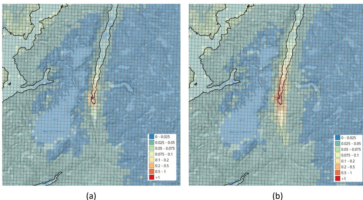
Figur 5-5 WRF-EMEP beregnet årsmiddel konsentrasjon (2015) for SO_2 ( \mu g/m^3 ) ved (a) dagens produksjon og (b) samlet med utvidet produksjon.
