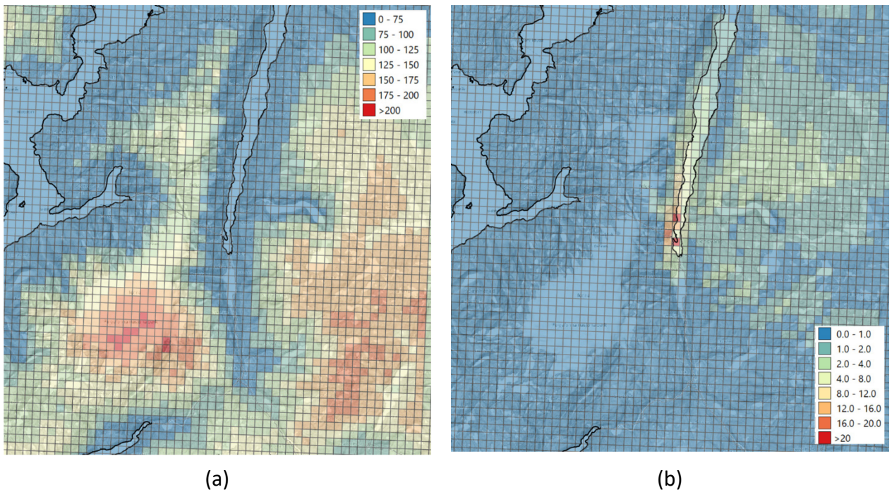
Figur 5-7 WRF-EMEP beregnet total våtavsetning av svovel [ \text{mgS}/\text{m}^2\text{år} ] ved (a) dagens produksjon (b) som differanse ved utvidet produksjon. Merk forskjellen i fargeskala mellom figurene hvor alle konturer i (b) faller innunder den første konturen i (a)
