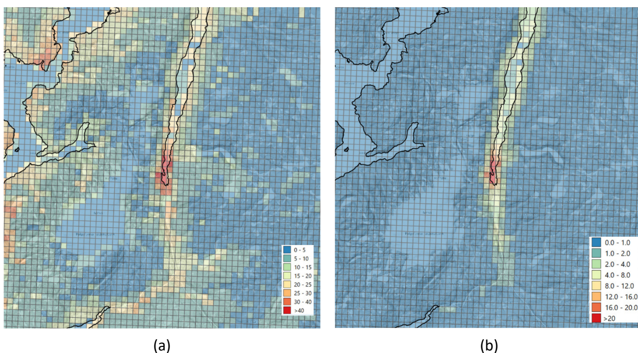
Figur 5-8 WRF-EMEP beregnet total tørravsetning av svovel [ \text{mgS}/\text{m}^2\text{år} ] ved (a) dagens produksjon (b) som differanse ved utvidet produksjon.
