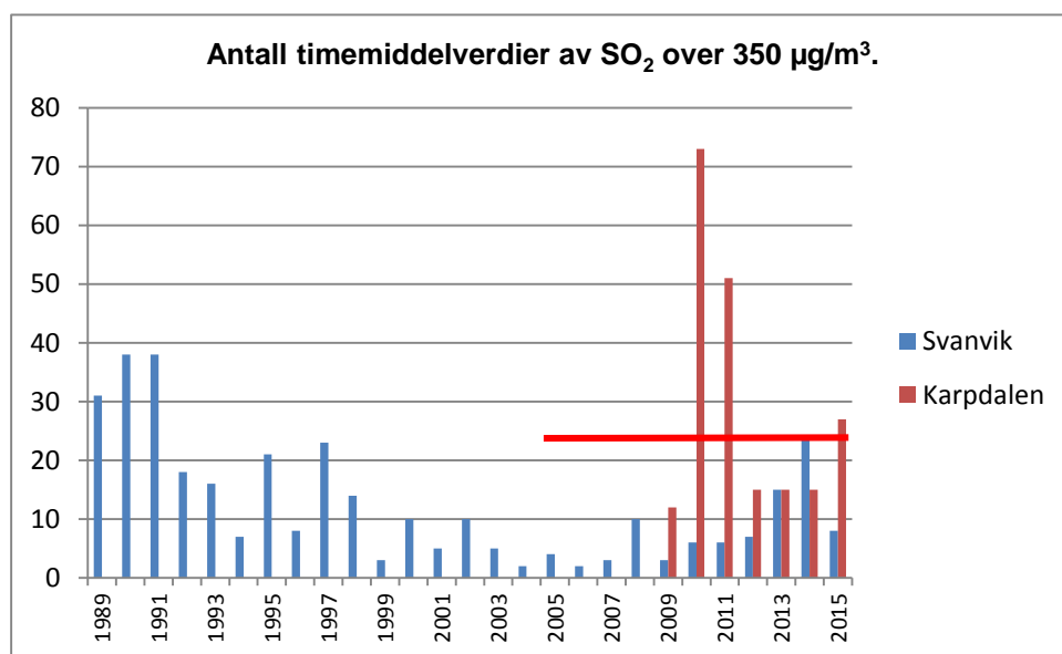
Figur 16: Antall timemiddelverdier av SO 2 over grenseverdien på 350 µg/m 3 på Svanvik (1989-2015) og i Karpdalen (2009-2015). Norsk lovverk tillater 24 overskridelser per kalenderår (gjeldende fra 2005, markert med rød linje).
