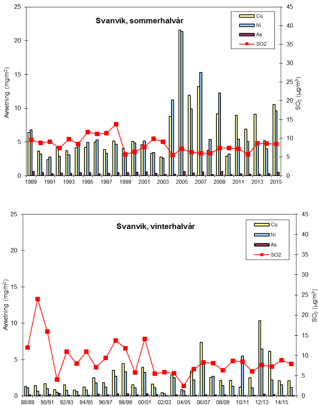
Figur 21: Avsetning med nedbør av Cu, Ni og As (mg/m 2 ) i sommerhalvårene fra 1989 til 2015 og i vinterhalvårene fra 1988/89 til 2015/16. Halvårsmiddelkonsentrasjonene av SO 2 er også vist (µg/m 3 ).
