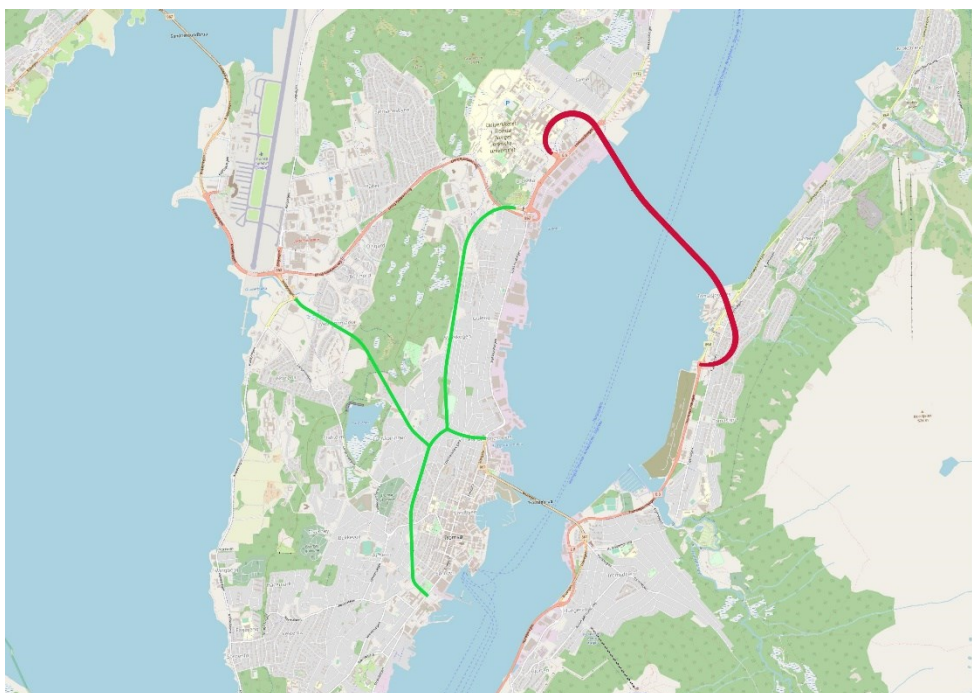
Figur 3-7: Sentrumstangenten med kobling mot Breivikatunnelen (grønn) er et toveis tunellsystem, mens Tromsøysundtunnelen (rød) er en enveis tunnel.
