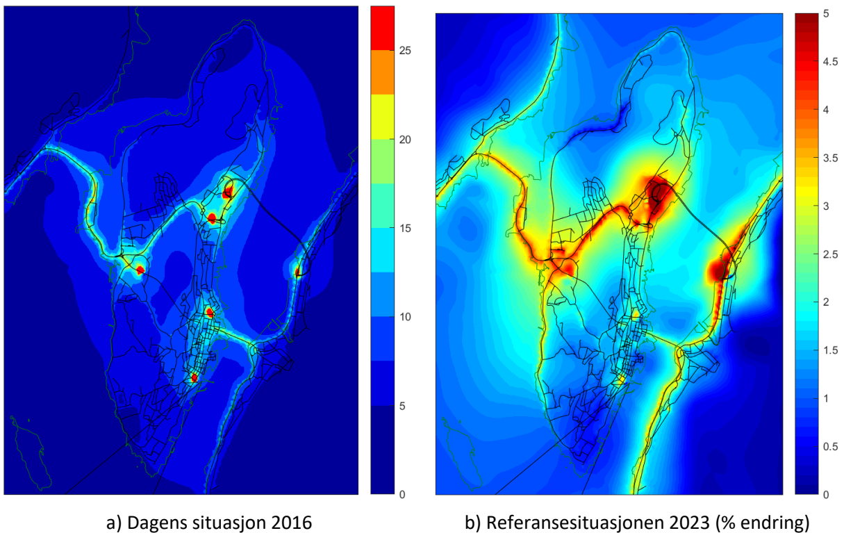
Figur S 2: Beregnet årsmiddelkonsentrasjon for PM_{10} for et utsnitt av modellområdet for a) Dagens situasjon 2016 og b) Referansesituasjonen 2023, vist som prosentvis endring fra 2016. Grenseverdien for årsmiddelverdi er på 25 \mu\text{g}/\text{m}^3 (markert som overgangen til rødt), mens regjeringens nasjonale mål og helsemyndighetenes anbefaling for årsmiddel er på 20 \mu\text{g}/\text{m}^3
