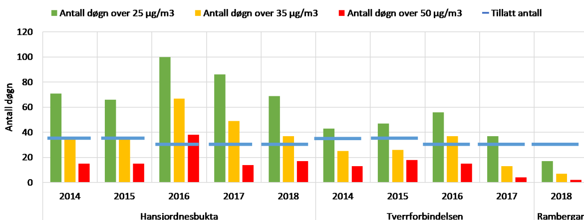
Figur 2-7: Antall døgn pr år med målt konsentrasjon av PM 10 over nedre vurderingsterskel på 25 µg/m 3 , over øvre vurderingsterskel på 35 µg/m 3 og over grenseverdien på 50 µg/m 3 , på målestasjoner i Tromsø i årene 2014-2018. Antall tillatte overskridelser av grenseveriden for døgnmiddel var 35 i 2014 og 2015 og 30 fra og med 2016.
