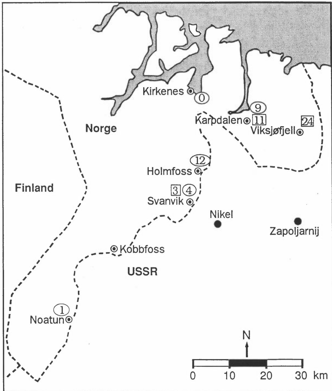
Figur 8: Antall døgnmiddelverdier av SO 2 over 100 µg/m 3 i perioden oktober 1990-mars 1991 målt med kontinuerlig registrerende prøvetakere □ og døgnprøvetakere ○.
