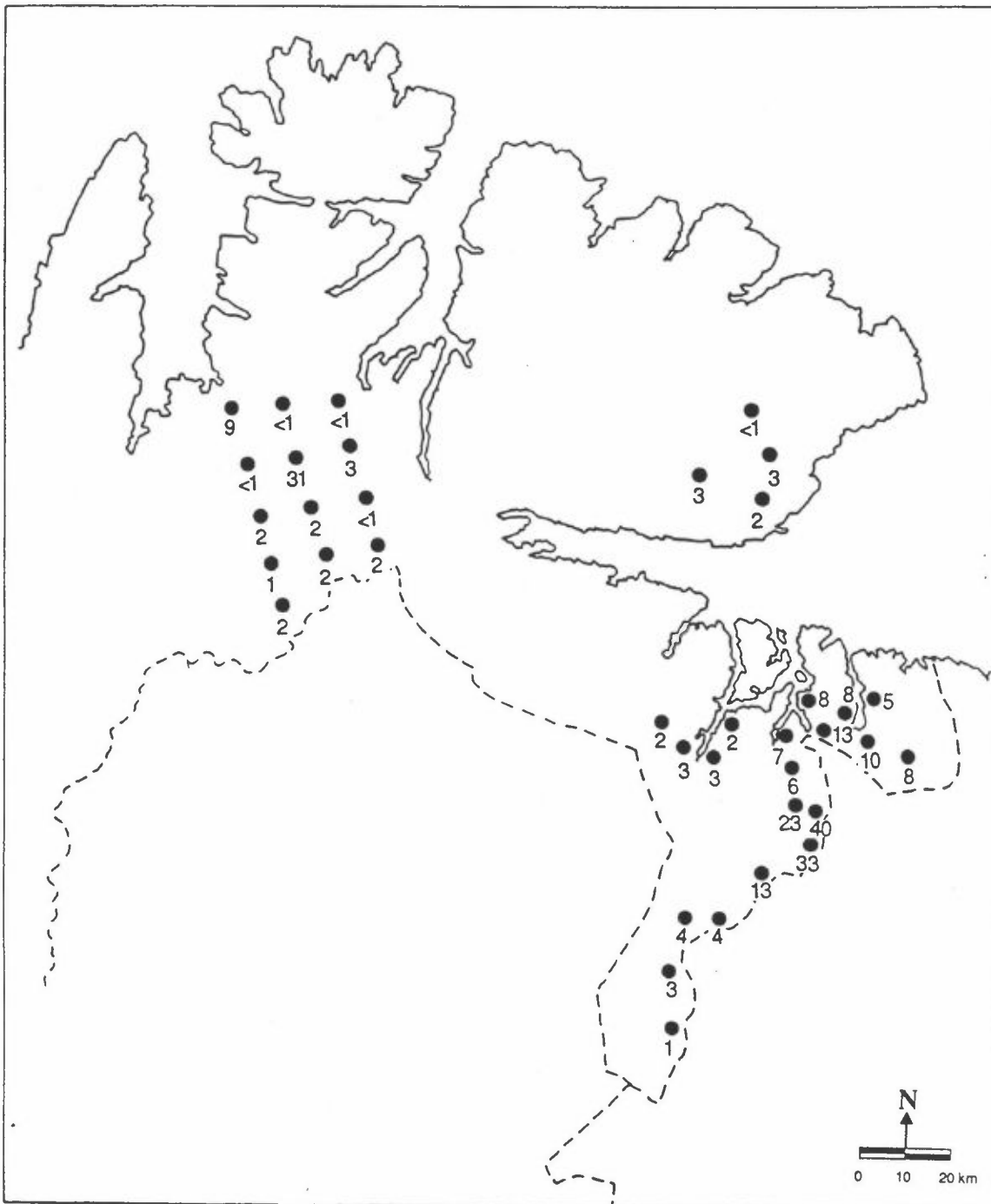
Figur 34: Konsentrasjoner av Cu i snøprøver fra Øst-Finnmark, mars/april 1991 (µg/l).
