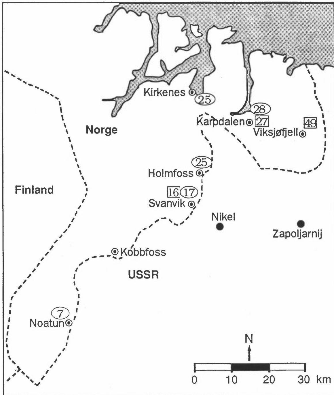
Figur 5: Middelerdier av \text{SO}_2 i perioden oktober 1990-mars 1991 målt med kontinuerlig registrerende prøvetakere □ og døgnprøvetakere ○ ( \mu\text{g}/\text{m}^3 ).
