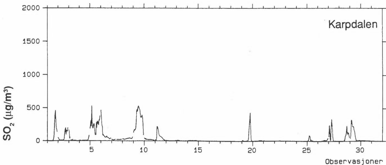
Figur 15: Timemiddelkonsentrasjoner av \text{SO}_2 i januar 1991 i Svanvik, Karpdalen og på Viksjøfjell ( \mu\text{g}/\text{m}^3 ).
