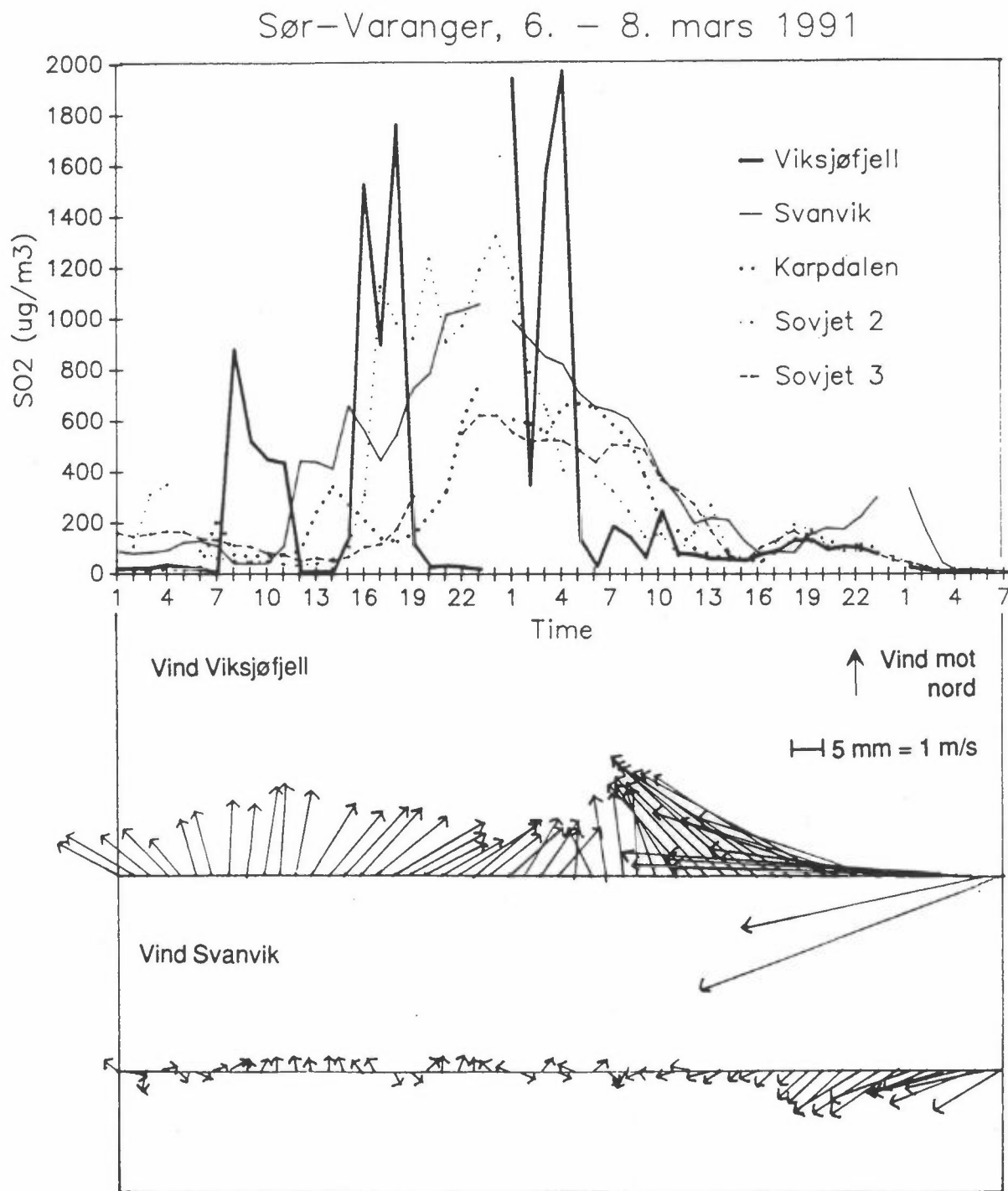
Figur 7: Middelkonsentrasjoner av SO 2 , vindretning og vindstyrke 6.-8. mars 1991.
