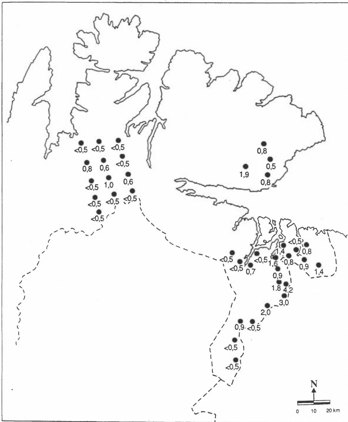
Figur 33: Konsentrasjoner av As i snøprøver fra Øst-Finnmark, mars/april 1991 ( \mu\text{g/l} ).
