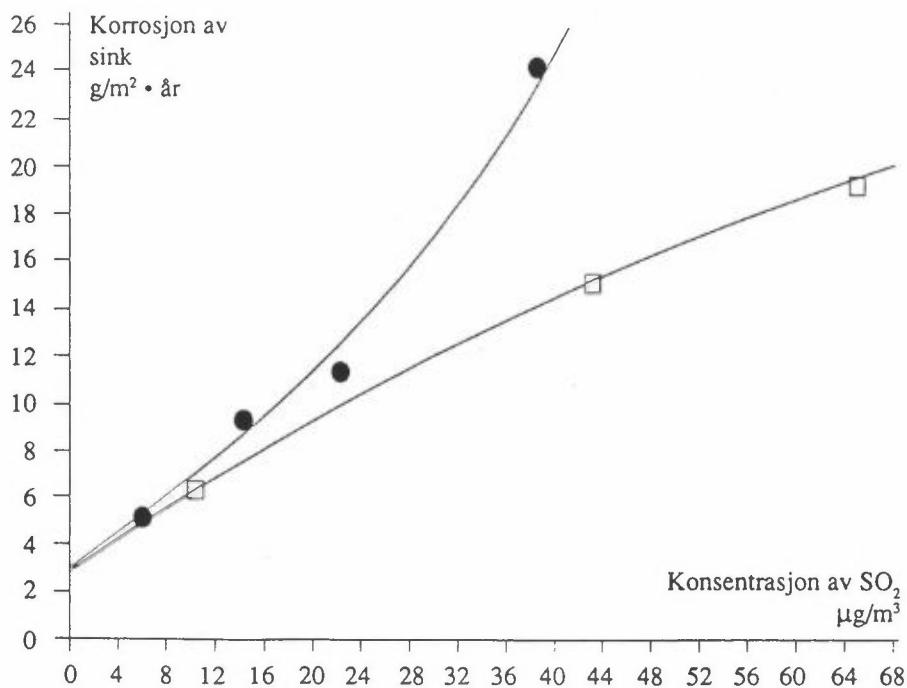
Figur 37: Årskorrosjon for sink som funksjon av SO 2 -konsentrasjonen (g/m 2 · a).
