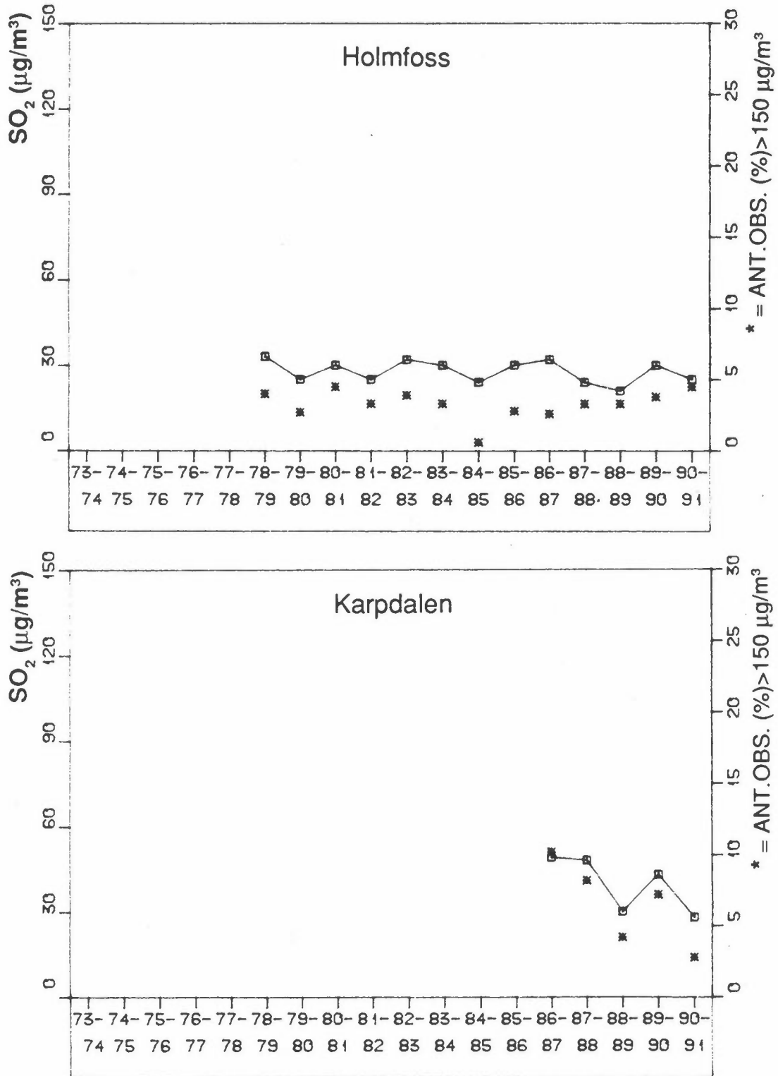
Figur 11: Vintermiddelkonsentrasjoner av SO 2 (µg/m 3 ) og frekvens av døgnmiddelverdier over 150 µg/m 3 i Holmfoss og Karpdalen.
