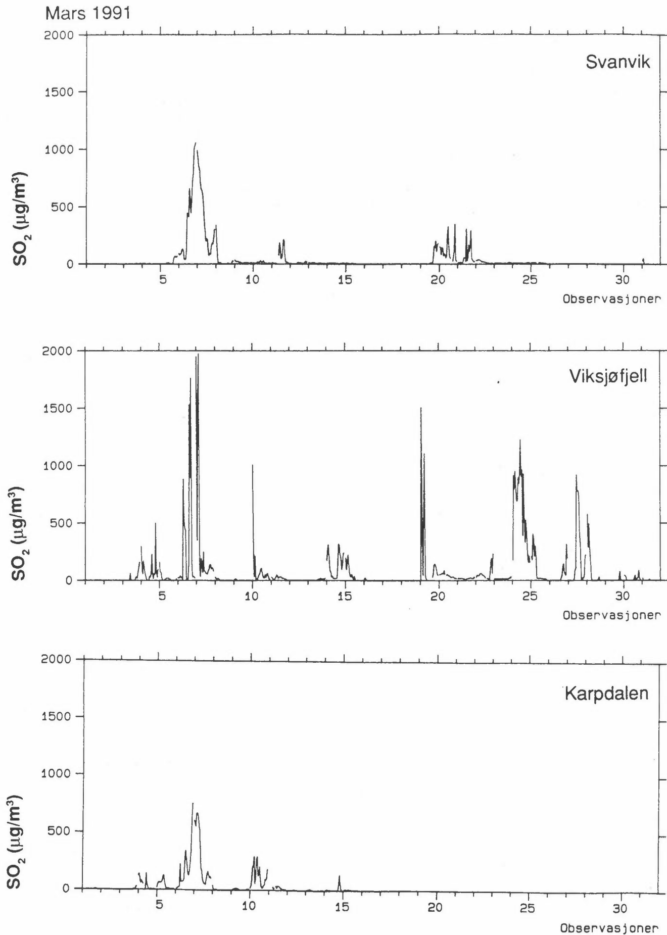
Figur 17: Timemiddelkonsentrasjoner av SO 2 i mars 1991 i Svanvik, Karpdalen og på Viksjøfjell (µg/m 3 ).
