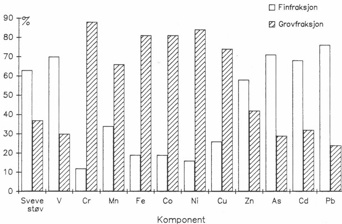
Figur 25: Andel av konsentrasjoner av metaller i to størrelsesfraksjoner av svevestøvparkler på Viksjøfjell i januar 1990-mars 1991.
