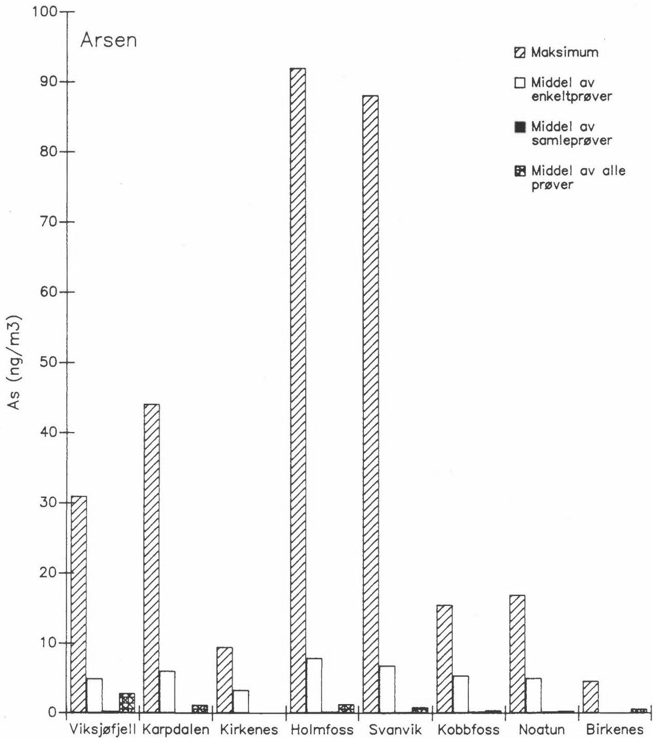
Figur 24: Middell- og maksimumsverdier av As i svevestøv (ng/m 3 ) i perioden januar 1990-mars 1991. (Kobbfoss ble nedlagt 1.10.1990, og målingene på Birkenes gjelder februar 1985-januar 1986).
