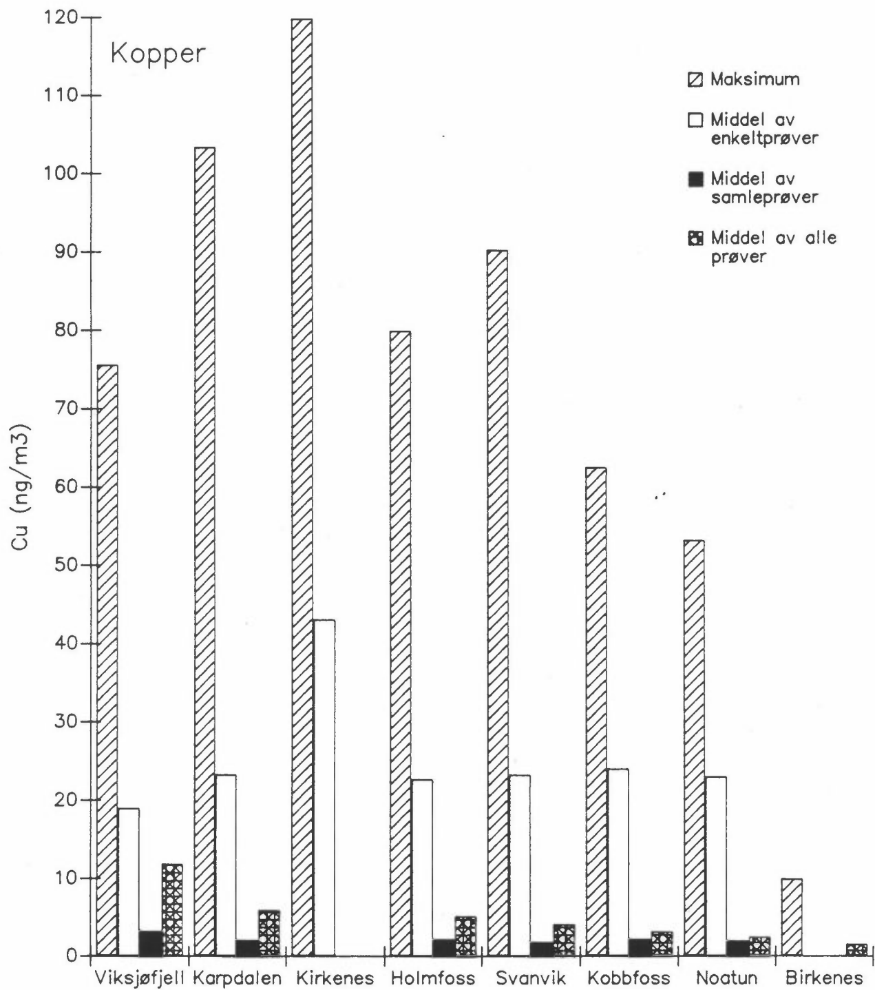
Figur 23: Middelt- og maksimumsverdier av Cu i svevestøv (ng/m 3 ) i perioden januar 1990-mars 1991. (Kobbfoss ble nedlagt 1.10.1990, og målingene på Birkenes gjelder februar 1985-januar 1986).
