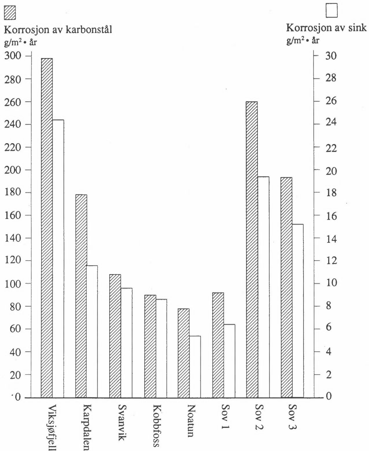
Figur 35: Årskorrosjon av karbonstål og sink på alle prøvesteder (g/m 2 · a).
