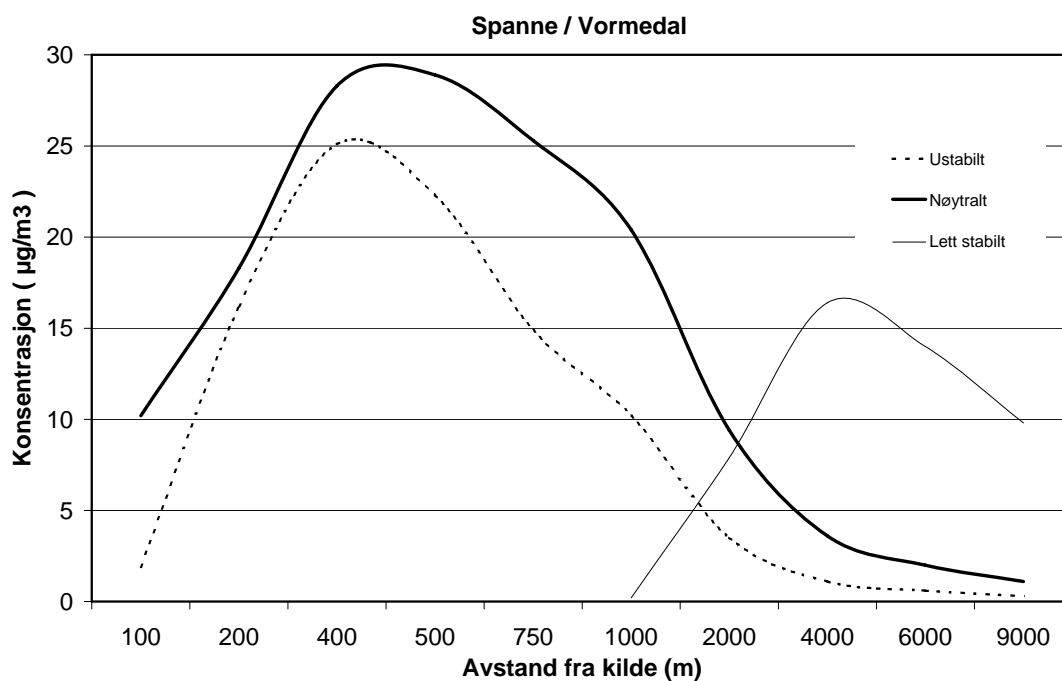
Figur 2: \text{NO}_2 -bidrag til bakkekonsentrasjon. 150 \text{ mg NO}_2/\text{m}^3 , 60\,000 \text{ Nm}^3/\text{h} .
