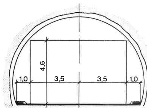
Tunnelprofil T9
