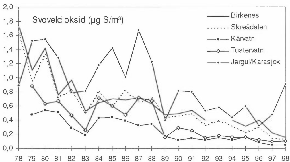
Figur 3.4: Årsmiddelkonsentrasjoner av svoveldioksid i luft på norske bakgrunnsstasjoner i 1978–1998.
