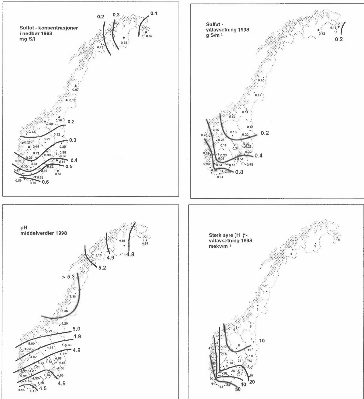
Figur 1.1: Middelskonsentrasjoner i nedbør og våtavsetning av sulfat (sjøsaltkorrigert) og sterk syre (pH) på norske bakgrunnsstasjoner i 1998.
