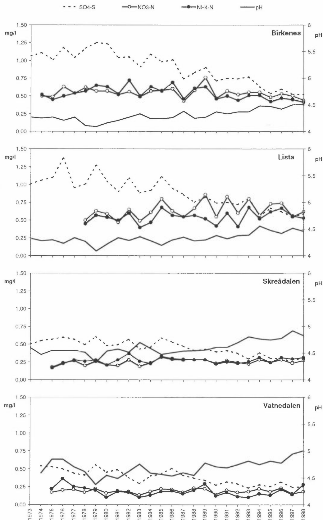
Figur 1.4: Veide årsmiddelkonsentrasjoner av sulfat (sjøsaltkorrigert), nitrat, ammonium og pH-middelverdier i nedbør på norske bakgrunnsstasjoner, 1973-1998.
