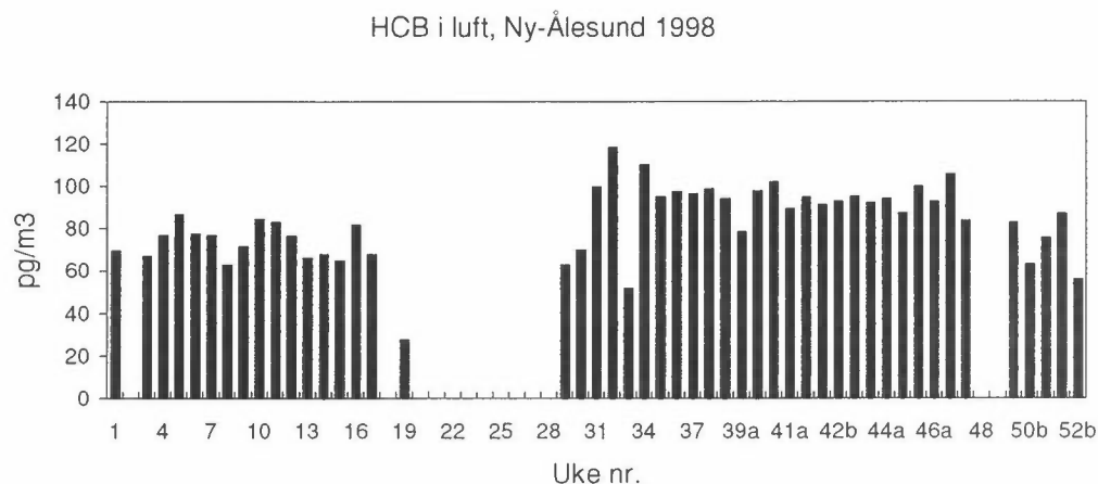
Figur 5.8: Ukentlig luftkonsentrasjon av HCB i Ny-Ålesund i 1998. I en del tilfeller ble flere målinger gjort i løpet av en uke. I slike tilfeller ble prøvene nummerert med ukenummer og en bokstav, f.eks. 39a og 39b.
