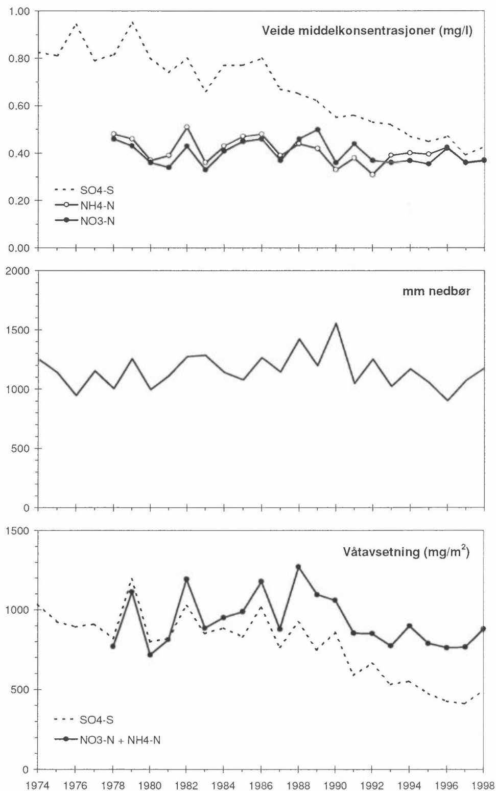
Figur 1.5: Veide årsmiddelkonsentrasjoner av sulfat (sjøsaltkorrigert), nitrat og ammonium, gjennomsnittlige årlige nedbørmengder og våtavsetninger av sulfat og sum (nitrat+ammonium) 1974-1998 for 7 representative stasjoner på Sørlandet og Østlandet: Birkenes, Lista, Skreådalen, Vatnedalen, Treungen, Gulsvik/Brekkebygda og Løken.
