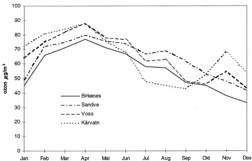
Figur 4.3: Månedsmiddeler av ozon 1997 ( \mu\text{g}/\text{m}^3 ) for Birkenes, Sandve, Voss og Kårvatn.
