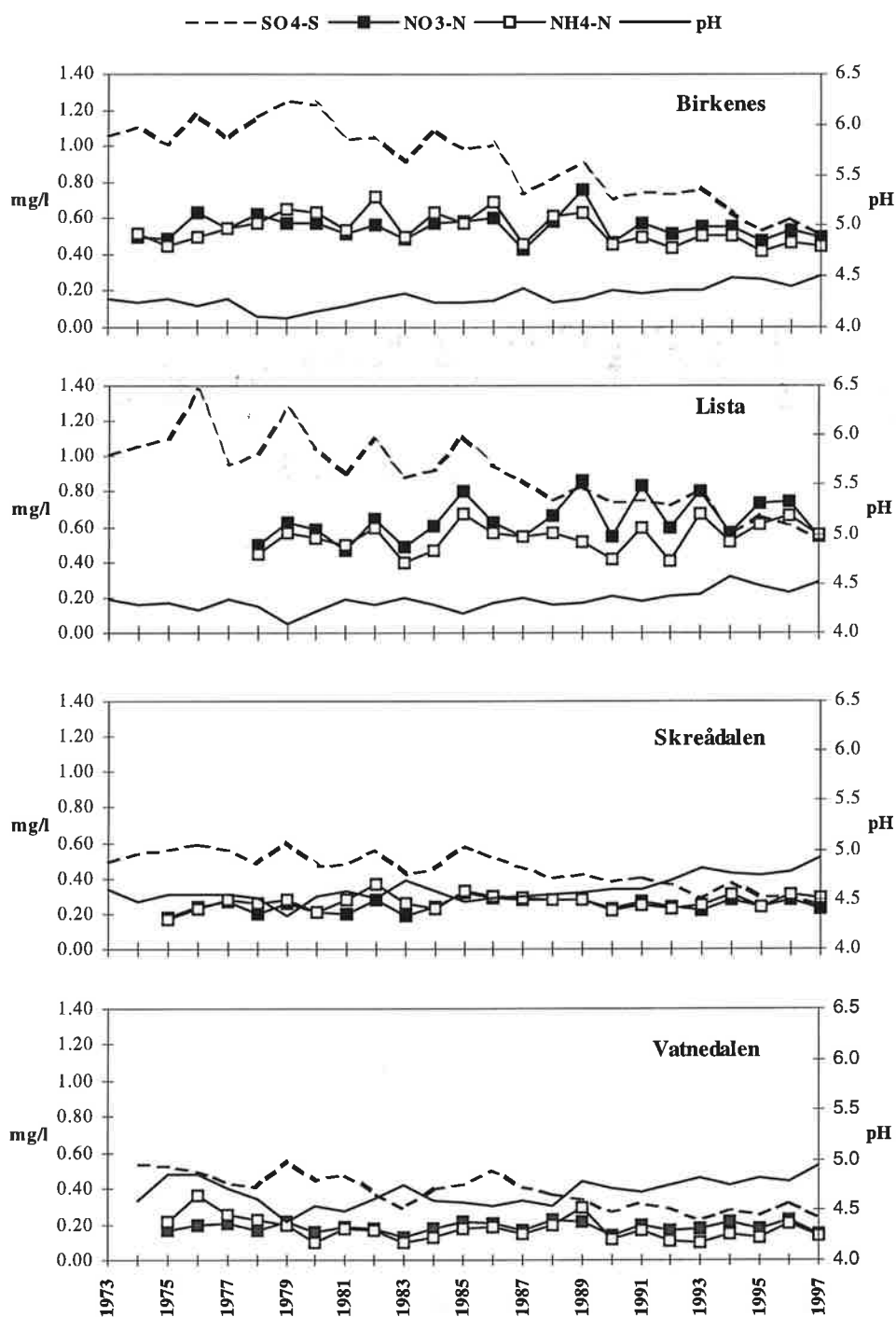
Figur 1.4: Veide årsmiddelkonsentrasjoner av sulfat (sjøsaltkorrigeret), nitrat, ammonium og pH-middelverdier i nedbør på norske bakgrunnsstasjoner, 1973-1997.
