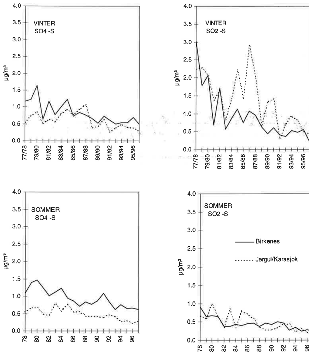
Figur 3.5: Middelkonsentrasjoner av partikulært sulfat og svoveldioksid i luft for vinterhalvårene 1978/1979-1996/1997 (oktober-mars) og sommerhalvårene 1978-1997 på Birkenes og Jergul/Karasjok.
