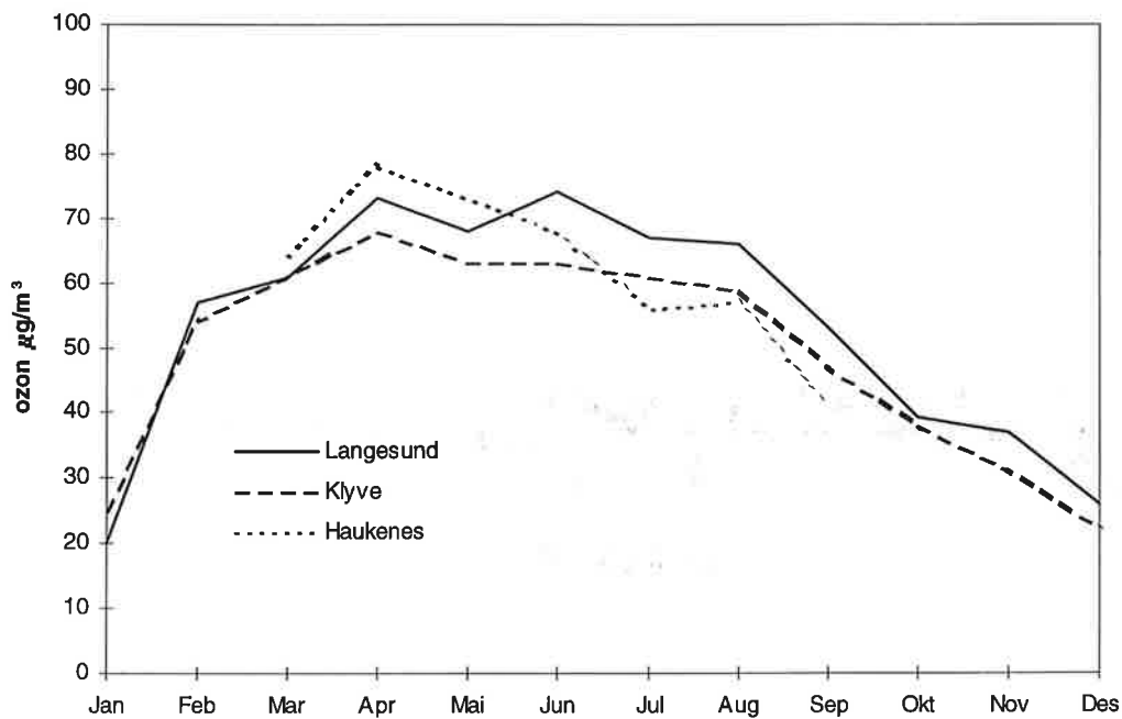
Figur 4.2: Månedsmiddeler av ozon 1997 ( \mu\text{g}/\text{m}^3 ) for Langesund, Klyve og Haukenes.
