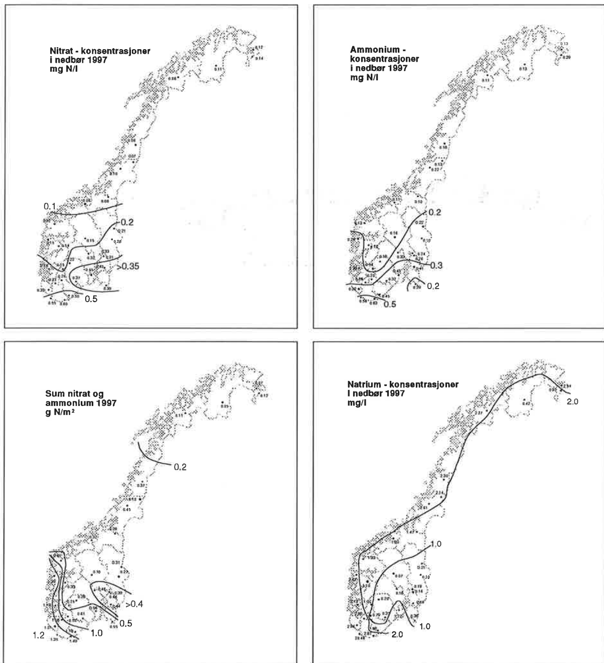
Figur 1.2: Middelkonsentrasjoner i nedbør av nitrat, ammonium og natrium, og våtavsetning av total nitrogen (nitrat + ammonium) på norske bakgrunnsstasjoner i 1997.
