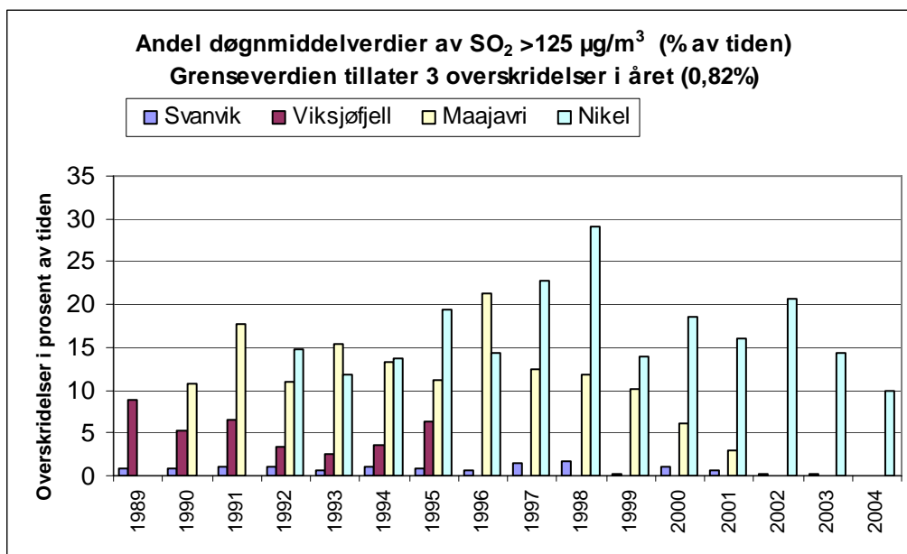
Figur 11: Andel av tiden grenseverdien for døgnmiddel av SO 2 på 125 µg/m 3 er overskredet i Svanvik (1989-2004), på Viksjøfjell (1989-1995, i Maajavri (1990-2001) og i Nikel (1992-2004) (3 tillatte overskridelser i året tilsvarer 0,82% av tiden).
