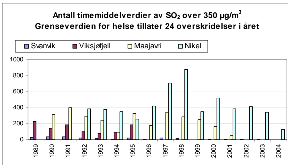
Figur 15: Antall timemiddelverdier av SO 2 over grenseverdien på 350 µg/m 3 i Svanvik (1989-2004), på Viksjøfjell (1989-1995), i Maajavri (1990-2001) og i Nikel (1992-2004) (24 tillatte overskridelser i året).
