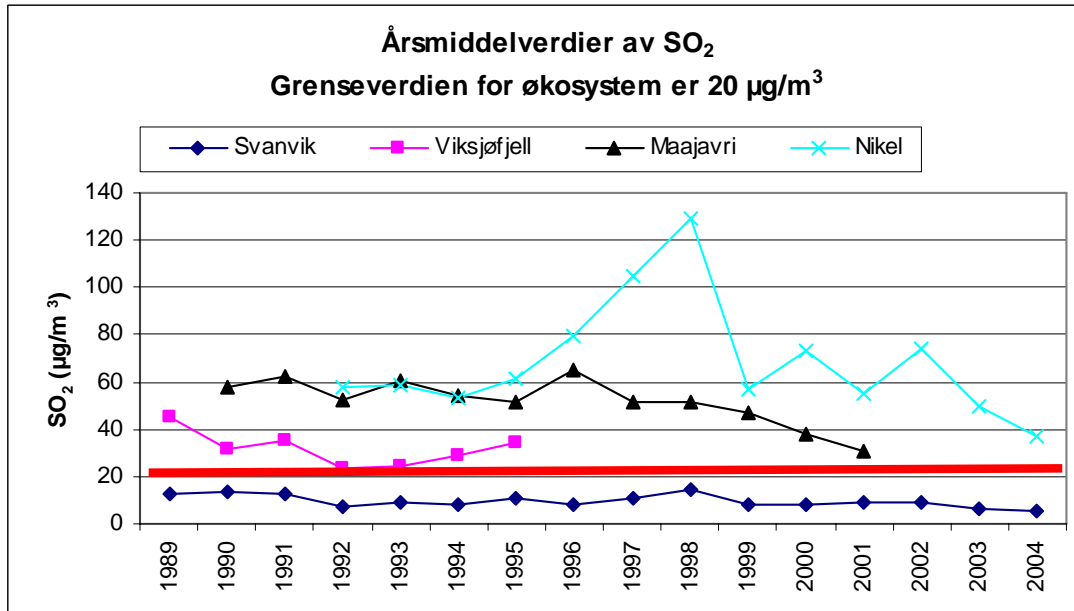
Figur 6: Årsmiddelverdier av SO 2 i Svanvik (1989-2004), på Viksjøfjell (1989-1995), i Maajavri (1990-2001) og i Nikel (1992-2004) (µg/m 3 ).
