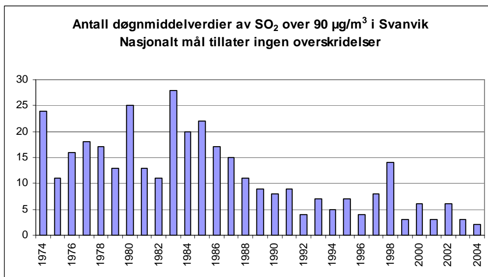
Figur 12: Antall døgnmiddelverdier av SO 2 over Nasjonalt mål på 90 µg/m 3 i Svanvik i årene 1974-2004 (ingen tillatte overskridelser).
