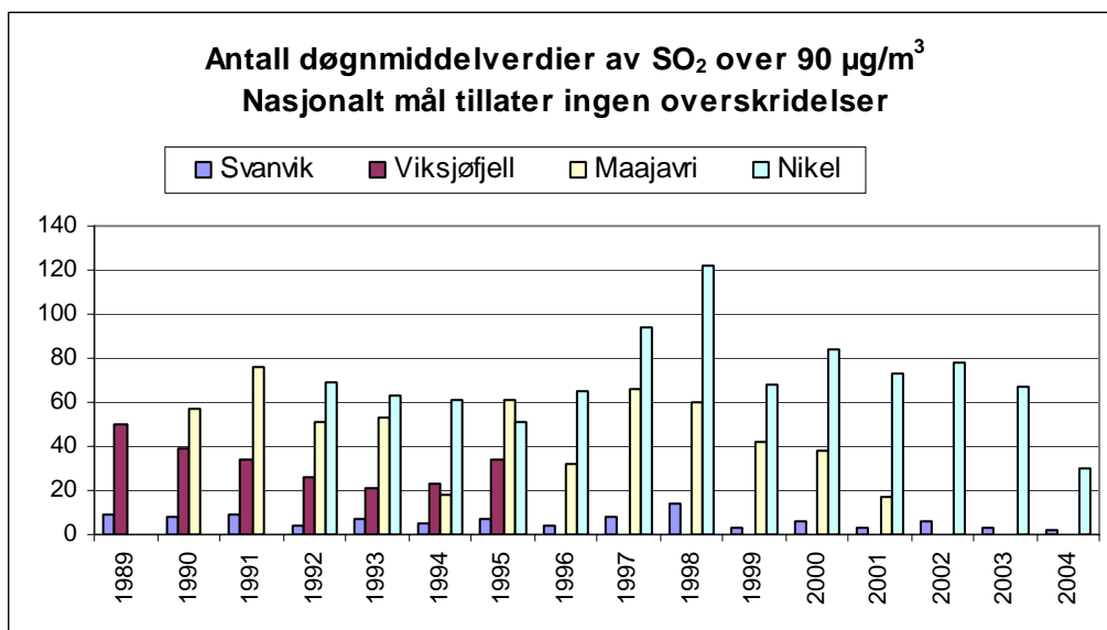
Figur 13: Antall døgnmiddelverdier av SO 2 over Nasjonalt mål på 90 µg/m 3 i Svanvik (1989-2004), på Viksjøfjell (1989-1995), i Maajavri (1990-2001) og i Nikel (1992-2004) (ingen tillatte overskridelser).
