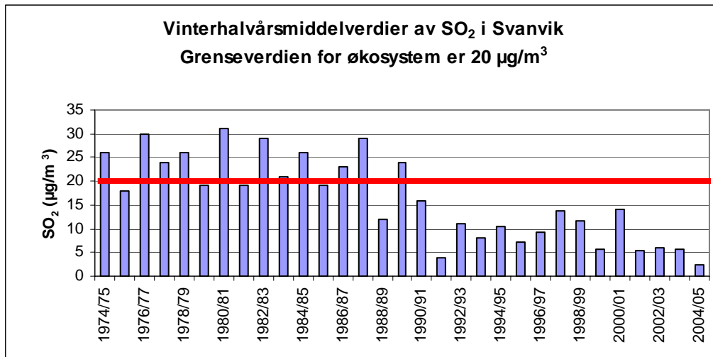
Figur 7: Vinterhalvårsmiddelverdier av SO 2 i Svanvik 1974/75 – 2004/05 (µg/m 3 ).
