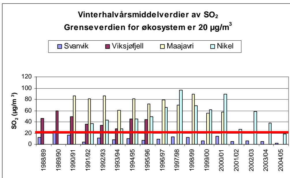
Figur 8: Vinterhalvårsmiddelverdier av SO 2 i Svanvik (1988/99-2004/05), på Viksjøfjell (1988/89-1995/96), i Maajavri (1990/91-2000/01) og i Nikel (1991/92-2004/05) (µg/m 3 ).
