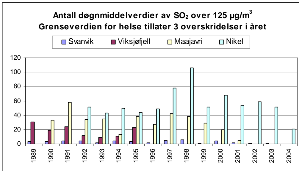
Figur 10: Antall døgnmiddelverdier av SO 2 over grenseverdien på 125 µg/m 3 i Svanvik (1989-2004), på Viksjøfjell (1989-1995), i Maajavri (1990-2001) og i Nikel (1992-2004) (3 tillatte overskridelser i året).
