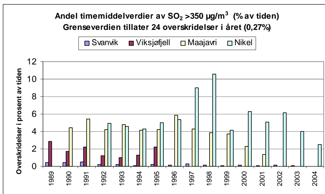
Figur 16: Andel av tiden grenseverdien for timemiddel av SO 2 på 350 µg/m 3 er overskredet i Svanvik (1989-2004), på Viksjøfjell (1989-1995), i Maajavri (1990-2001) og i Nikel (1992-2004) (24 tillatte overskridelser i året tilsvarer 0,27% av tiden).
