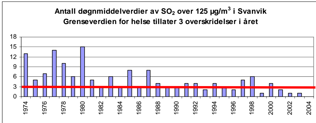
Figur 9: Antall døgnmiddelverdier av SO 2 over grenseverdien på 125 µg/m 3 i Svanvik i årene 1974-2004 (3 tillatte overskridelser i året).
