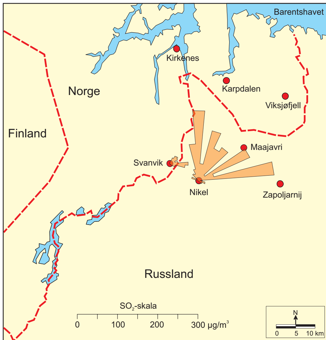
Figur 4: Middelskonsentrasjoner av SO 2 i Svanvik og Nikel i perioden oktober 2004-mars 2005 (µg/m 3 ). Figuren viser middelskonsentrasjoner av SO 2 for hver av 36 10°-vindsektorer. Svanvik er belastet fra Nikel og Zapoljarnij (mest fra Nikel).
