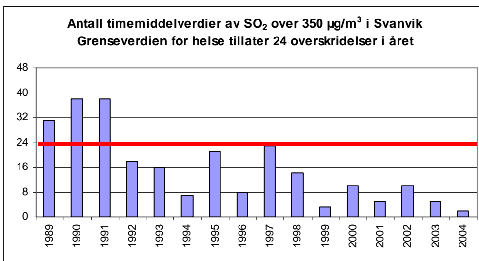
Figur 14: Antall timemiddelverdier av SO 2 over grenseverdien på 350 µg/m 3 i Svanvik i årene 1989-2004 (24 tillatte overskridelser i året).
