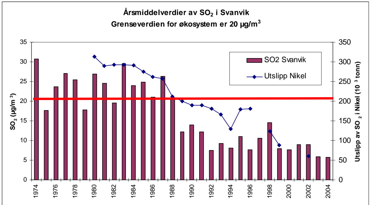
Figur 5: Årsmiddelverdier av SO 2 i Svanvik i årene 1974-2004 (µg/m 3 ).
