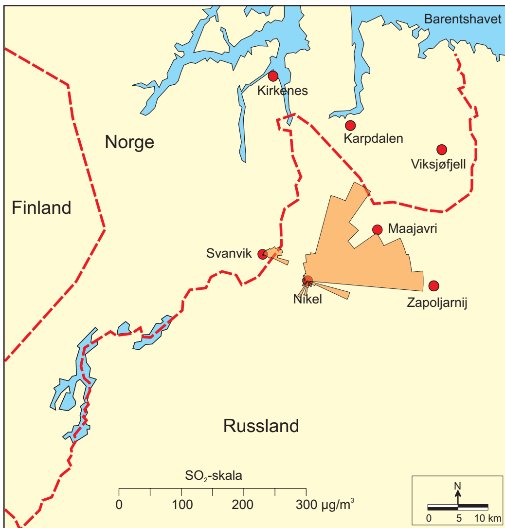
Figur 3: Middelkonsentrasjoner av \text{SO}_2 i Svanvik og Nikel i perioden april-september 2004 ( \mu\text{g}/\text{m}^3 ). Figuren viser middelkonsentrasjoner av \text{SO}_2 for hver av 36\ 10^\circ -vindsektorer. Svanvik er belastet fra Nikel og Zapoljarnij (mest fra Nikel).
