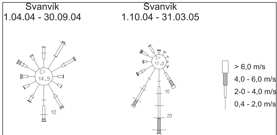
Figur 2: Vindroser fra Svanvik for periodene april-september 2004 og oktober 2004-mars 2005. (Vindrosene viser frekvensen av vind i tolv 30-graders sektorer, dvs. hvor ofte det blåser fra disse retningene).
