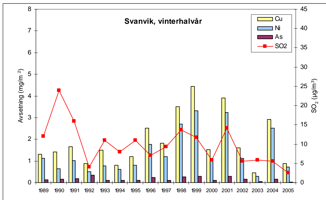
Figur 17: Avsetning med nedbør av Cu, Ni og As (mg/m 2 ) i sommerhalvårene fra 1989 til 2004 og i vinterhalvårene fra 1988/89 til 2004/05. Halvårsmiddelkonsentrasjonene av SO 2 er også vist (µg/m 3 ).
