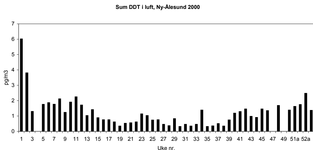
Figur 5.10: Ukentlig luftkonsentrasjon av "sum DDT" (sum o,p' -DDE, p,p' -DDE, o,p' -DDD, p,p' -DDD, o,p' -DDT og p,p' -DDT) i Ny-Ålesund i 2000. I en del tilfeller ble flere målinger gjort i løpet av en uke. I slike tilfeller ble prøvene nummerert med ukenummer og en bokstav, f.eks. 51a og 51b.
