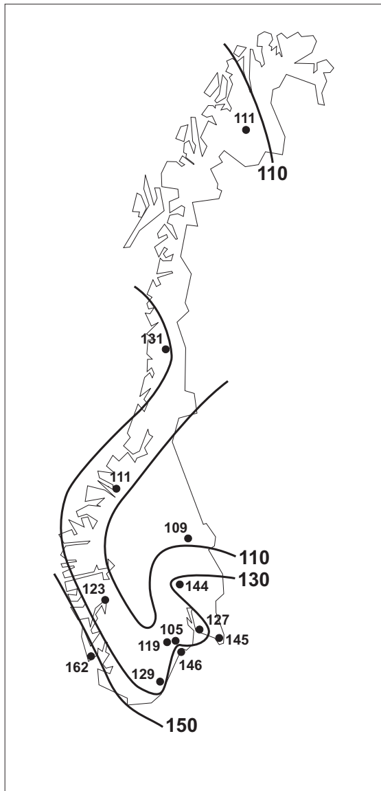
Figur 4.10: Antall døgn med 8-timers middelveirdier av ozon over 60 \mu\text{g}/\text{m}^3 , april-september 2000.
