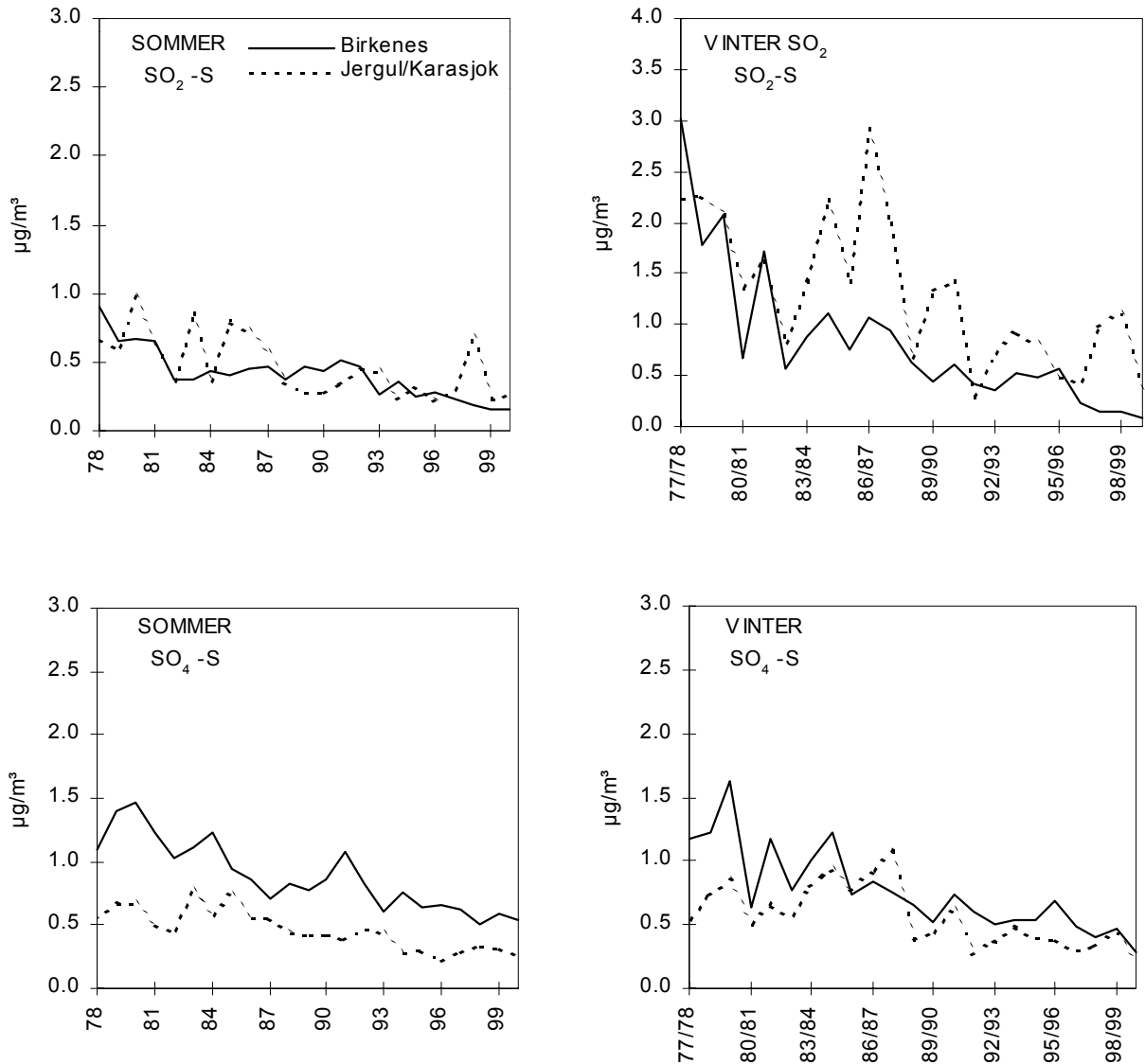
Figur 3.8: Middelskonsentrasjoner av partikulært sulfat og svoveldioksid i luft for vinterhalvårene 1978/1979 - 1999/2000 (oktober-mars) og sommerhalvårene 1978-2000 på Birkenes og Jergul/Karasjok.
