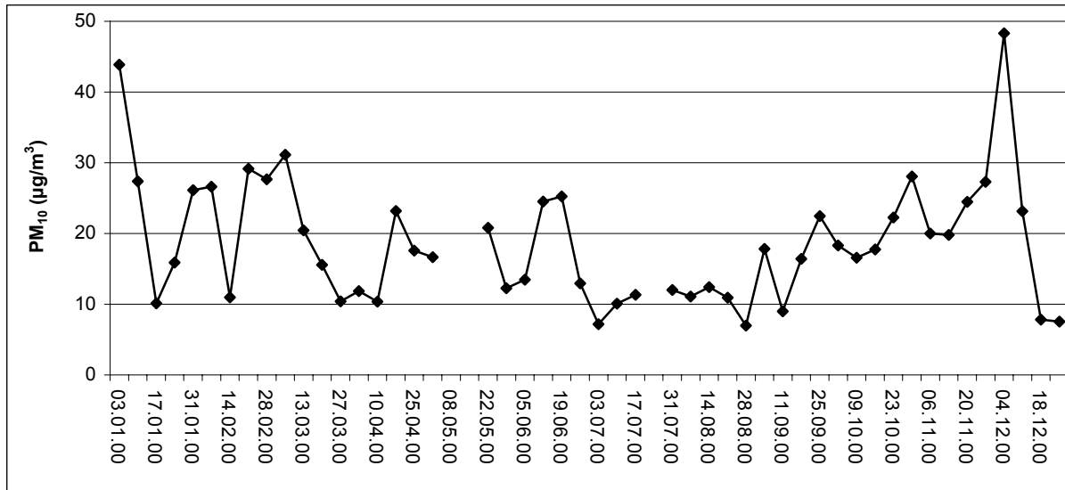
Figur 6.6: Konsentrasjon av PM 10 basert på ukkesmidler for Lista målt i tidsrommet 03.01.00–31.12.00. For periodene 08.05.00–22.05.00 og 24.07.00–31.07.00 eksisterer det ikke målinger.
