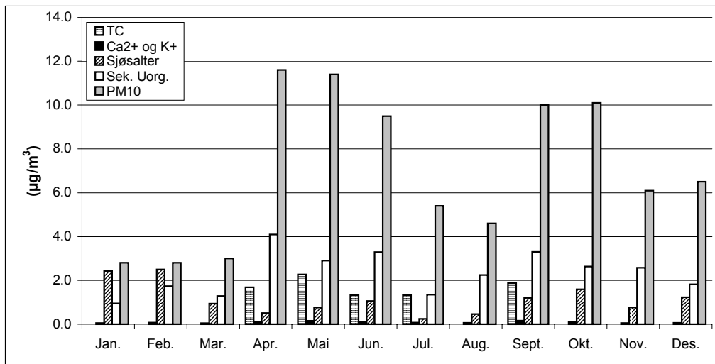
Figur 6.5: Konsentrasjon og kjemisk spesiering av PM_{10} -fraksjonen for perioden 01.01.00–31.12.00 på Birkenes. Negative og manglende verdier for PM_{10} og korresponderende verdier for de kjemiske forbindelsene er ikke inkludert.
