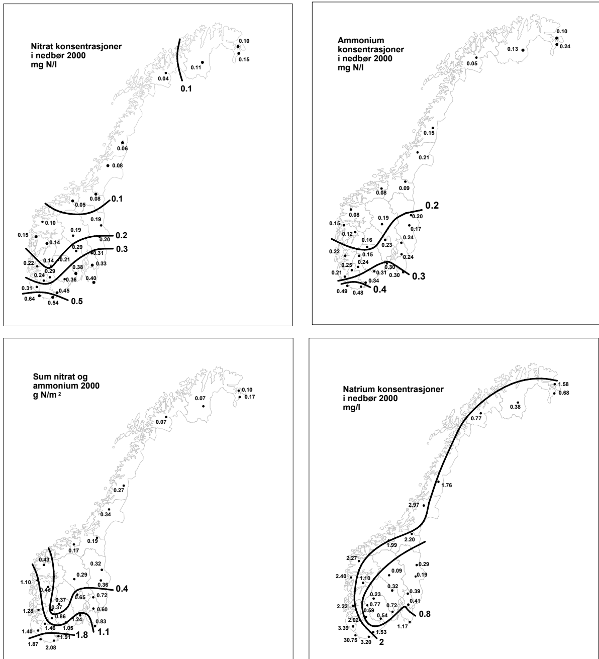
Figur 1.2: Middelskonsentrasjoner i nedbør av nitrat, ammonium og natrium, og våtavsetning av total nitrogen (nitrat + ammonium) på norske bakgrunnsstasjoner i 2000.
