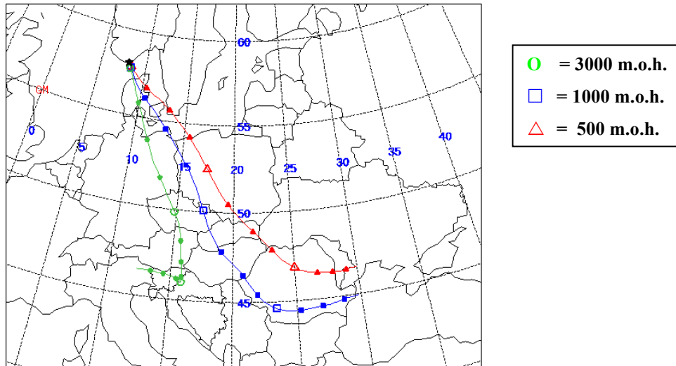
Figur 6.2: 72 timers tilbaketrajektorier for 30.04.00 (Birkenes). Konsentrasjon av PM_{10} = 28,1 \mu\text{g}/\text{m}^3 .
