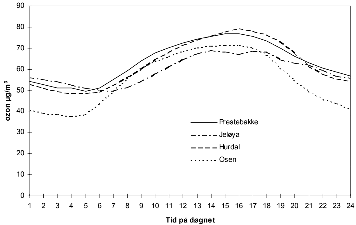
Figur 4.5: Midlere døgnvariasjon av ozon ( \mu\text{g}/\text{m}^3 ) for Prestebakke, Jeløya, Hurdal og Osen, april-september 2000.
