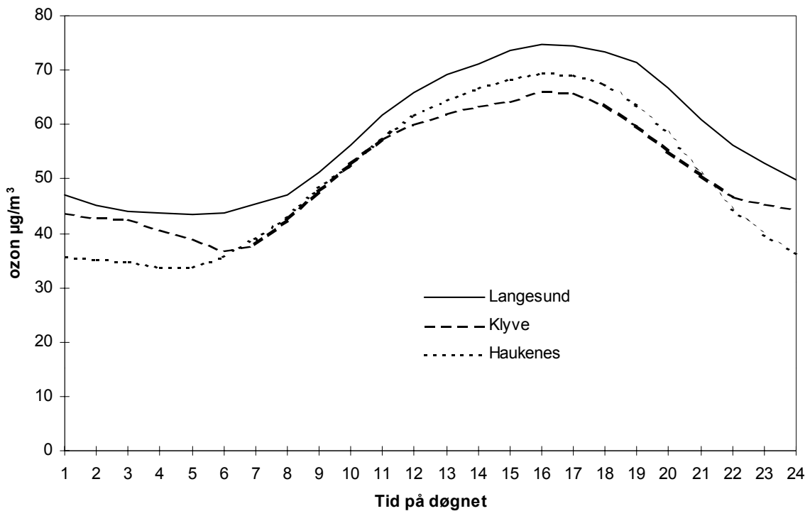
Figur 4.6: Midlere døgnvariasjon av ozon ( \mu\text{g}/\text{m}^3 ) for Langesund, Klyve og Haukenes, april-september 2000.
