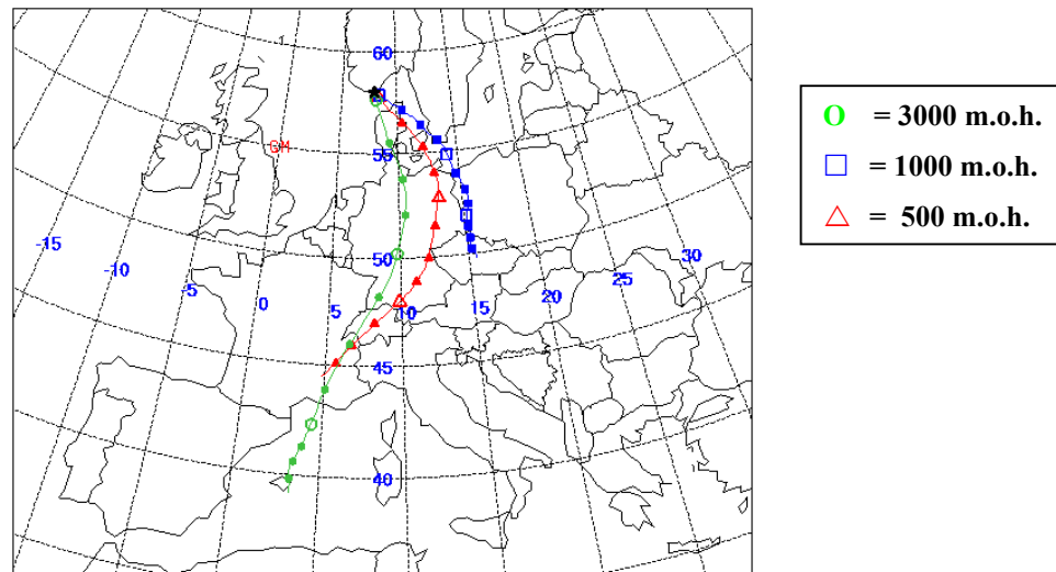
Figur 6.3: 72 timers tilbaketrajektorier for 30.09.00 (Birkenes). Konsentrasjon av PM_{10} = 32,6 \mu\text{g}/\text{m}^3 .
