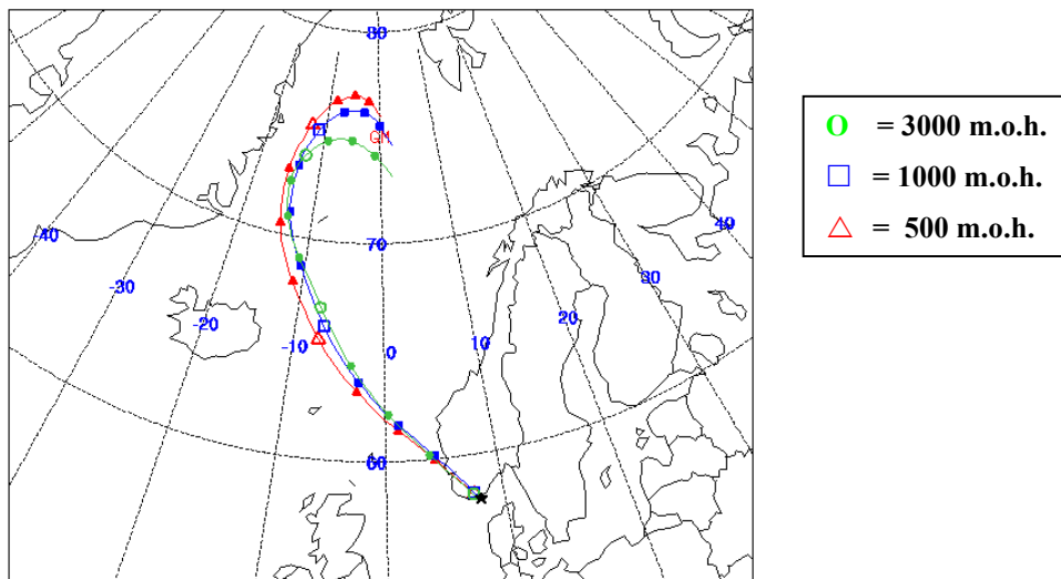
Figur 6.4: 72 timers tilbaketrajektorier for 08.08.00 (Birkenes). Konsentrasjon av PM_{10} = 2,6 \mu\text{g}/\text{m}^3 .
