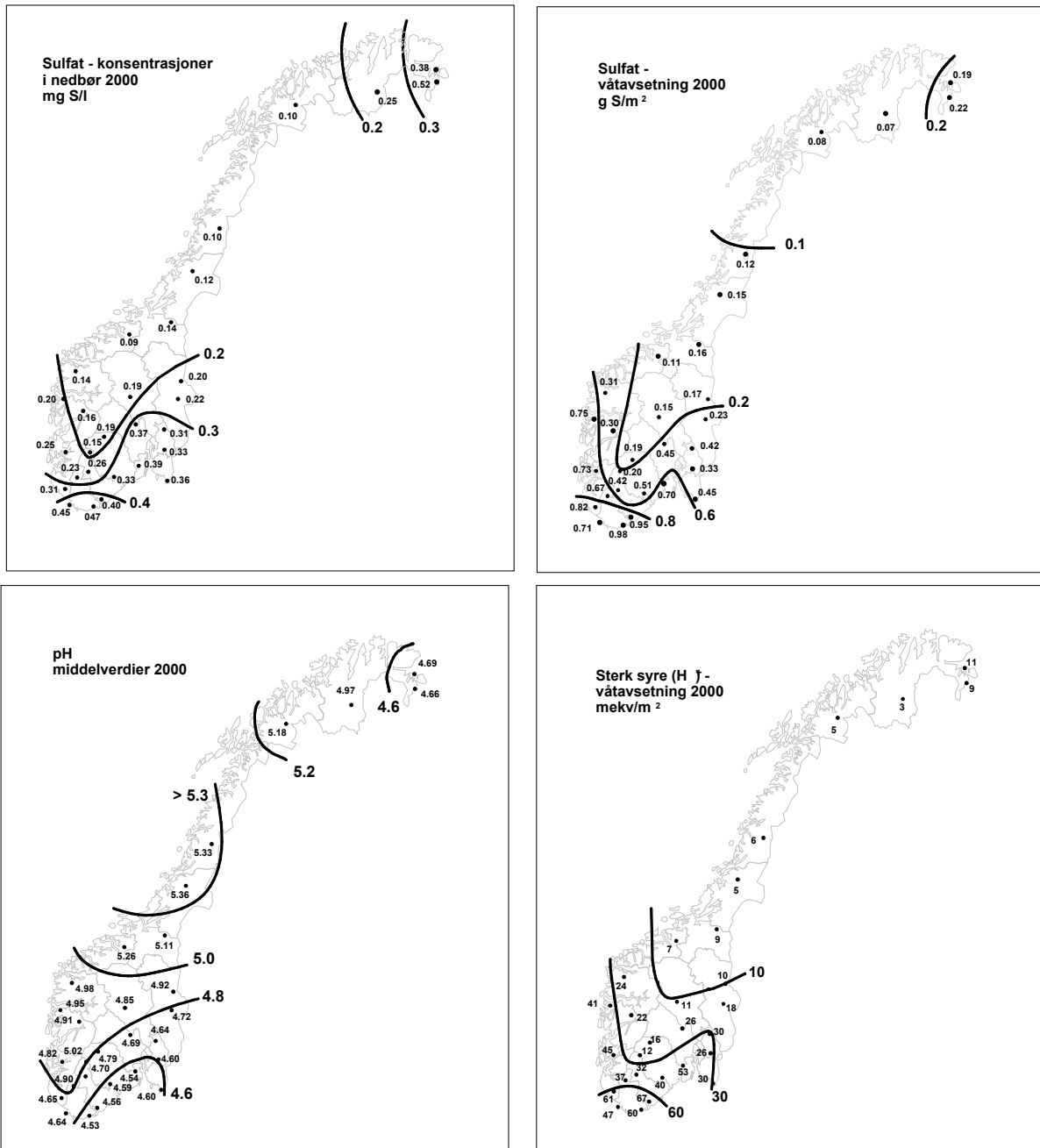
Figur 1.1: Middelskonsentrasjoner i nedbør og våtavsetning av sulfat (sjøsaltkorrigert) og sterk syre (pH) på norske bakgrunnsstasjoner i 2000.
